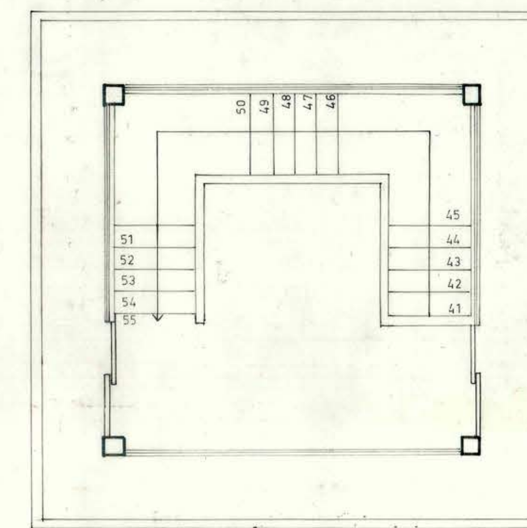
PLANTA 4º PISO MIRADOR
