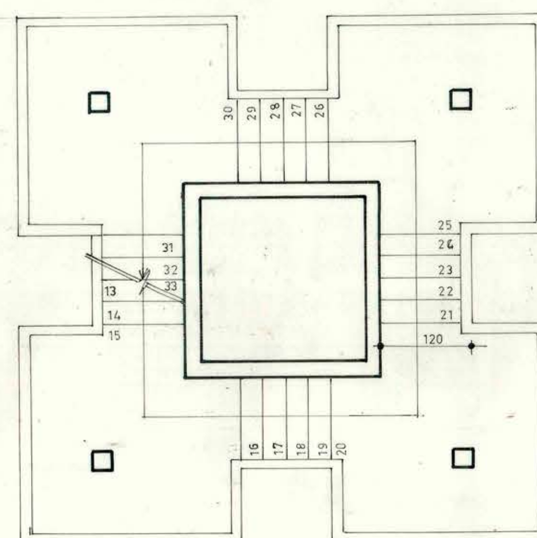
PLANTA 2º PISO
