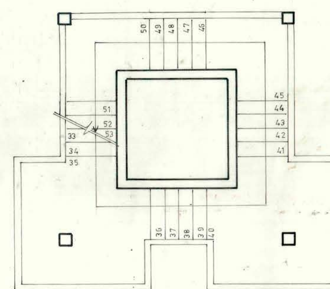
PLANTA 3er PISO
