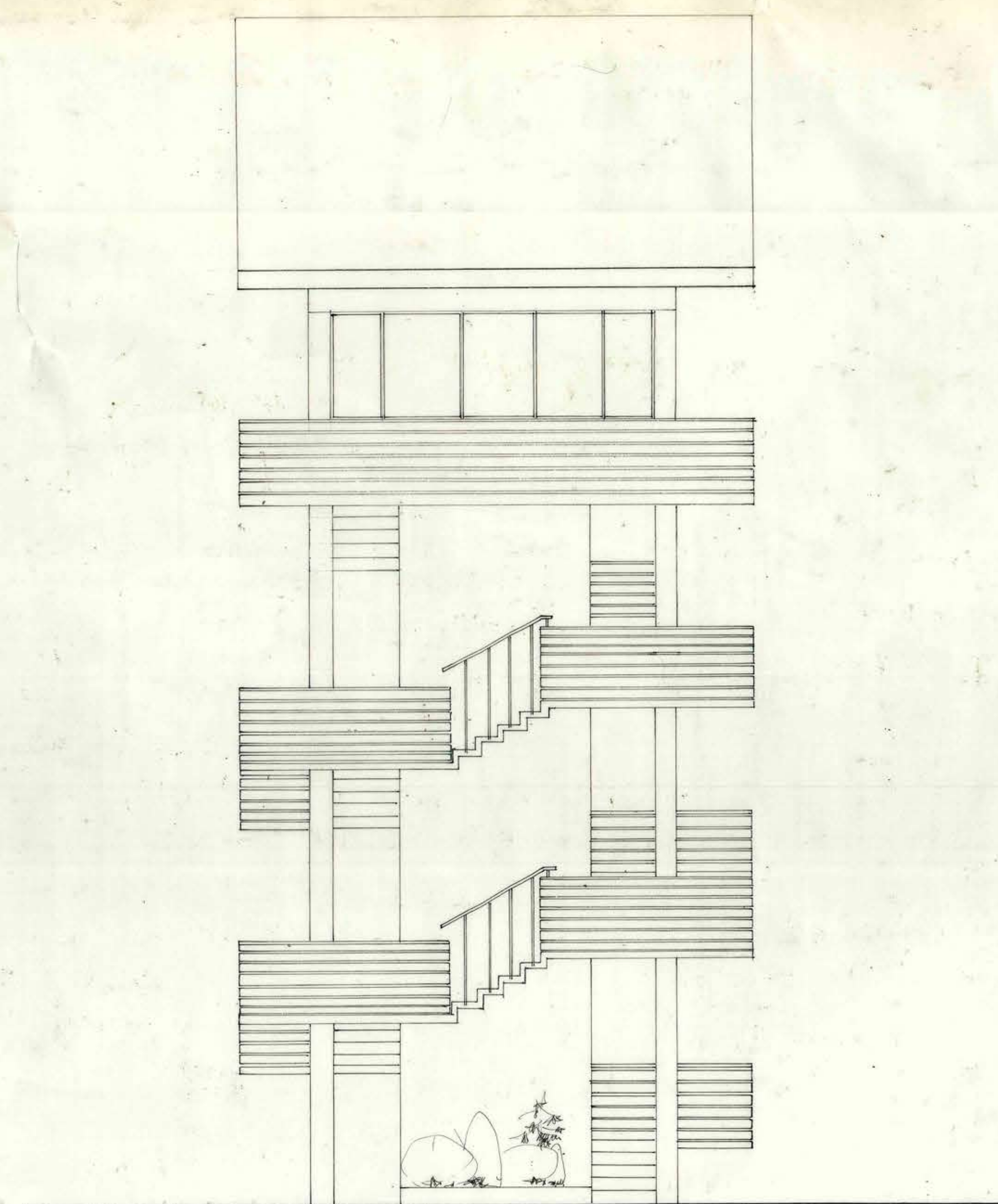
ELEVACION SUR
