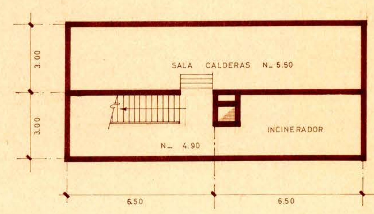
TESORERIA PROVINCIAL NIVEL - 4.90
