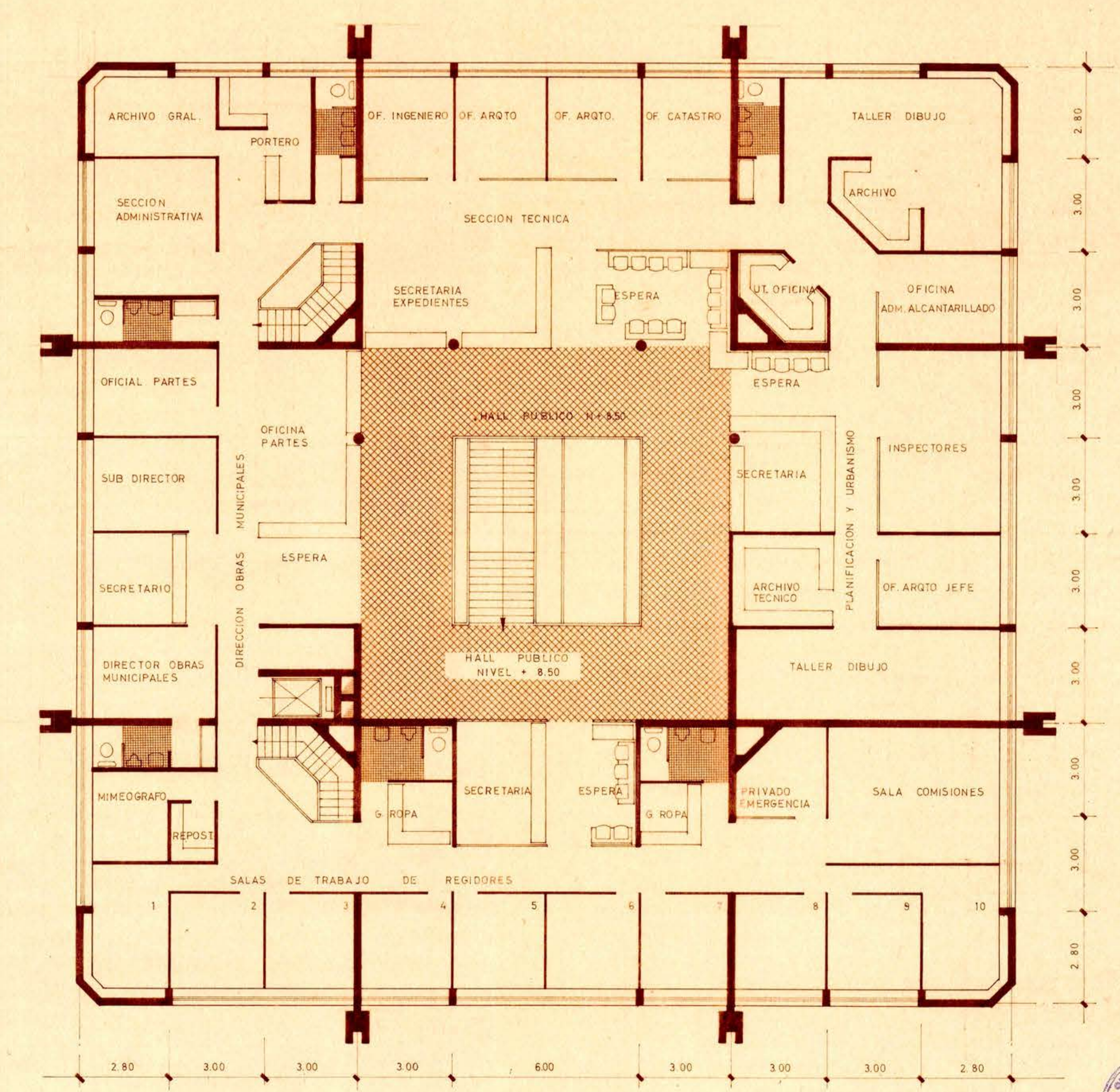
EDIFICIO CONSISTORIAL NIVEL + 8.50
