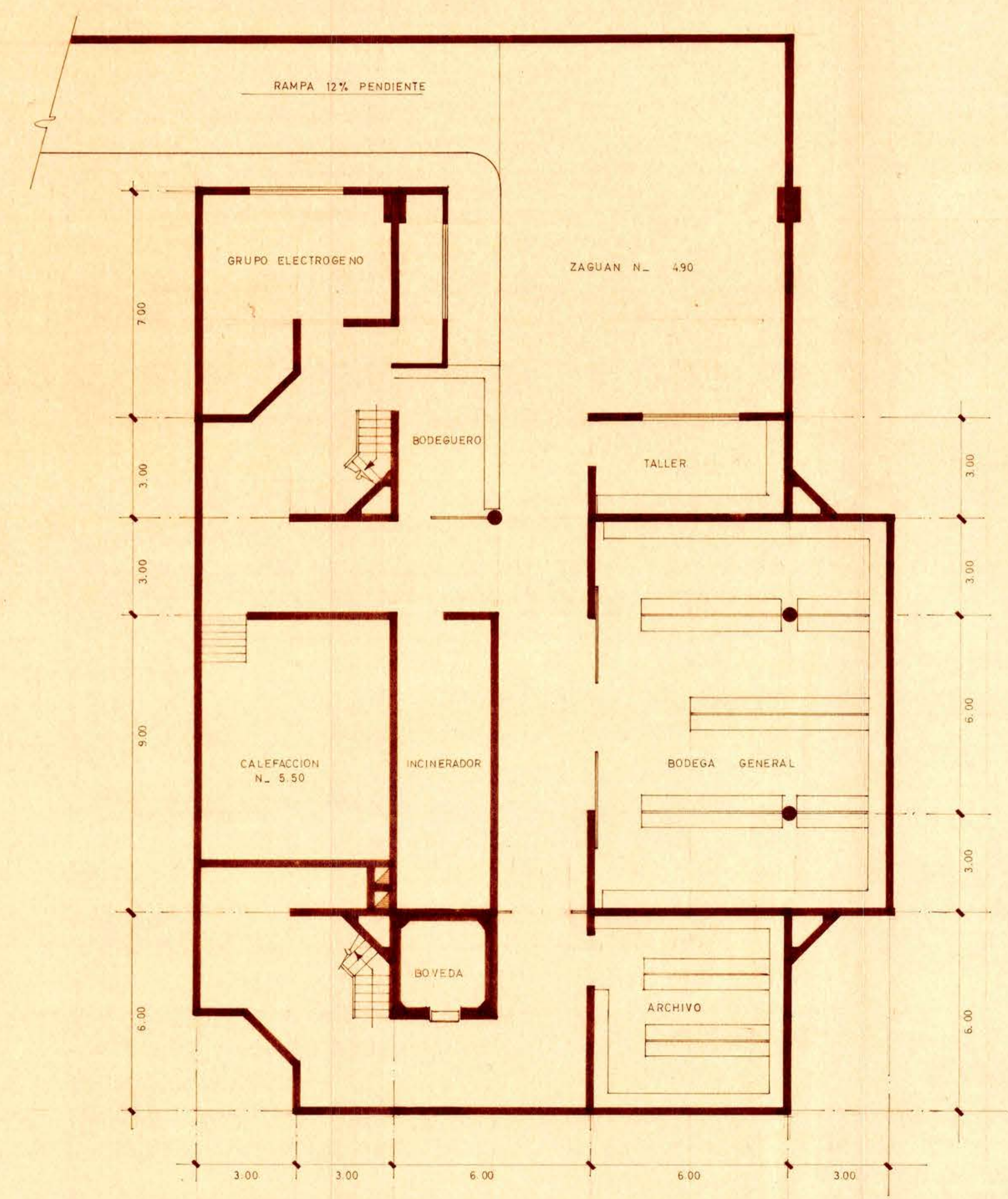
EDIFICIO CONSISTORIAL NIVEL - 4.90
