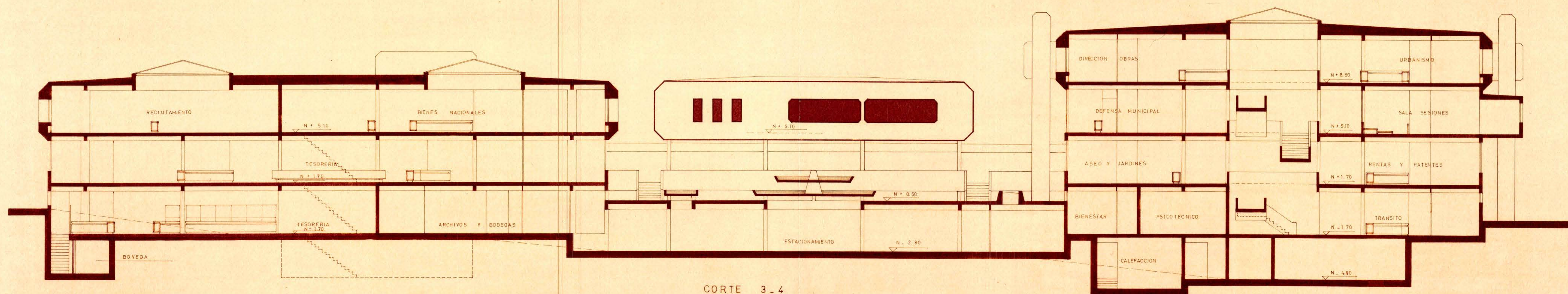
CORTE 3-4
