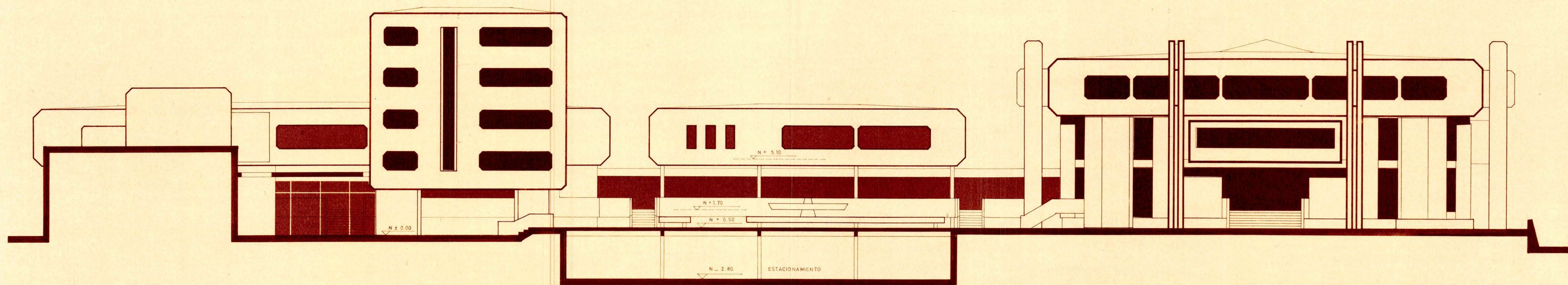
CORTE 1-2 FACHADA ORIENTE
