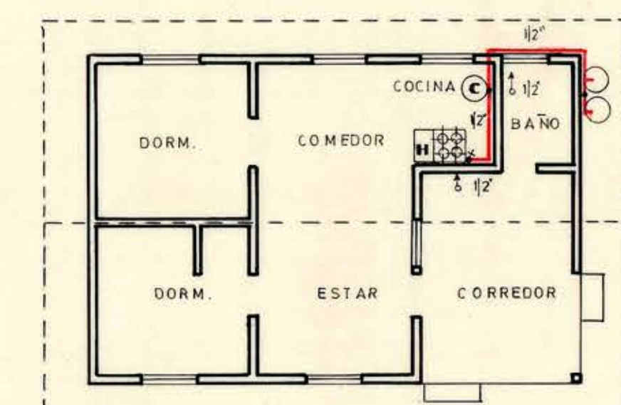
VIVIENDA VISITAS
