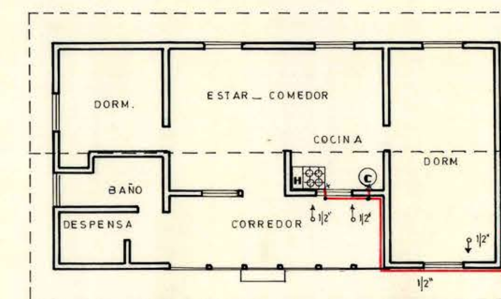
VIVIENDA FUNCIONARIOS
