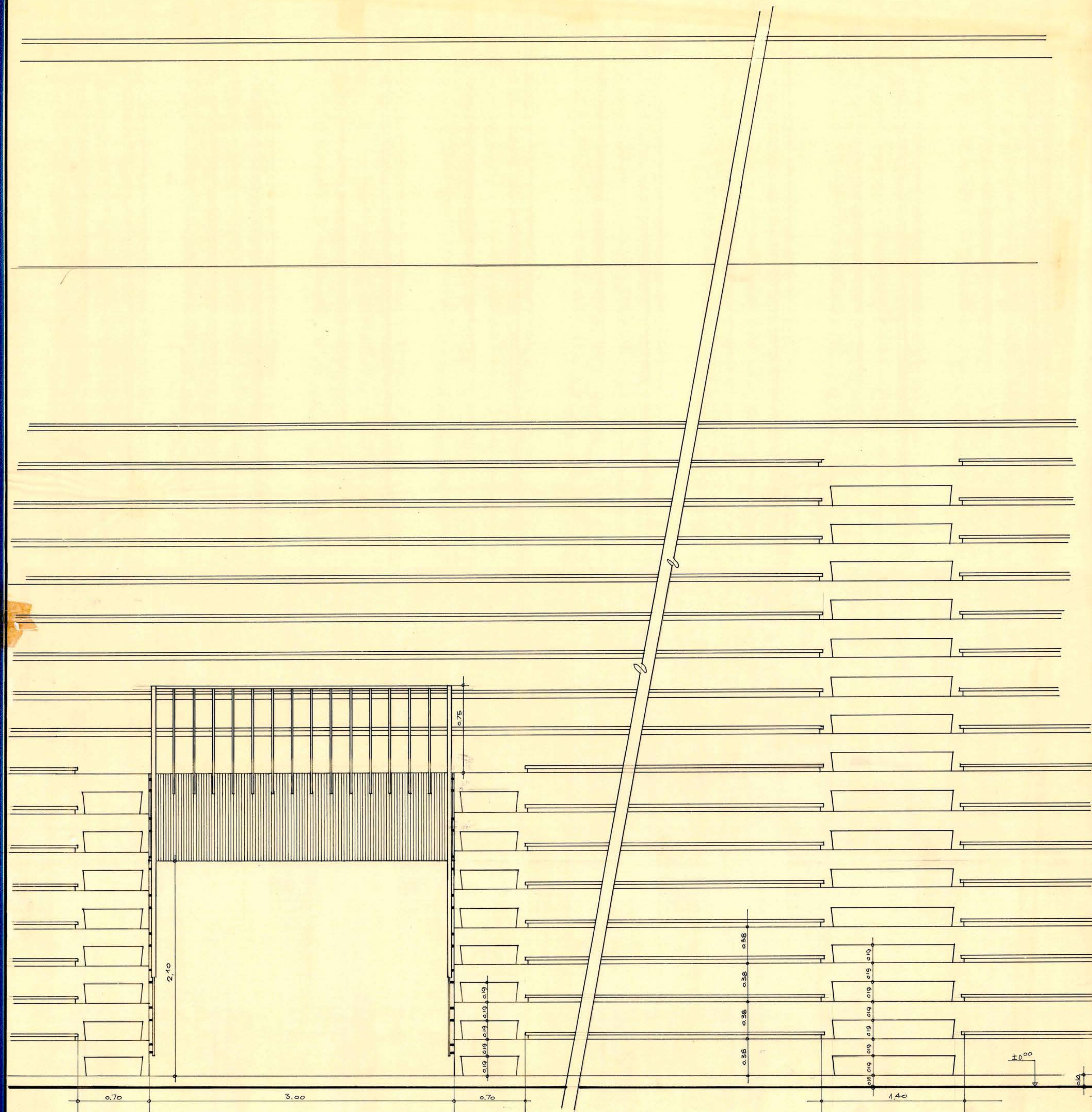
• FACHADA GRADERIAS • 1:20
