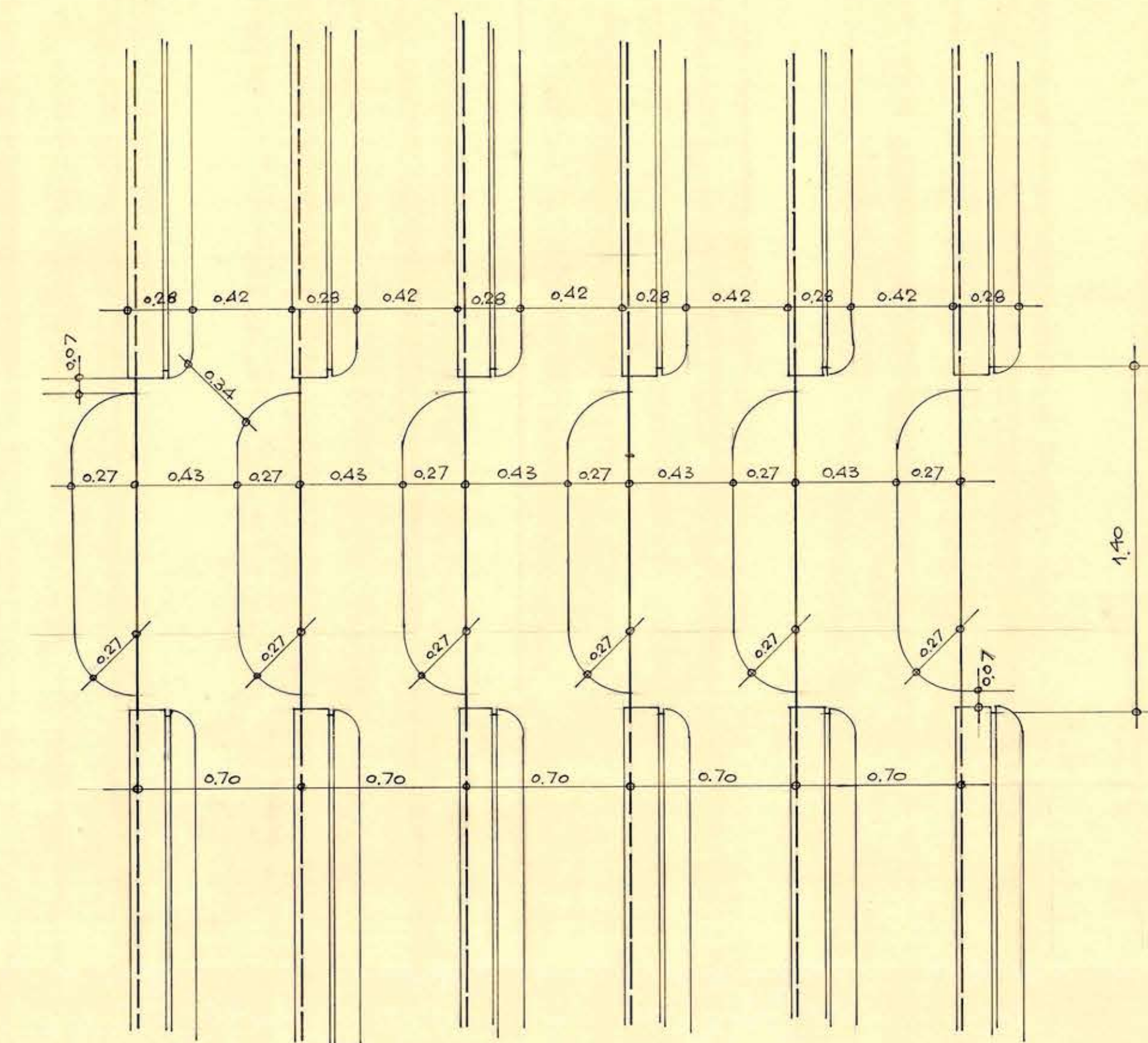
• DETALLE PELDAÑOS • 1:20
