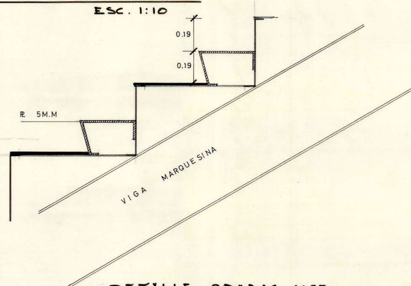
DETALLE GRADAS MET ESC. 1:10
