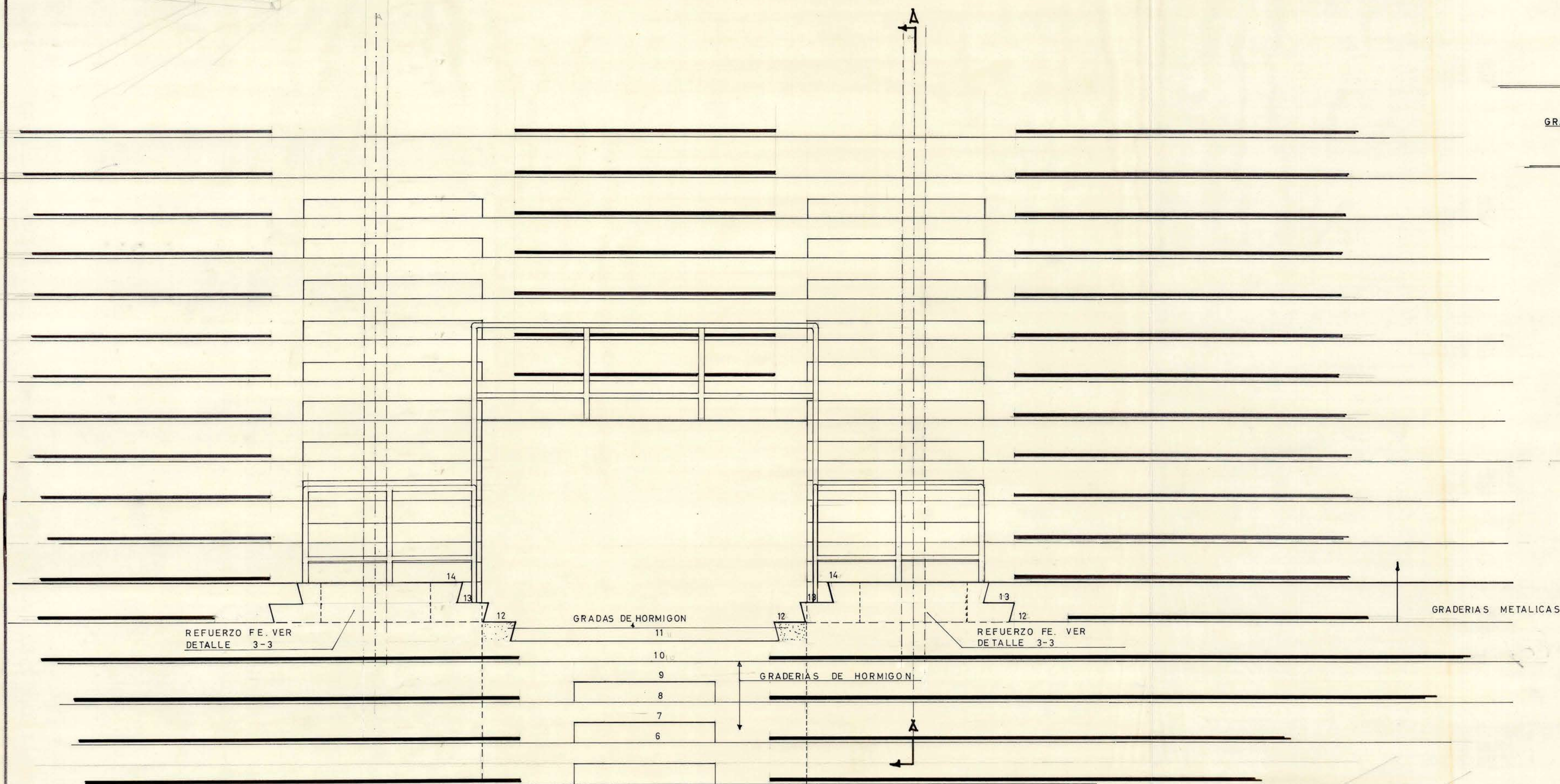
VISTA BOCA GRADERIAS DESDE LA CANCHA FUTBAL ESC. 1:20
