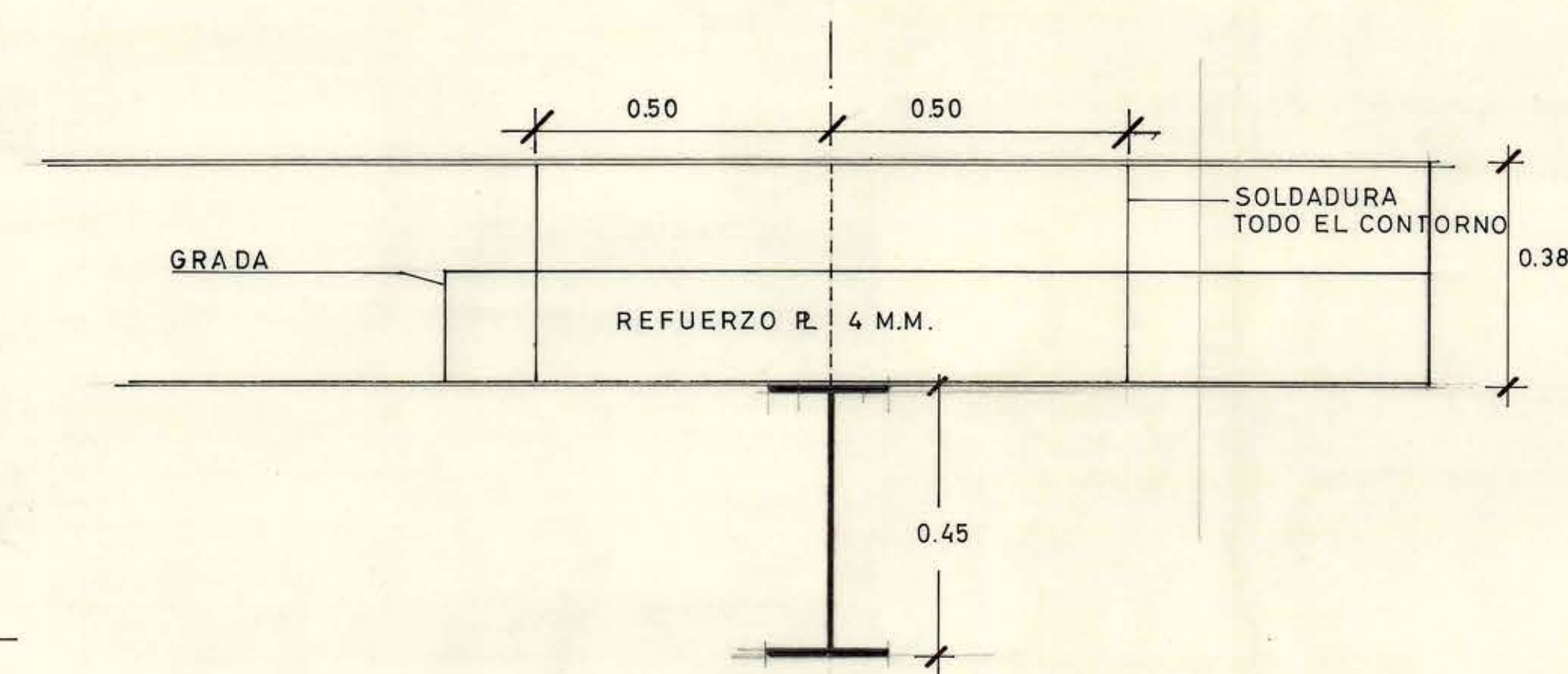
DETALLE 3-3 ESC. 1:10
