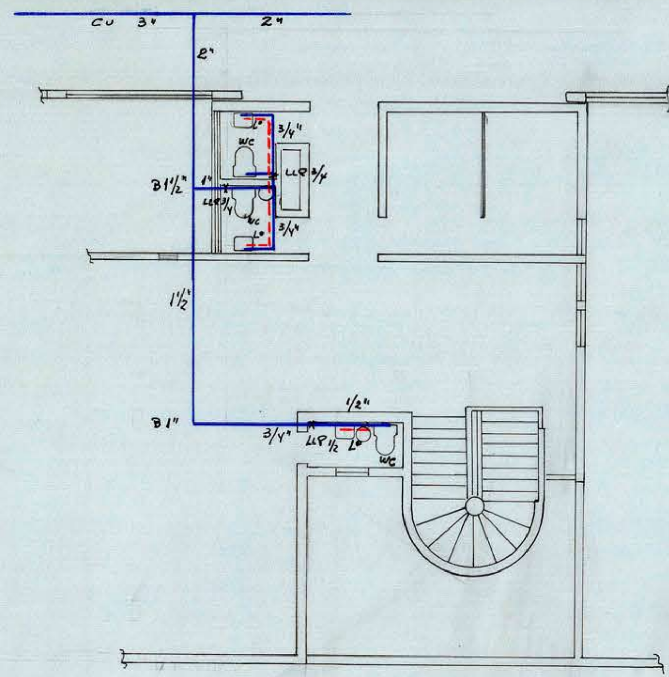
PLANTA 2º PISO
