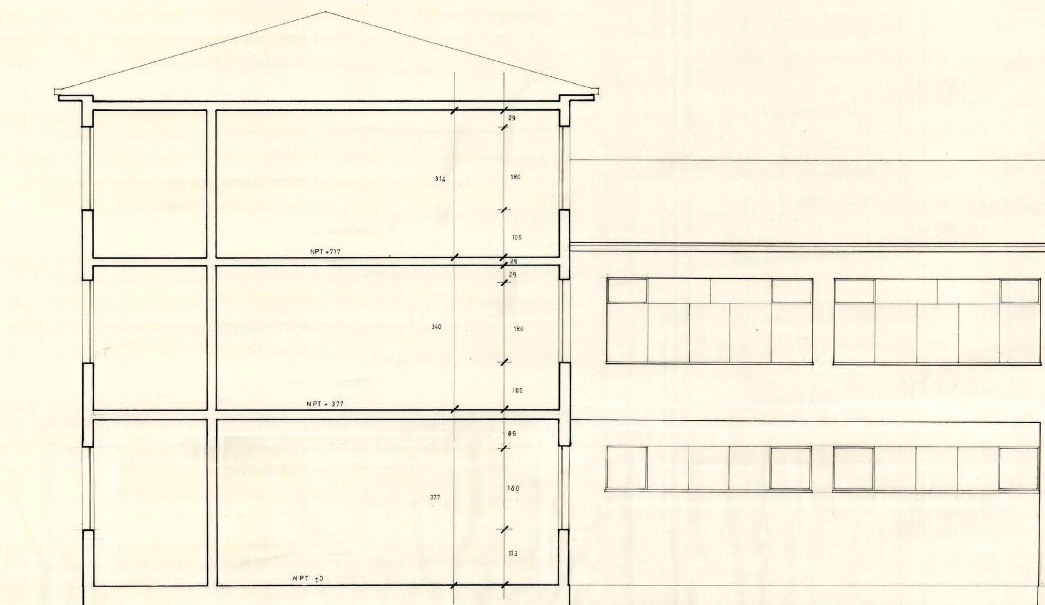
CORTE A-A.
