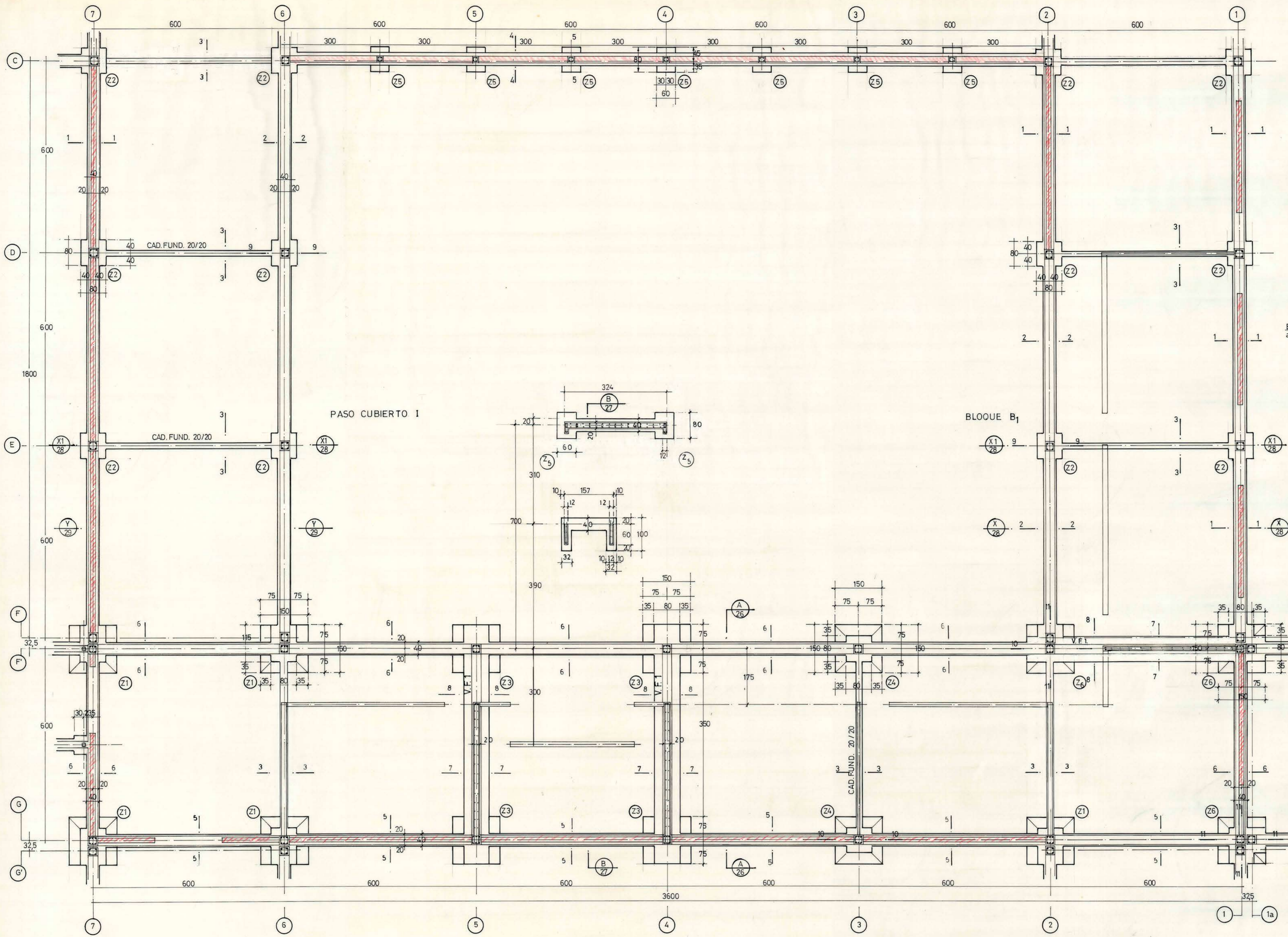
PLANTA FUNDACIONES BLOQUE B ESCALA 1:50
