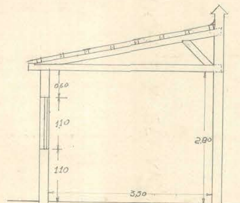
Corte A-A
