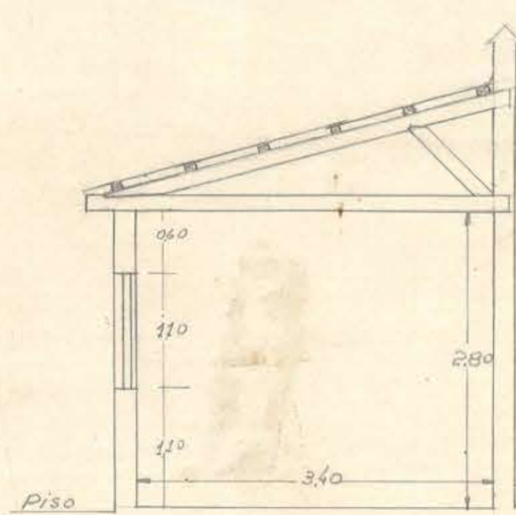
Corte A-A.
