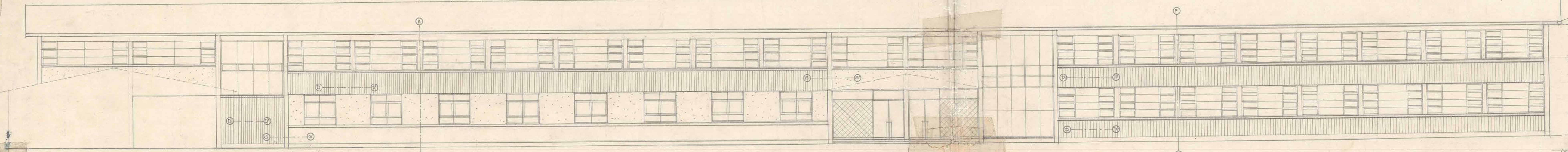
FACHADA NOR-PONIENTE.
