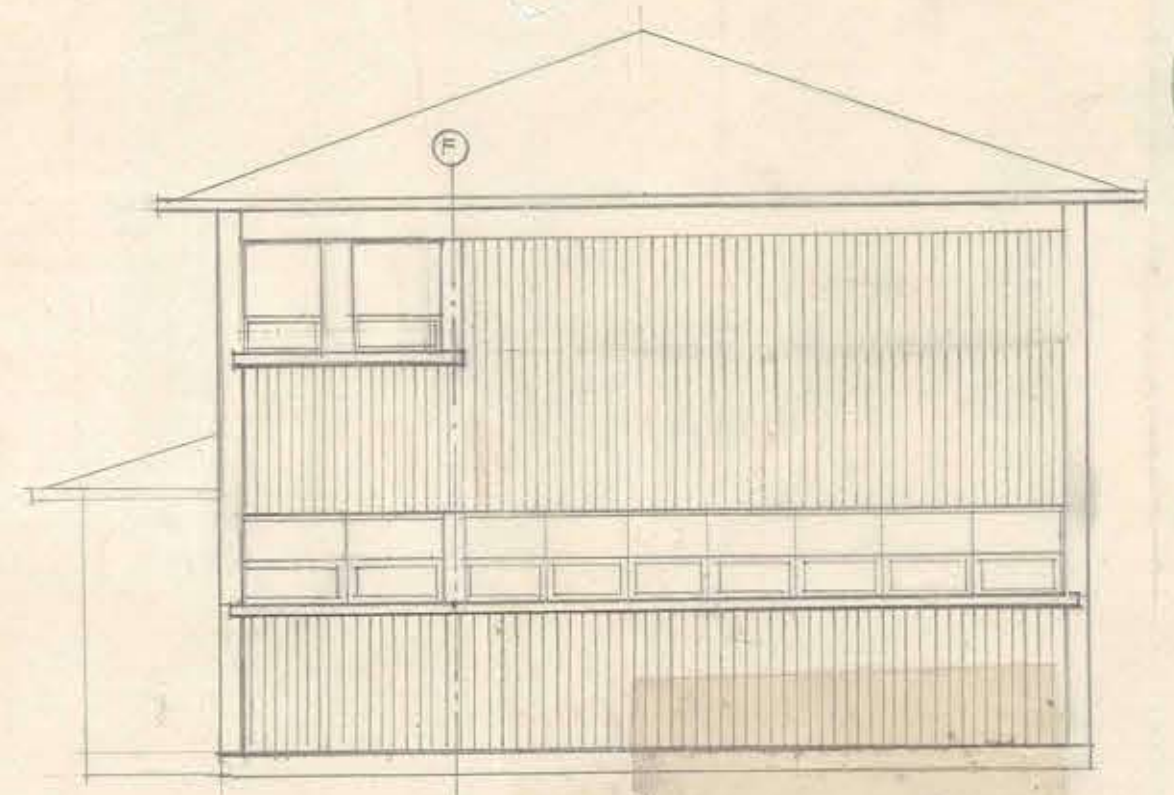
FACHADA ORIENTE C. CALAMA.
