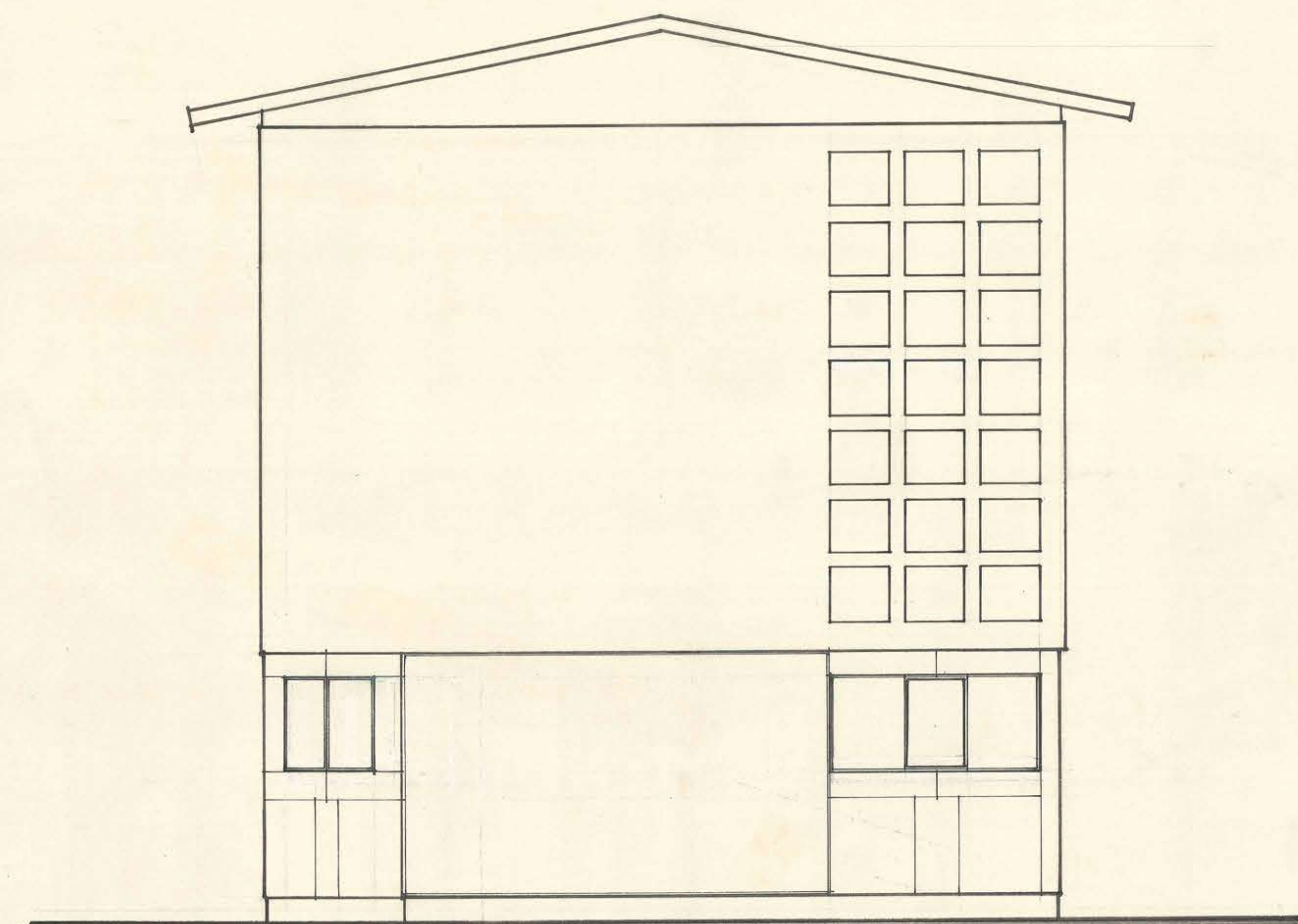
FACHADA NORTE ES. 1:50.-
