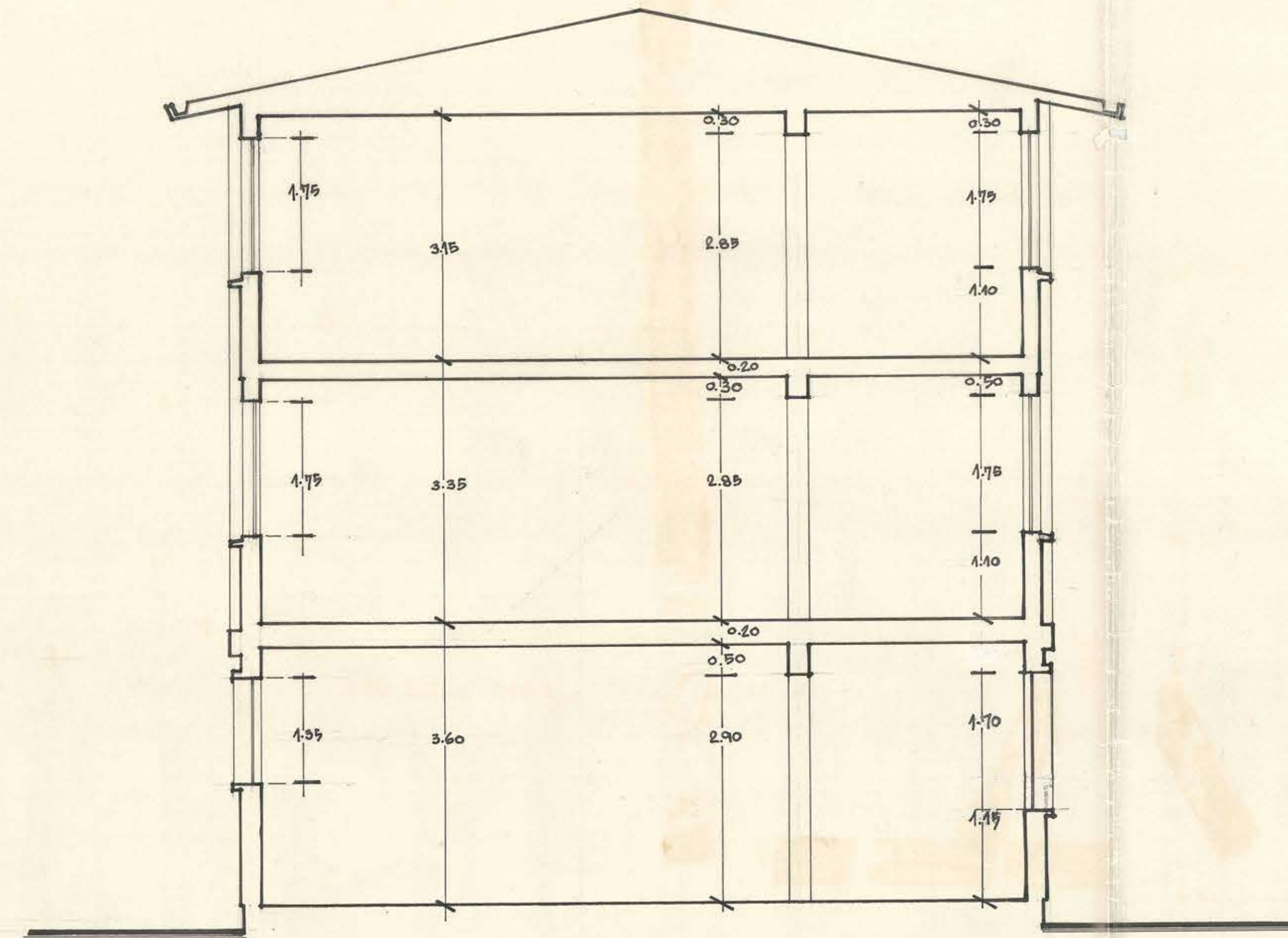
CORTE TRANSVERSAL X-X
