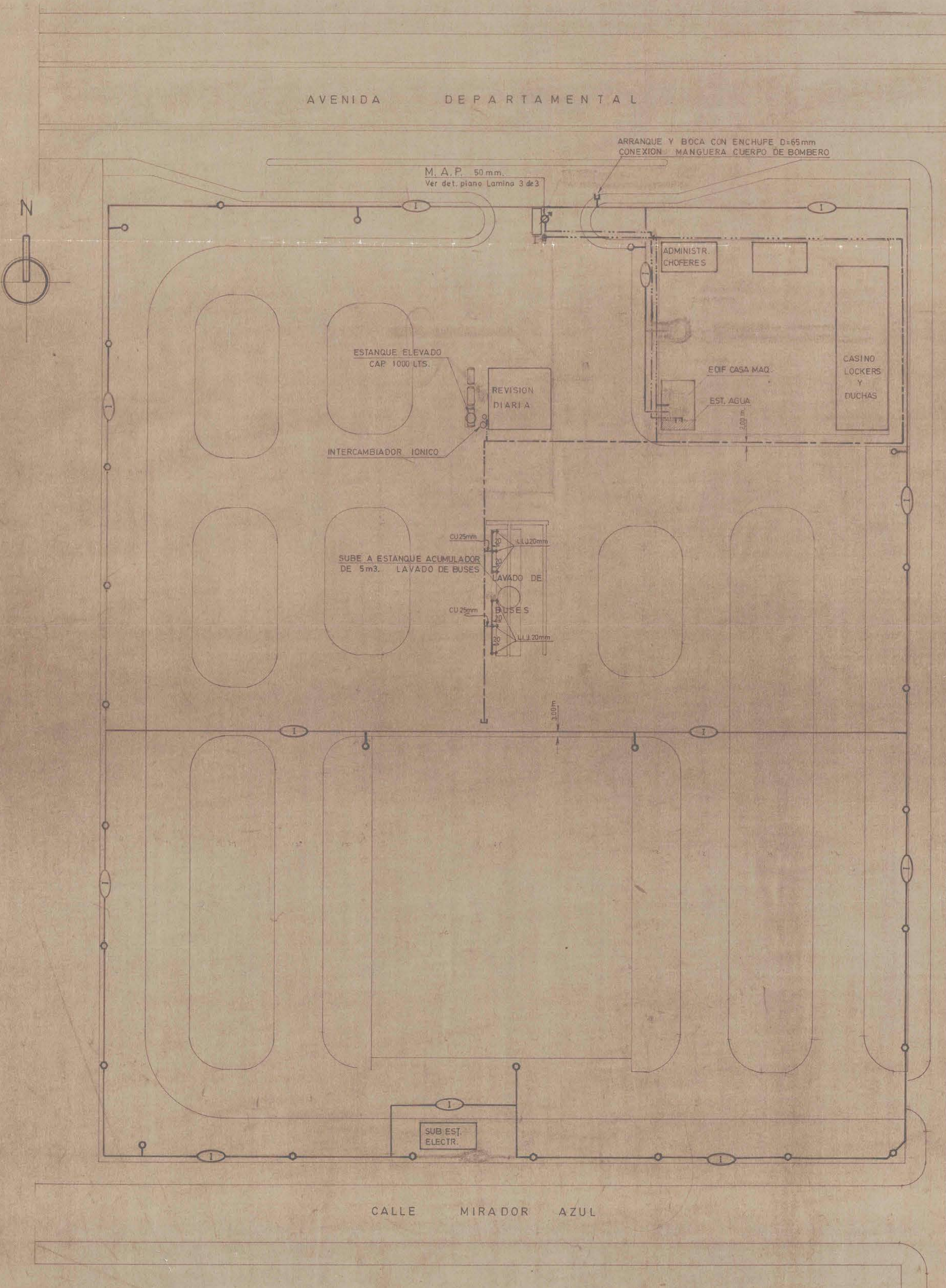
PLANTA GENERAL ESCALA 1:500
