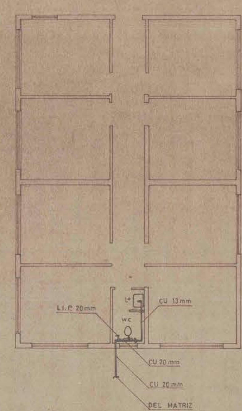
OFICINA ADMINISTRACION ESCALA 1:100
