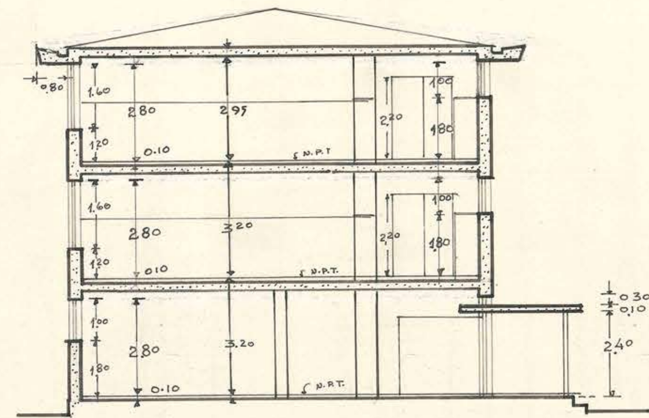
SECCION A-B
