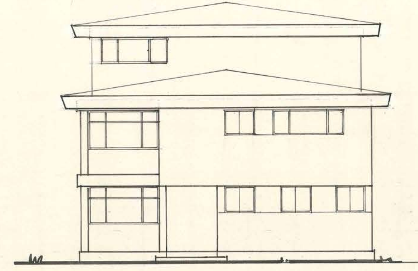
FACHADA ORIENTE
