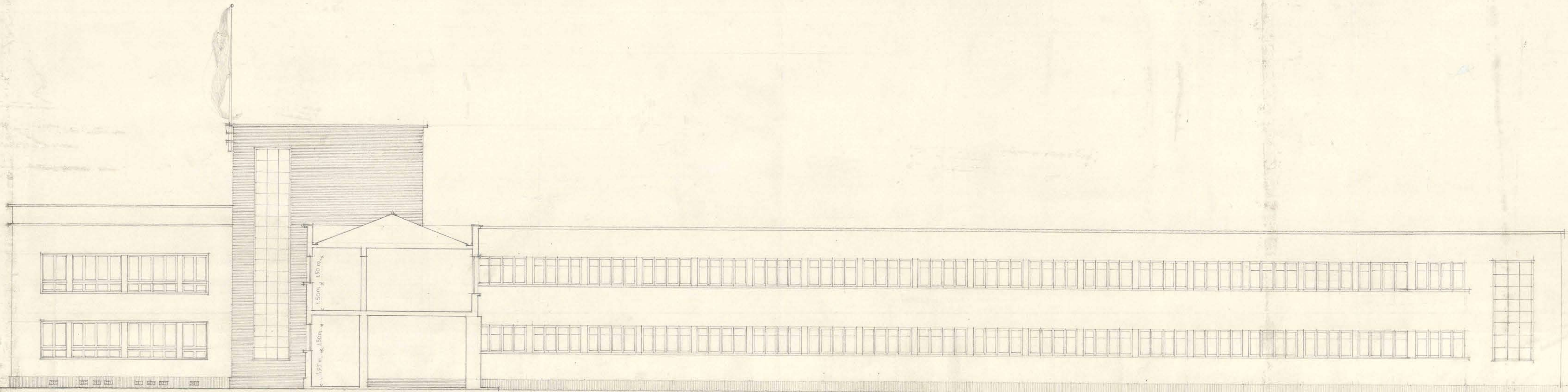
FACHADA SUR Y SECCION PATIO CUBIERTO.
