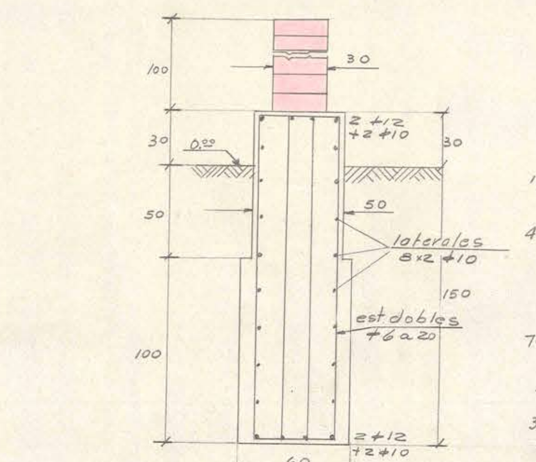
CORTE B-B
