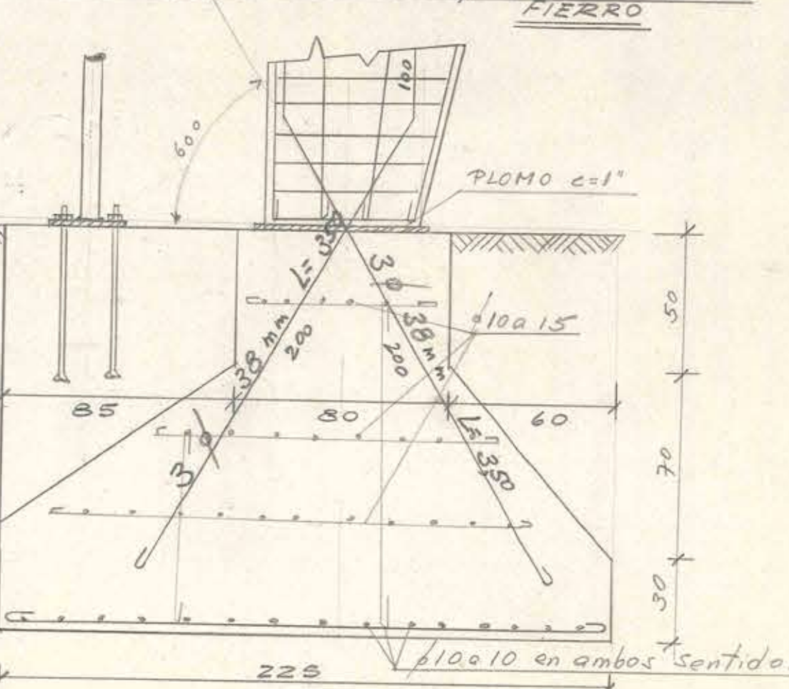
FUNDACION MACCHON (4) Y PRIMER PILAR FIERRO
