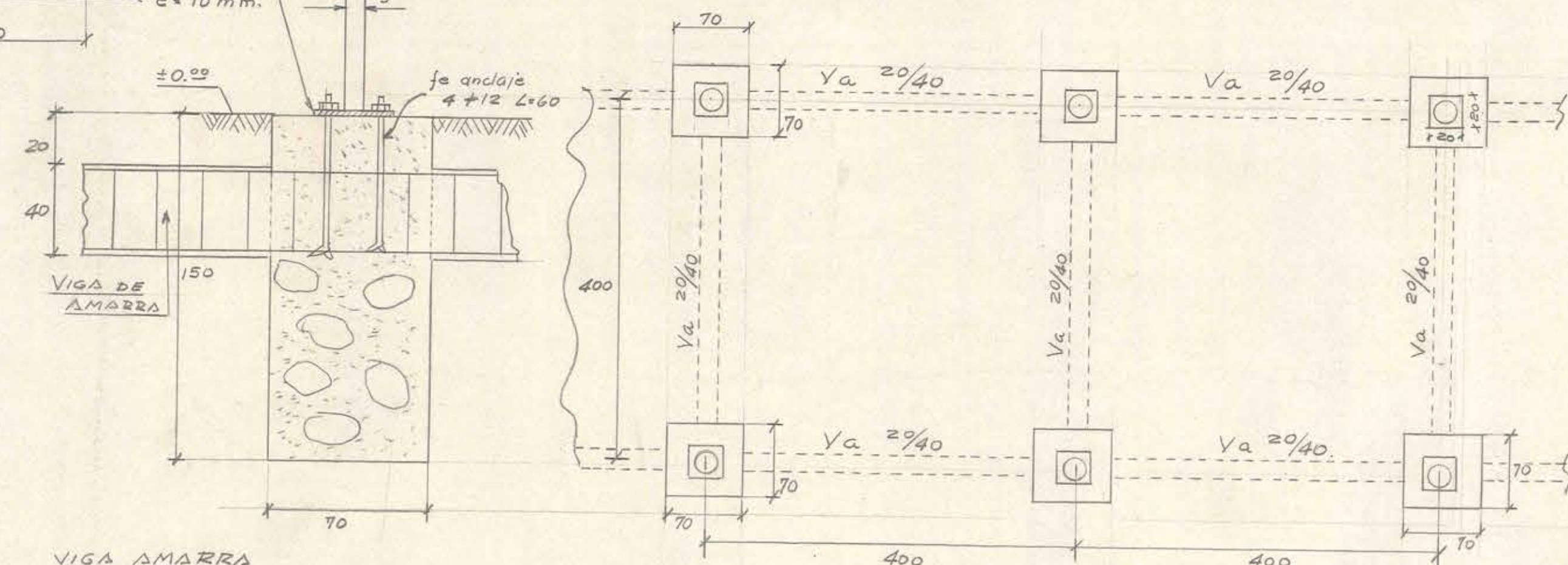
PLANTA FUNDACIONES PILARES FIERRO CORREDOR
