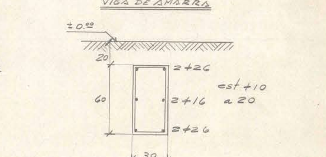
CORTE F-F
