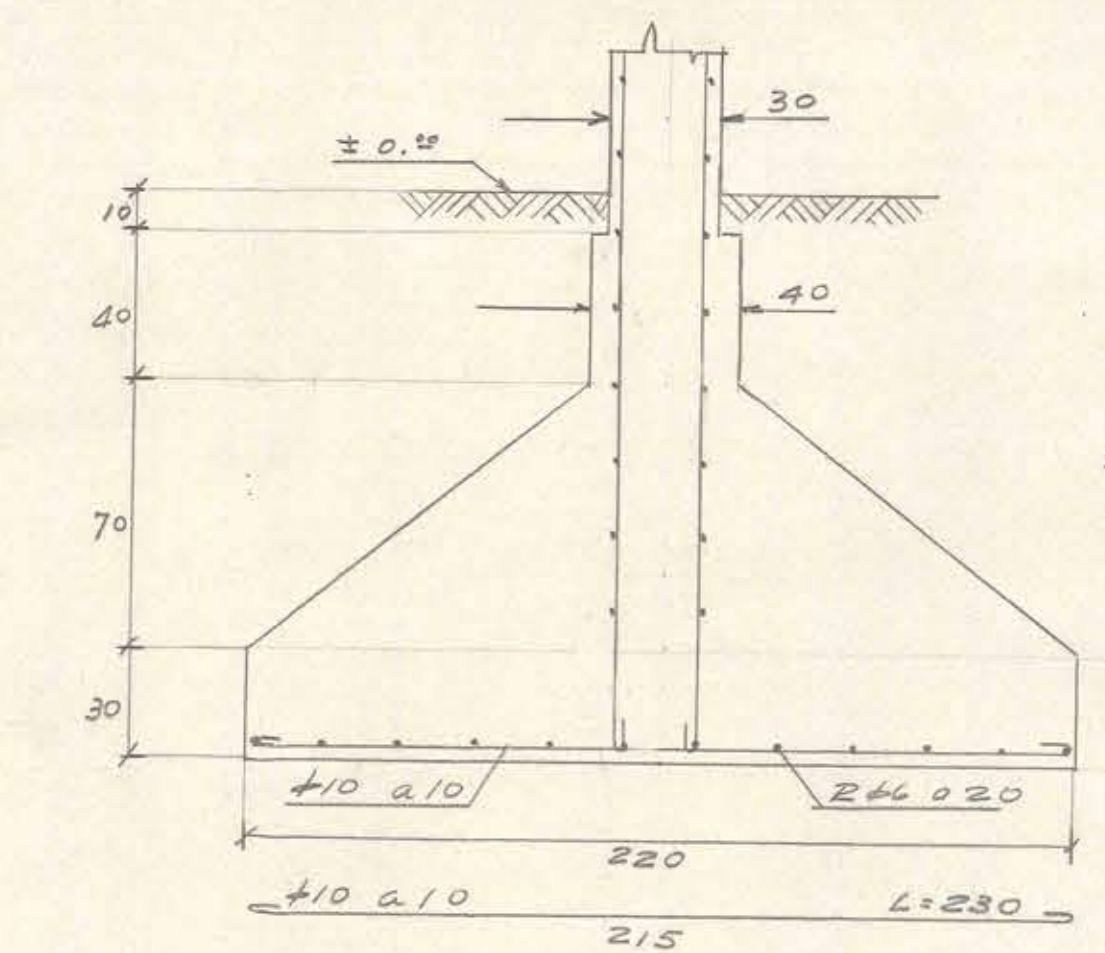
CORTE A-A
