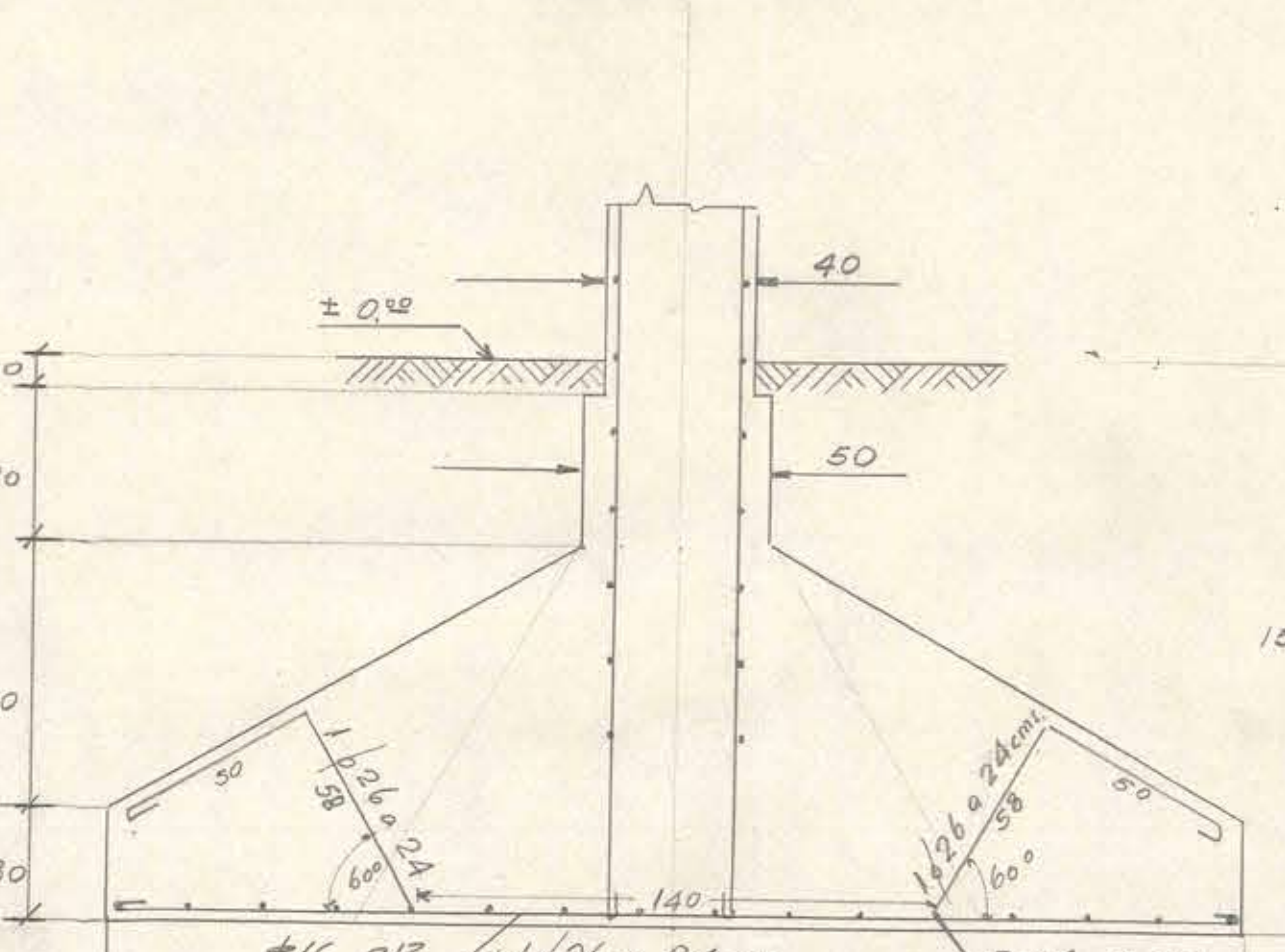
CORTE C-C
