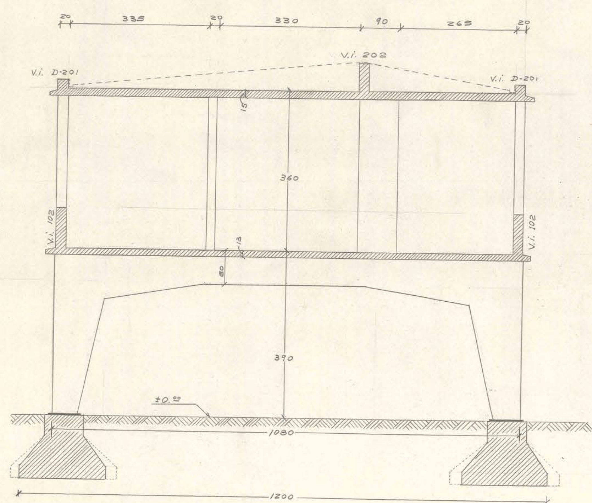
CORTE I-I
