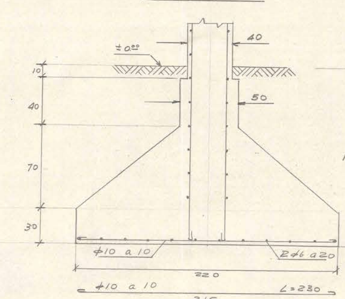
CORTE A1-A1
