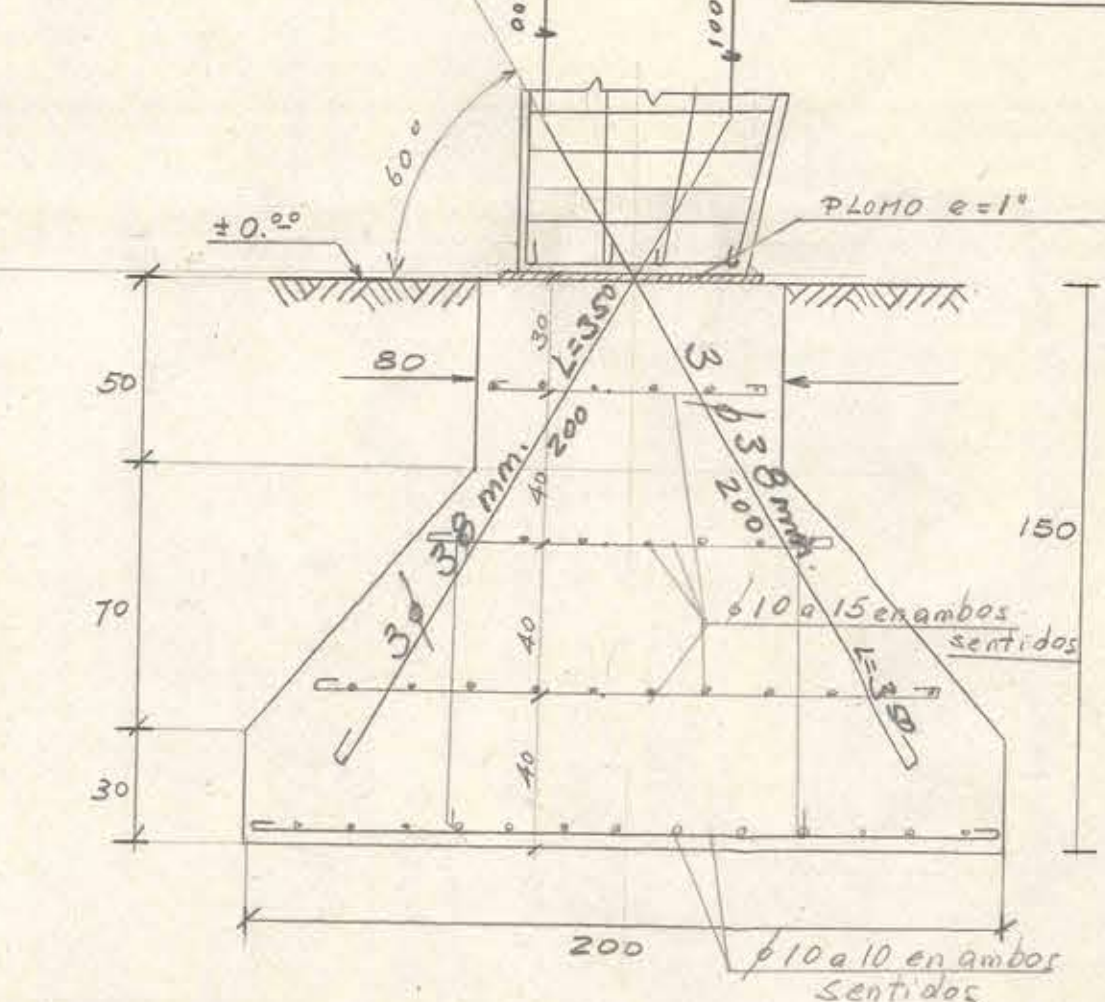
FUNDACION MARCOS (2)
