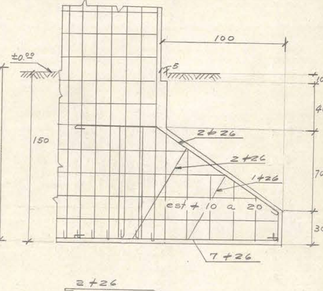
VOLADO FUND. A, A1, C
