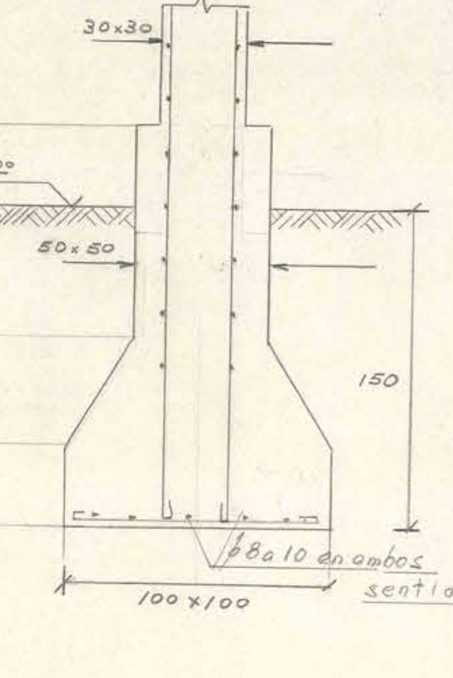
FUNDACION PILAR (5)
