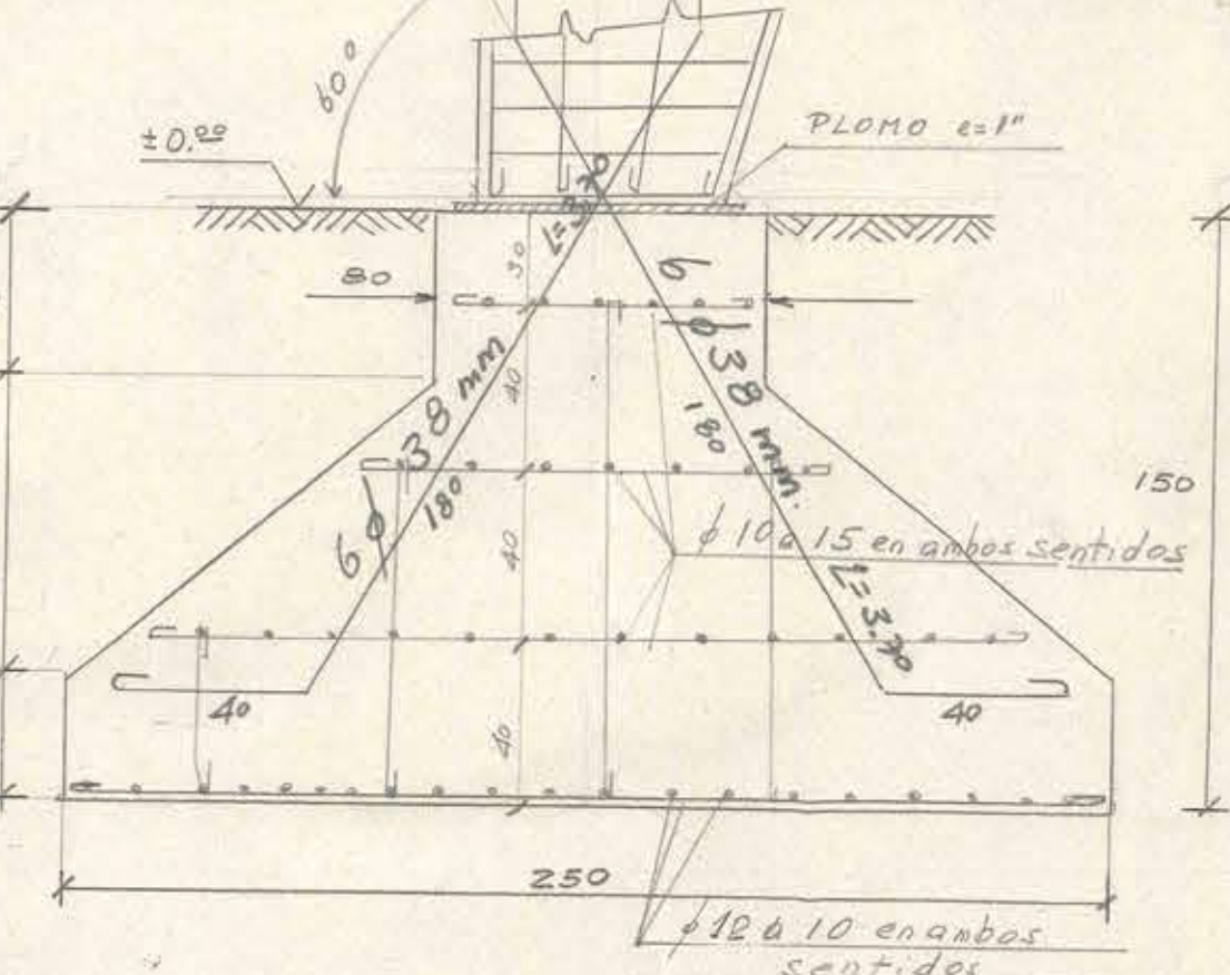
FUNDACION MACCHON (4) Y PRIMER PILAR FIERRO
