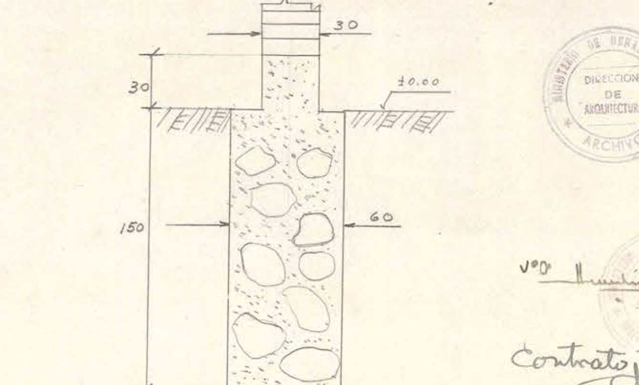
CORTE E-E
