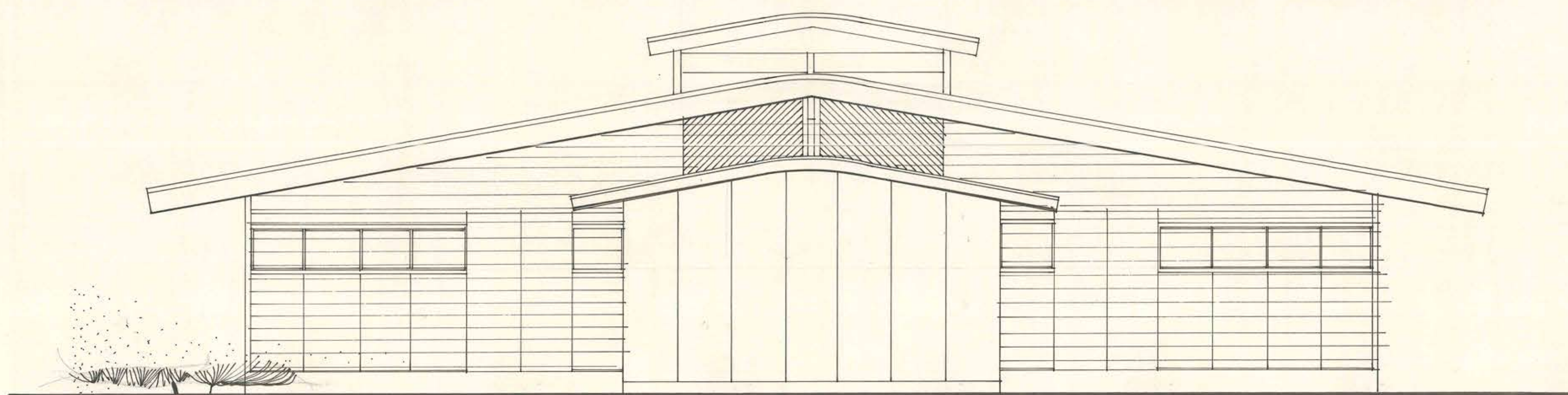
ELEVACION POSTERIOR
