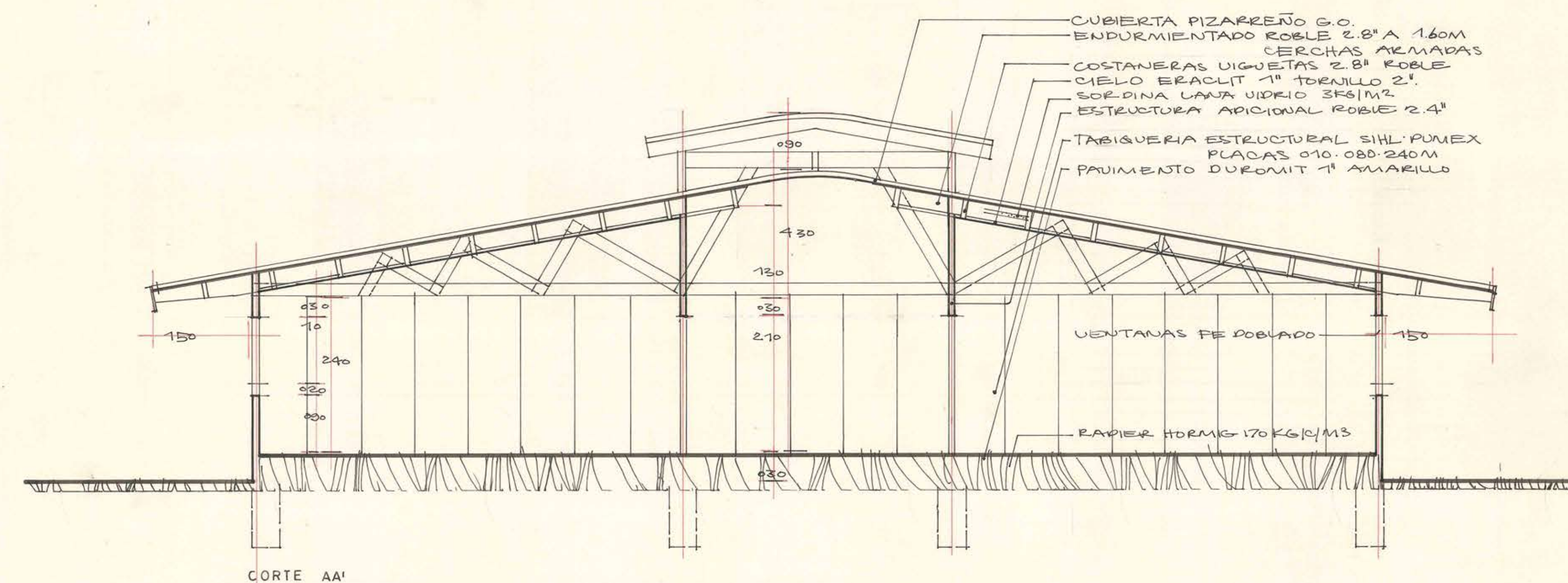
CORTE AA'
