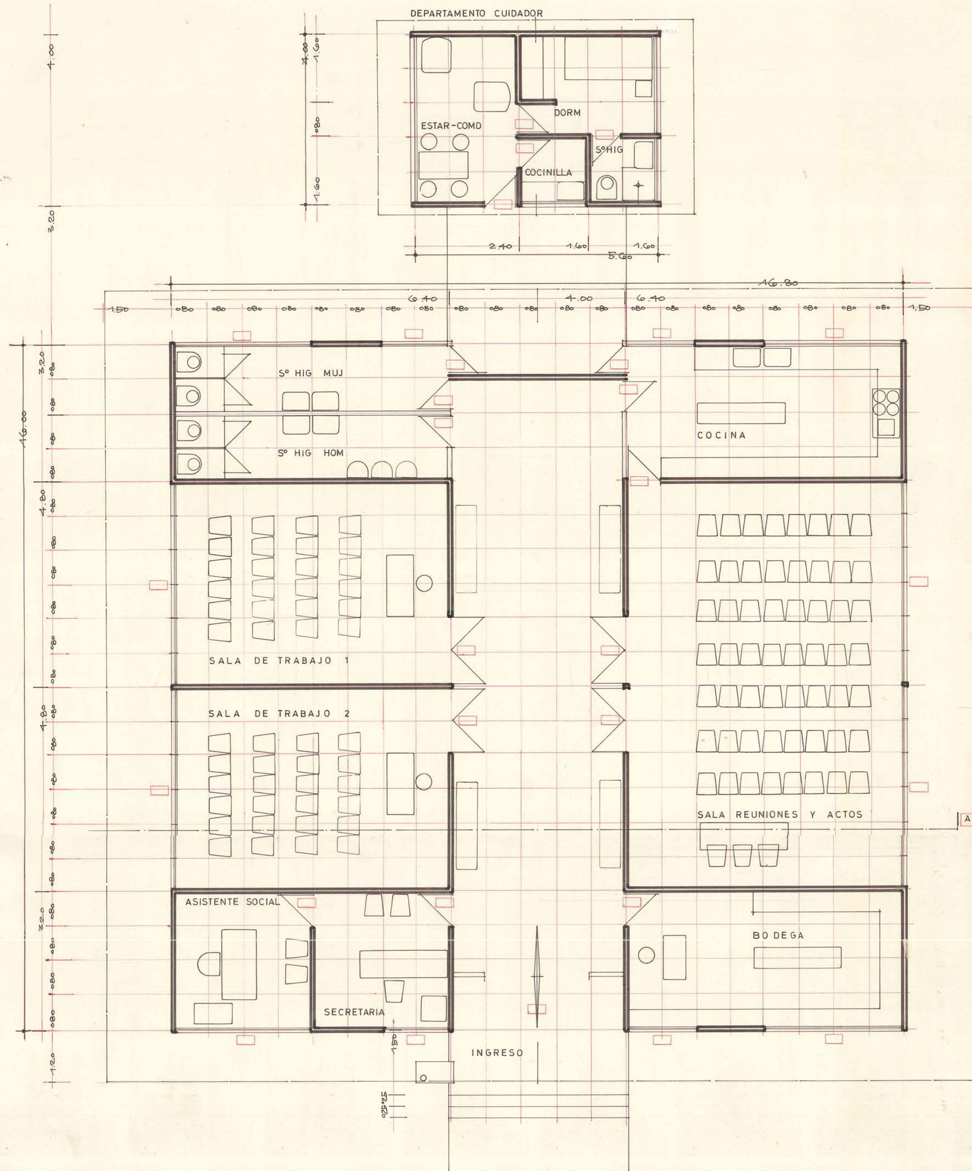
PLANTA GENERAL
