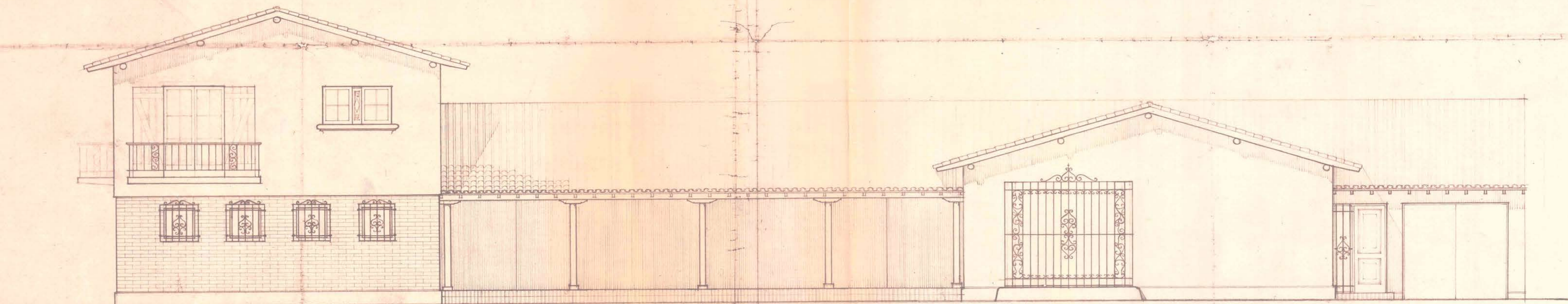
FACHADA PONIENTE
