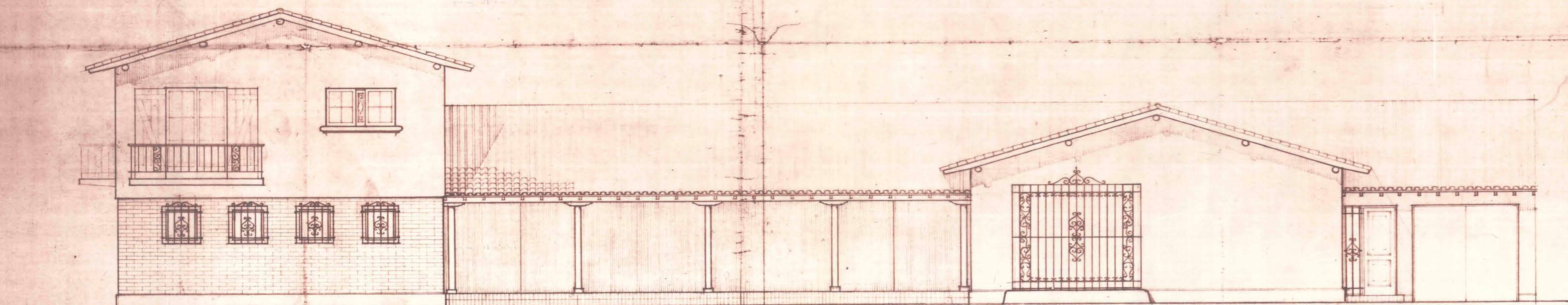
— FACHADA PONIENTE —
