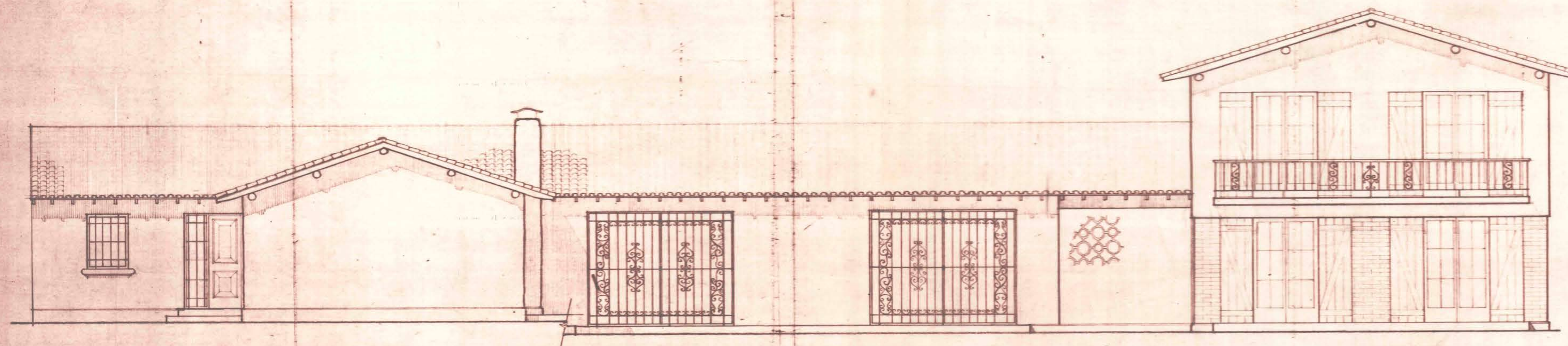
— FACHADA ORIENTE —
