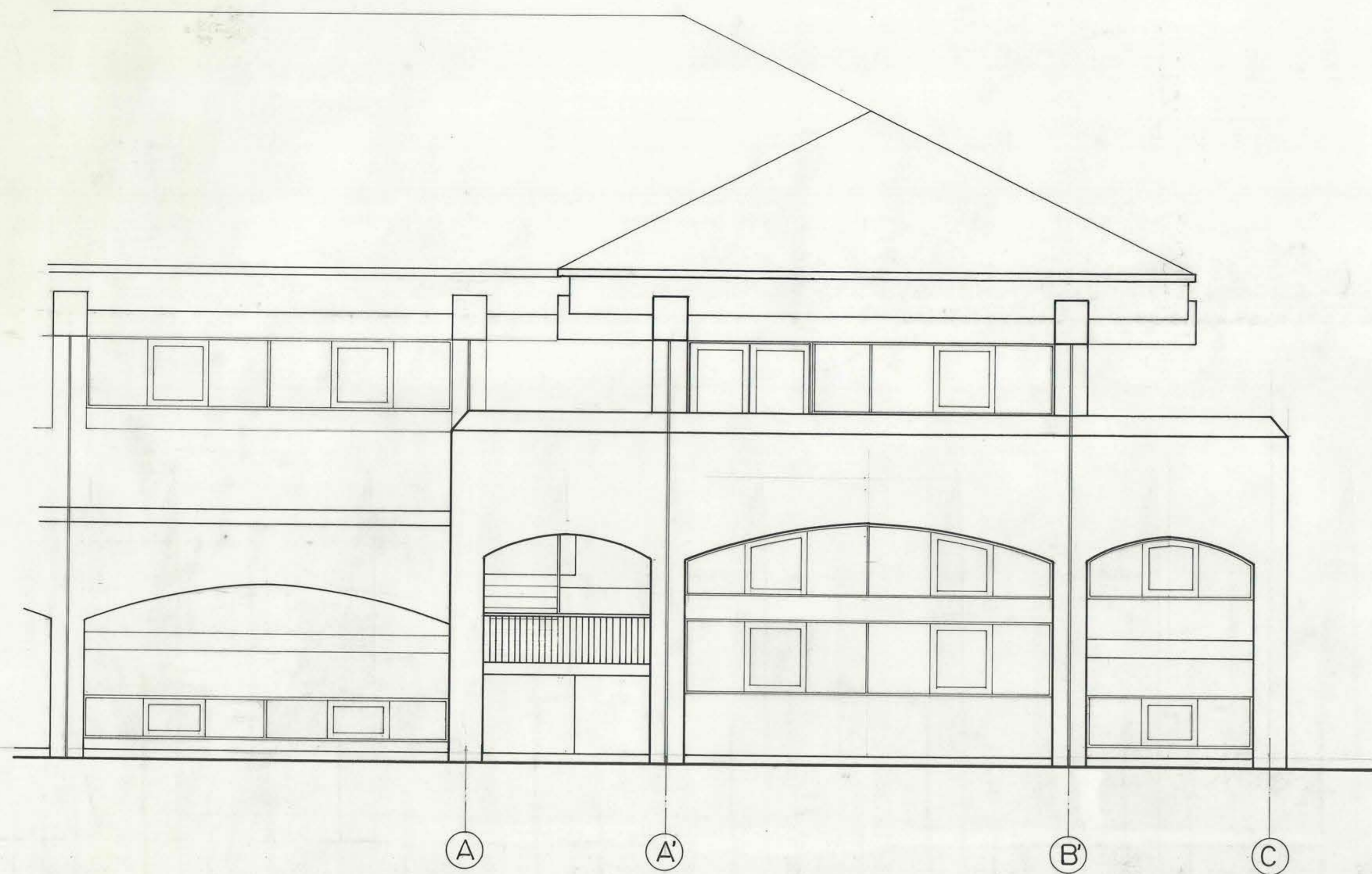
ELEVACION SUR CUERPO D esc 1 : 50
