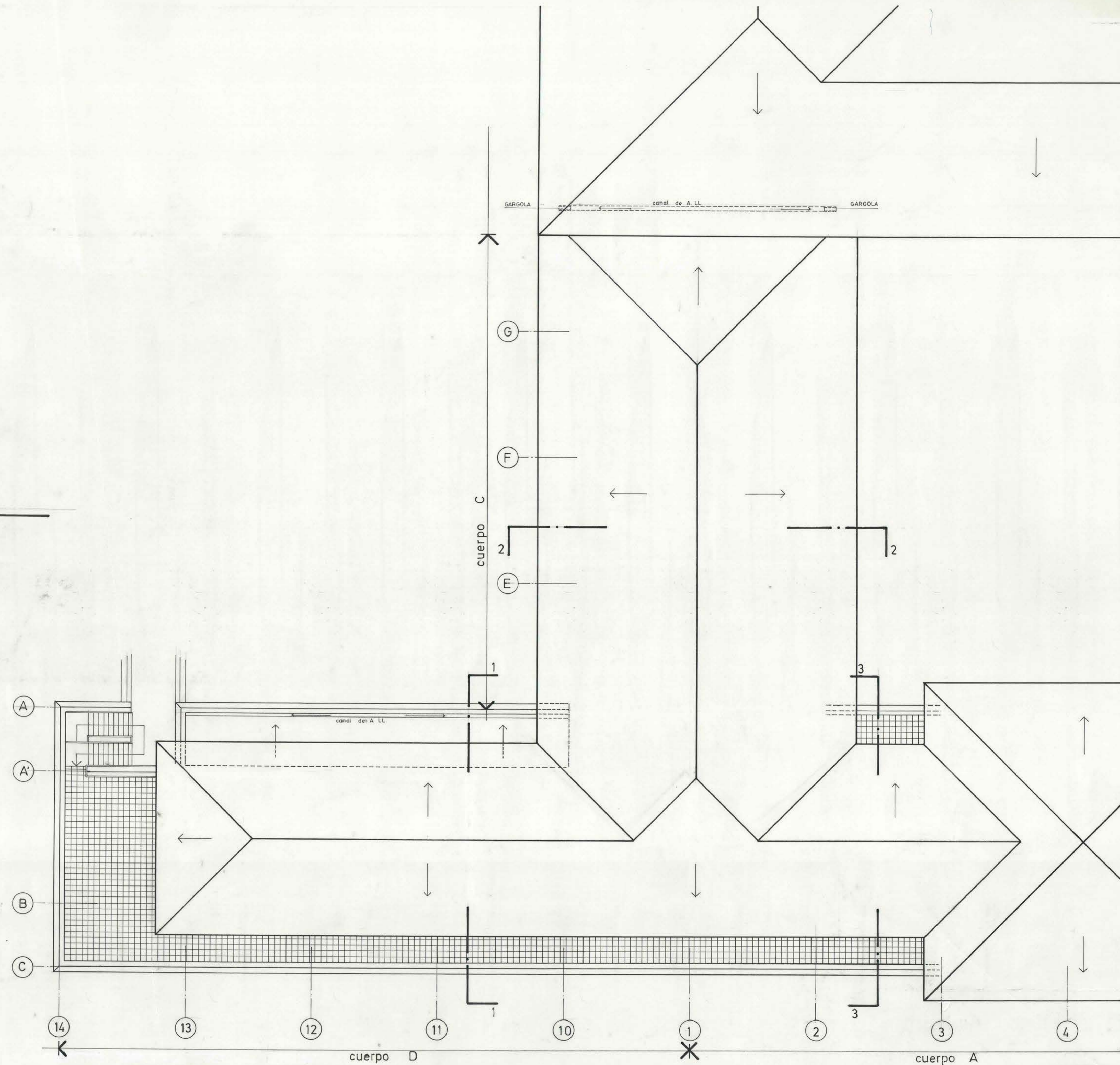
PLANTA DE CUBIERTA esc 1 : 100
