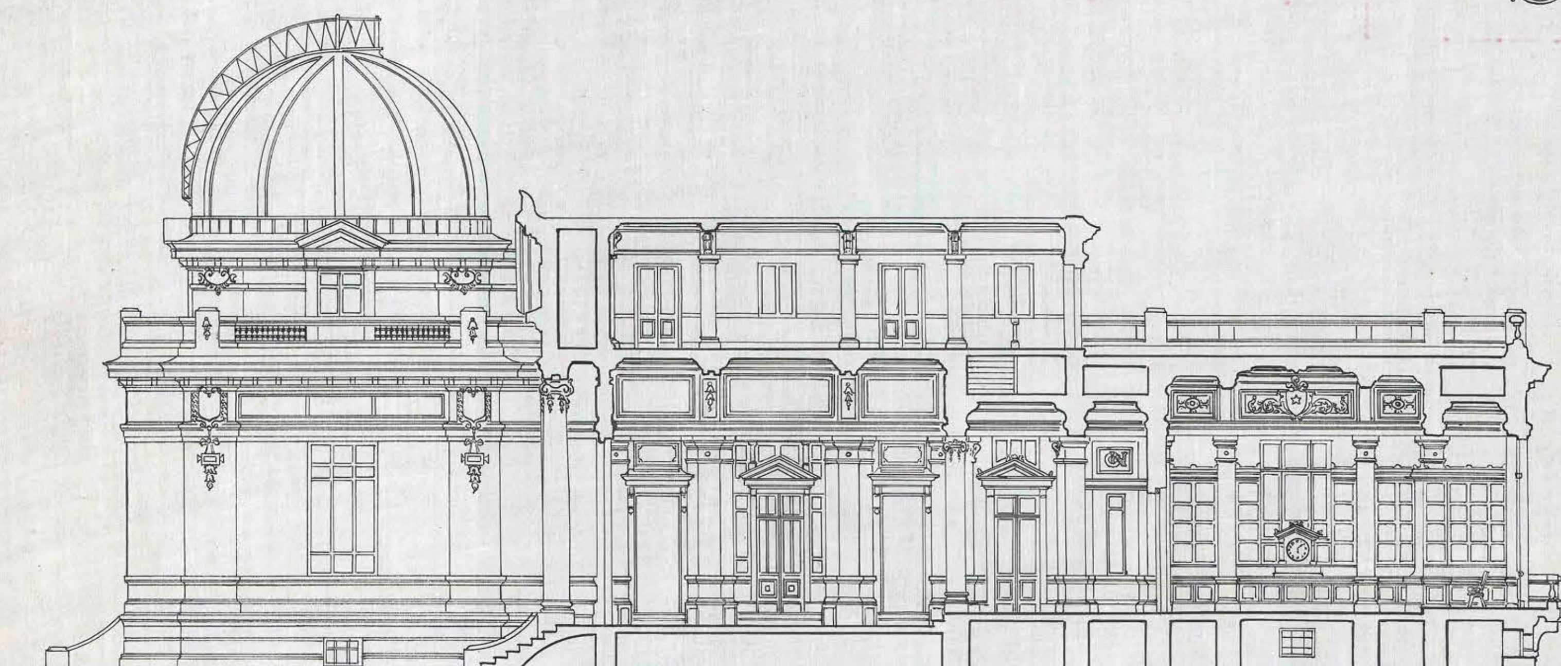
SECCION -CD-
