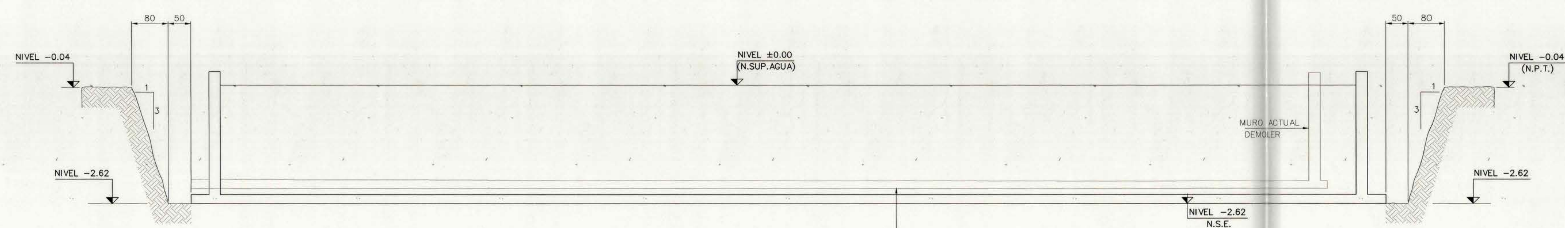
SECCION TRANSVERSAL DE EXCAVACIONES PISCINA SUR ESCALA 1:50
