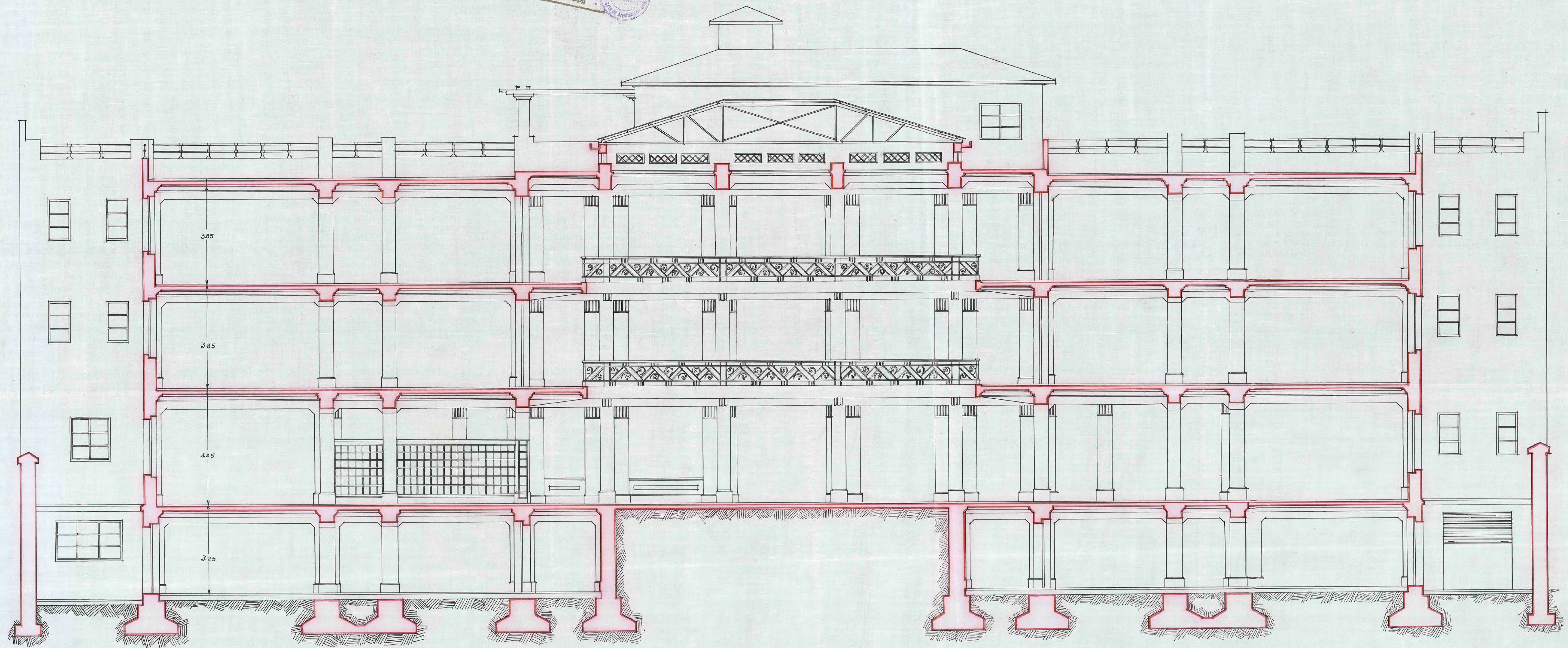
CORTE - TRANSVERSAL.
