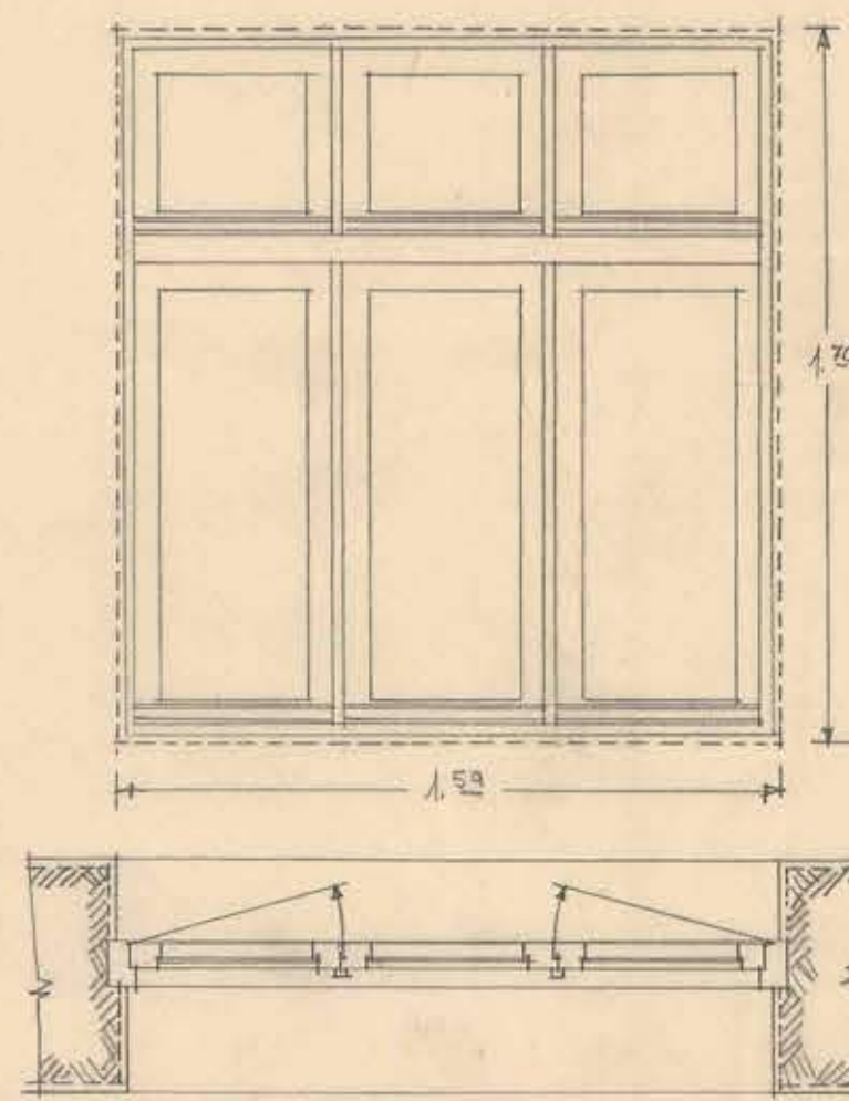
VENTANA/ TIPO "F". /ON 4.
