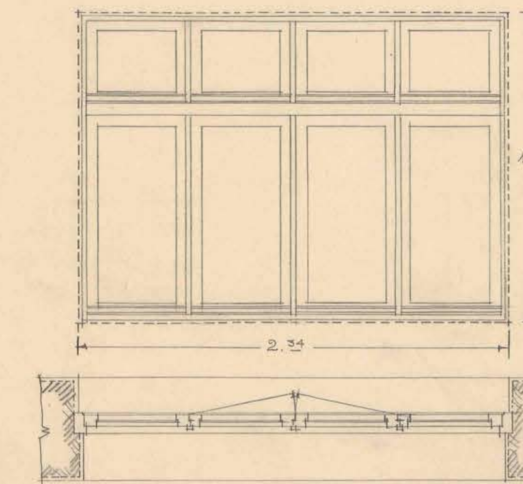
VENTANA/ TIPO "E". /ON 4.
