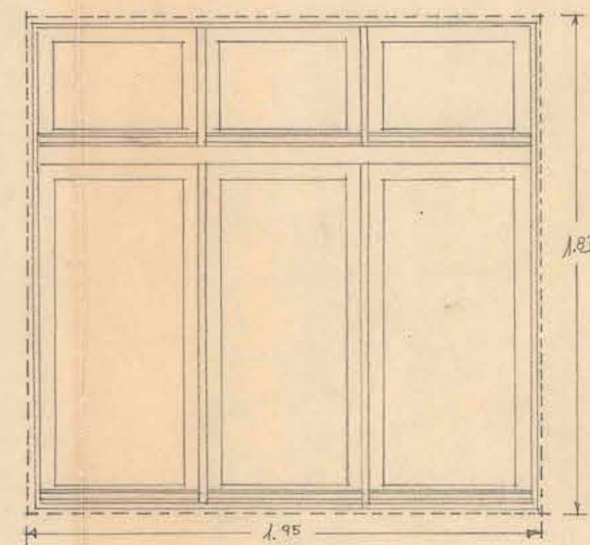
VENTANA TIPO "G". E/ 1.
