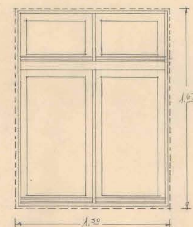
VENTANA TIPO "E". E/ 1.
