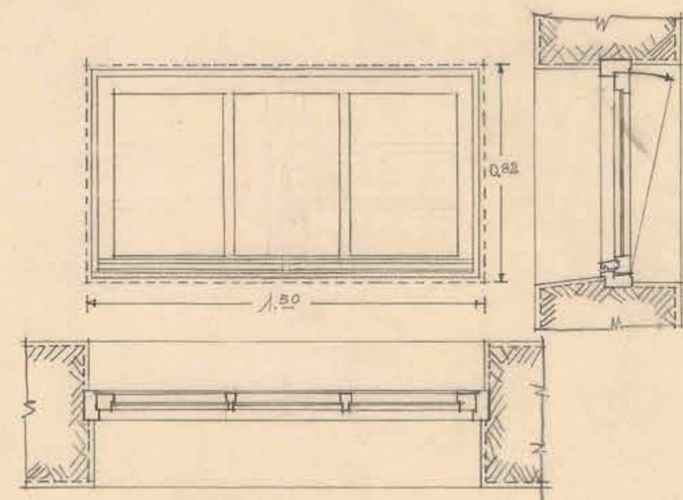
VENTANA/ TIPO "A". /ON 8.
