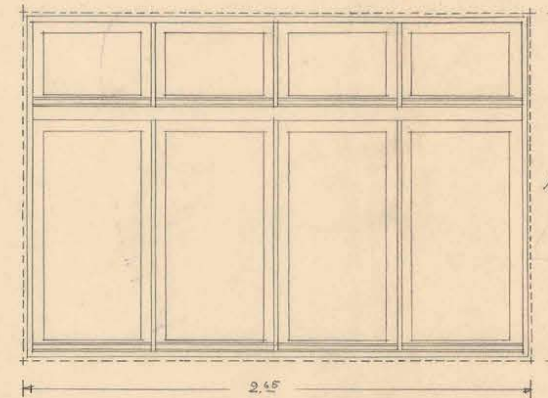
VENTANA TIPO "D". E/ UNA.
