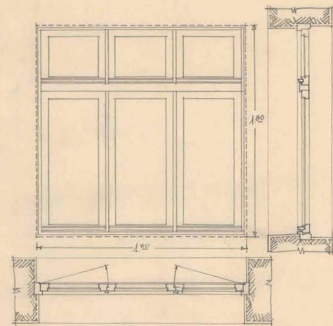
VENTANA TIPO "C". E/ UNA.
