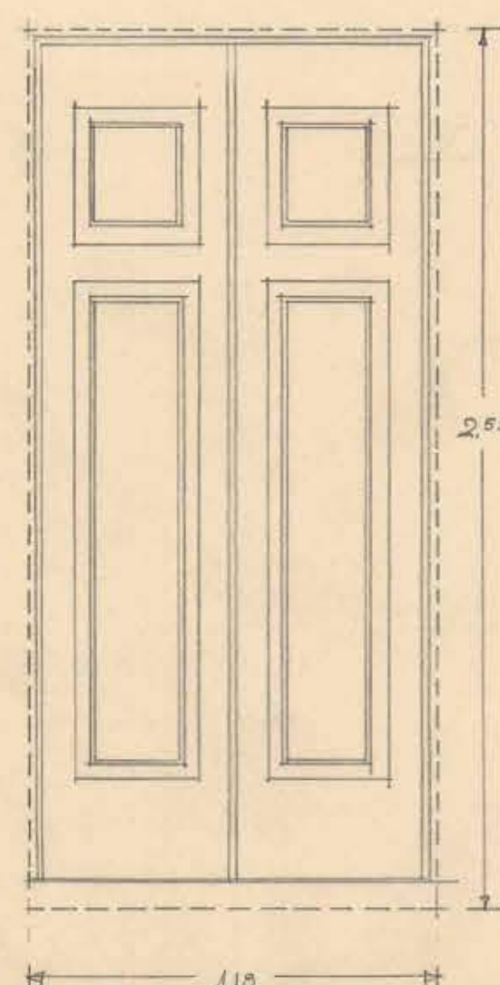
PUERTA TIPO "7" E/ UNA.
