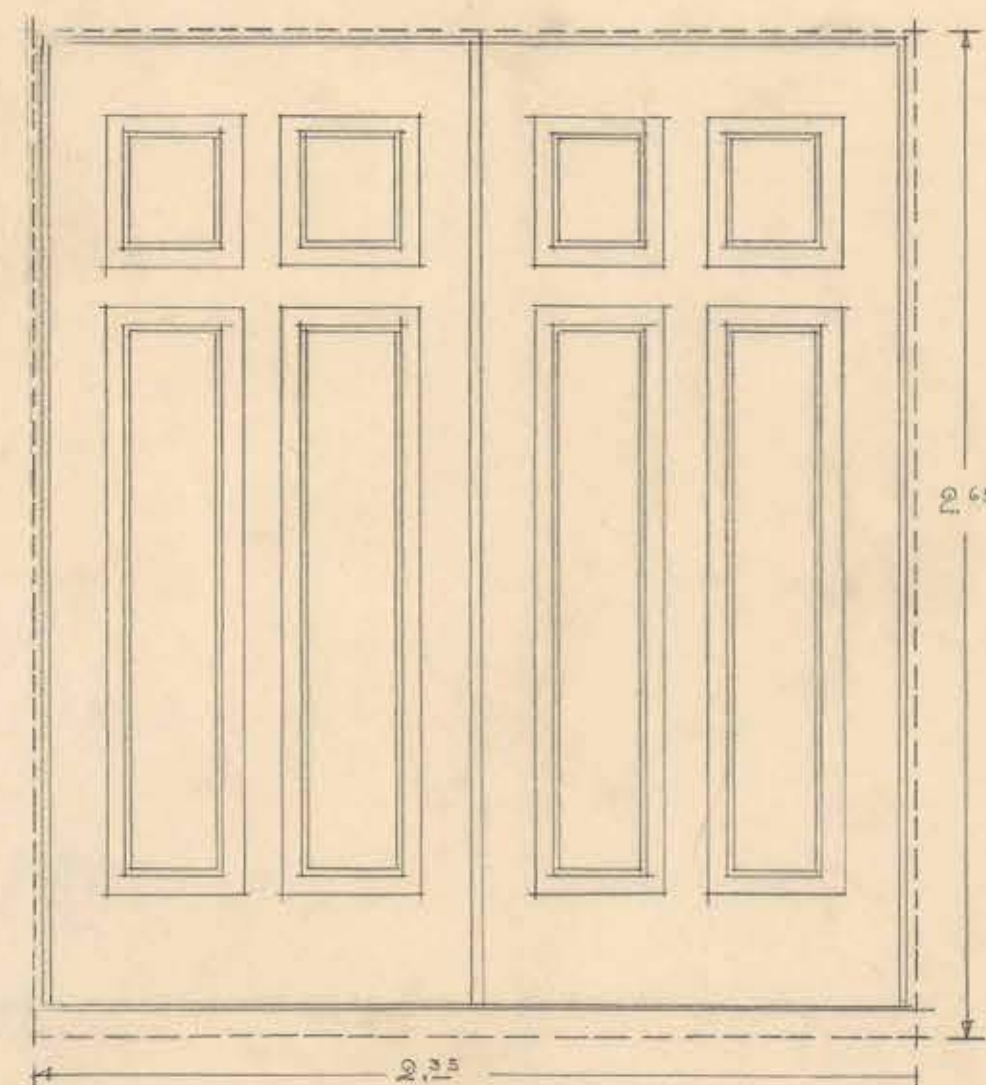
PUERTA TIPO "6" E/ UNA.
