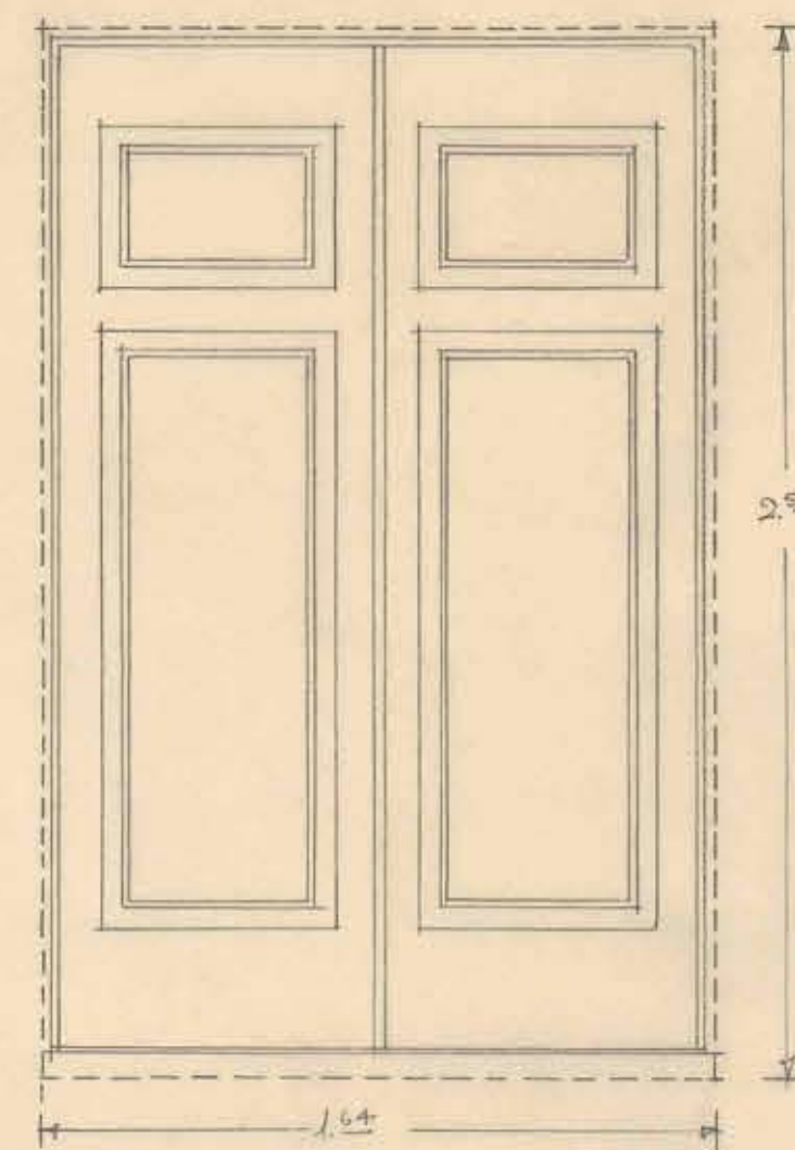
PUERTA TIPO "4" E/ UNA
