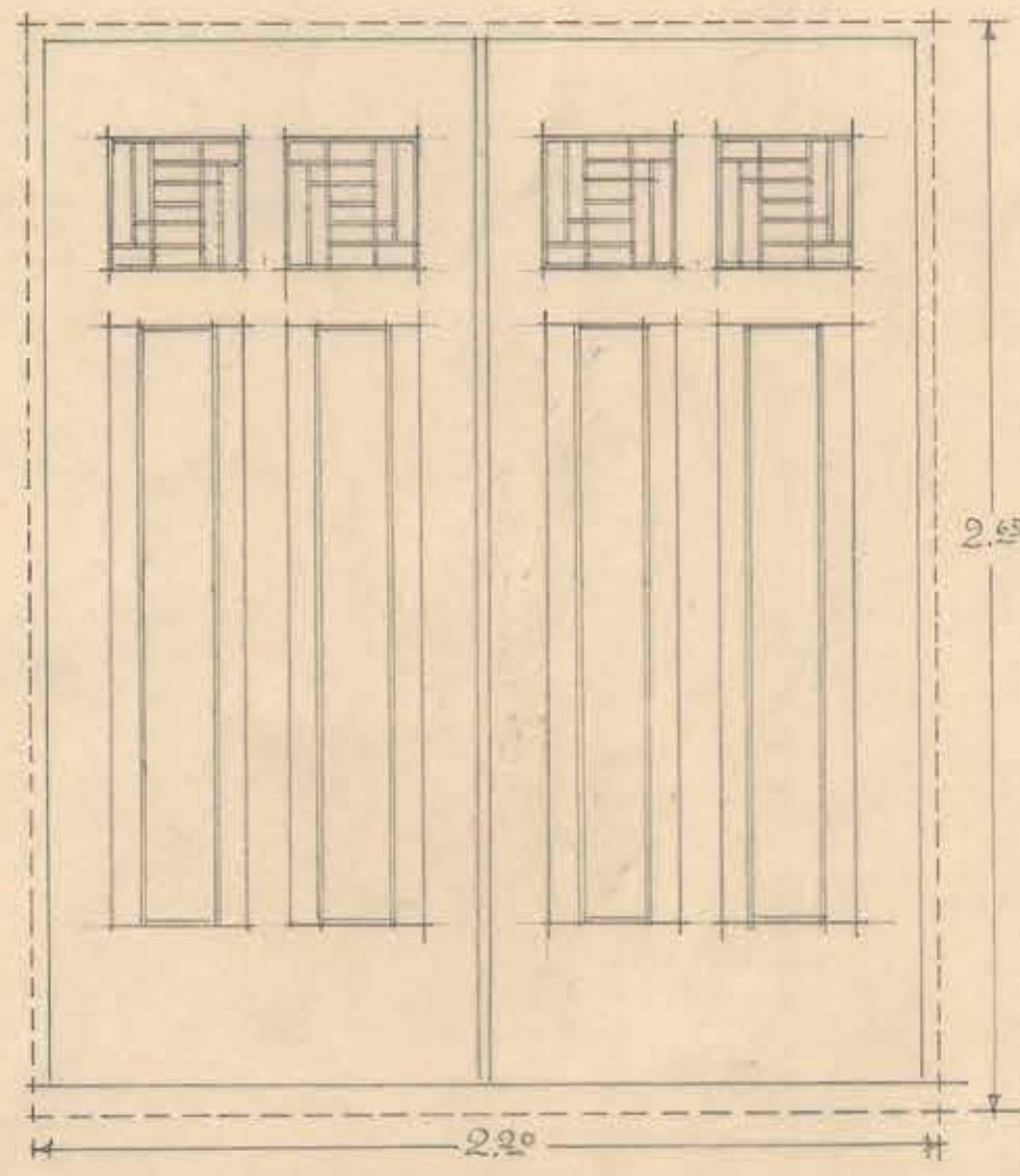
PUEERTA TIPO "f" - E/ UNA.
