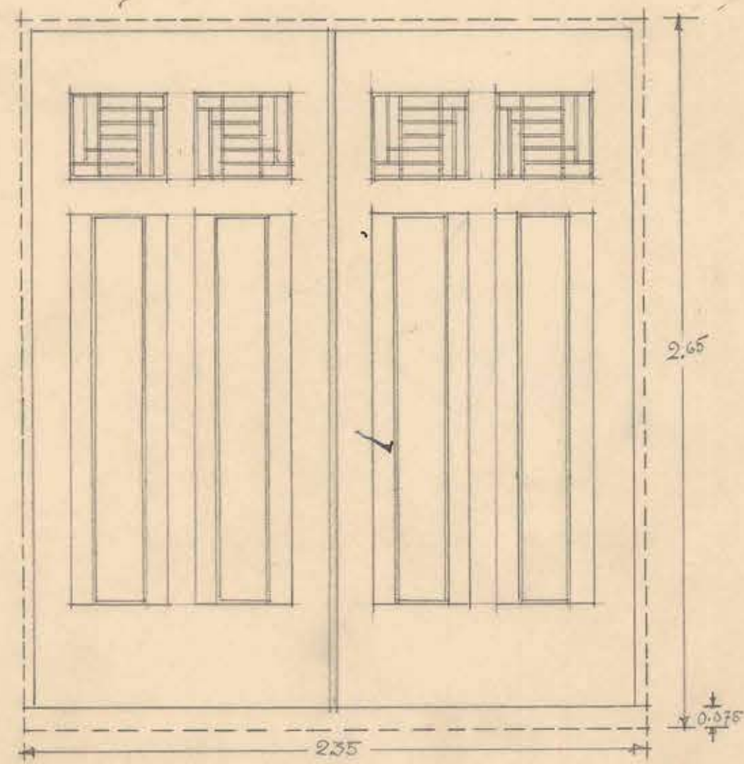
PUEERTA TIPO "h" - E/ UNA.
