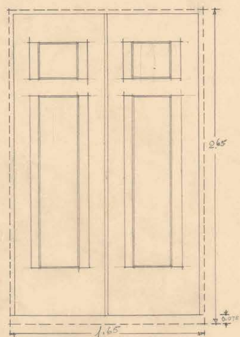
PUEERTA TIPO "g" - E/ UNA.
