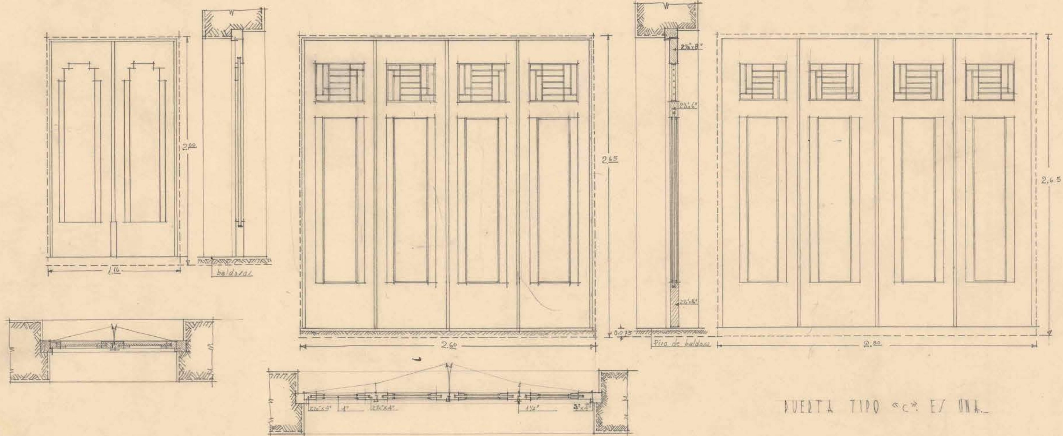
PUEERTA TIPO "a" - ON DOZ.
