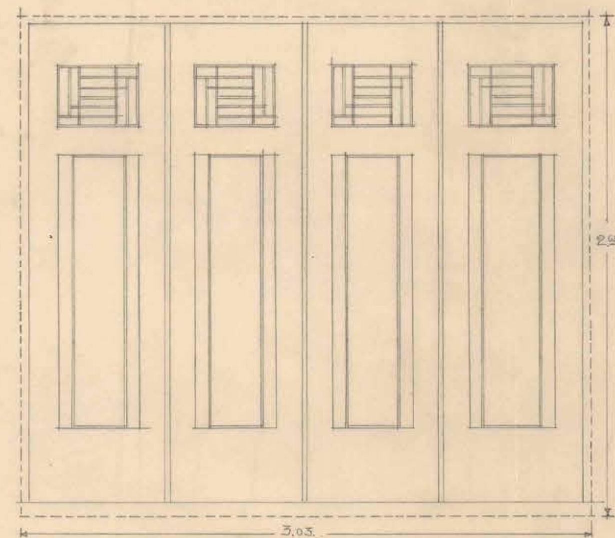
PUEERTA TIPO "d" - E/ UNA.
