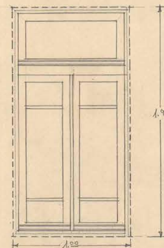
VENTANA/ TIPO "B2" y "B3" / ON 4.
