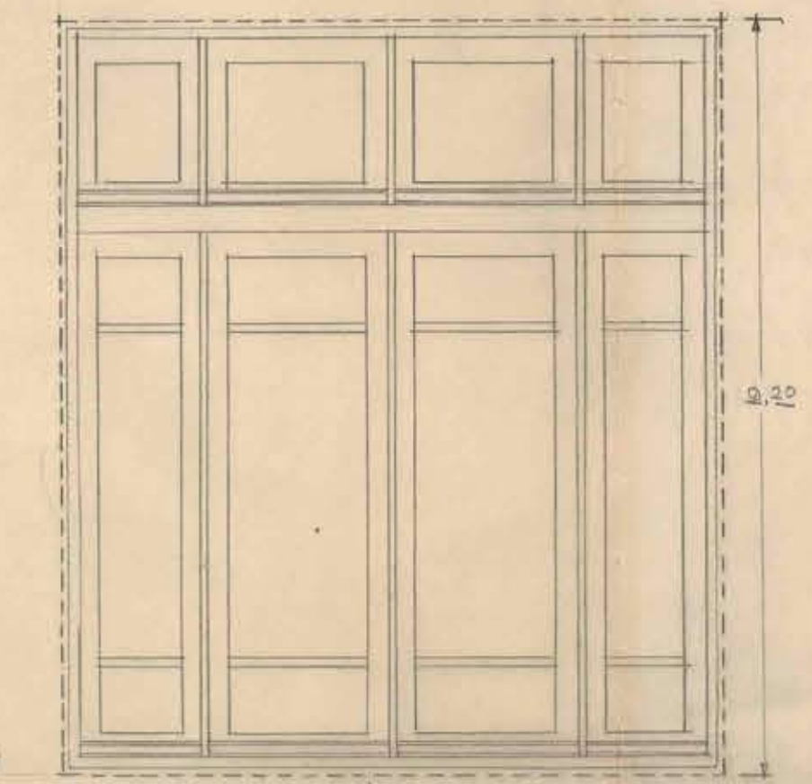
VENTANA/ TIPO "G4" / ON 4.
