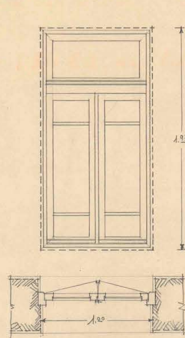
VENTANA/ TIPO "B4" / ON 2.
