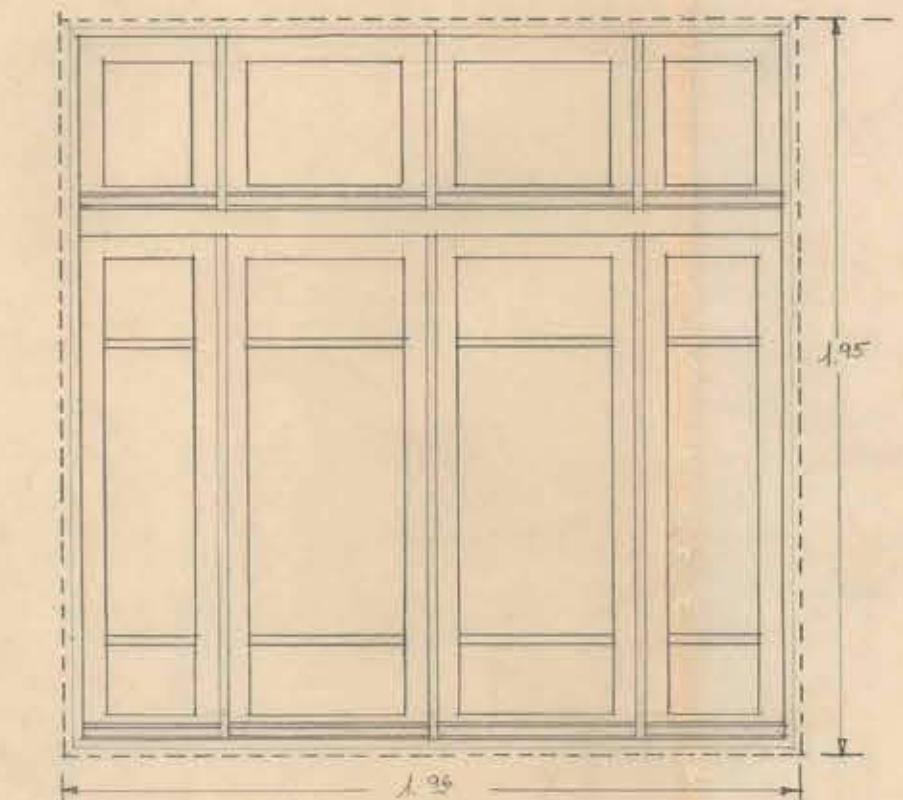
VENTANA/ TIPO "G2" y "G3" / ON 8.
