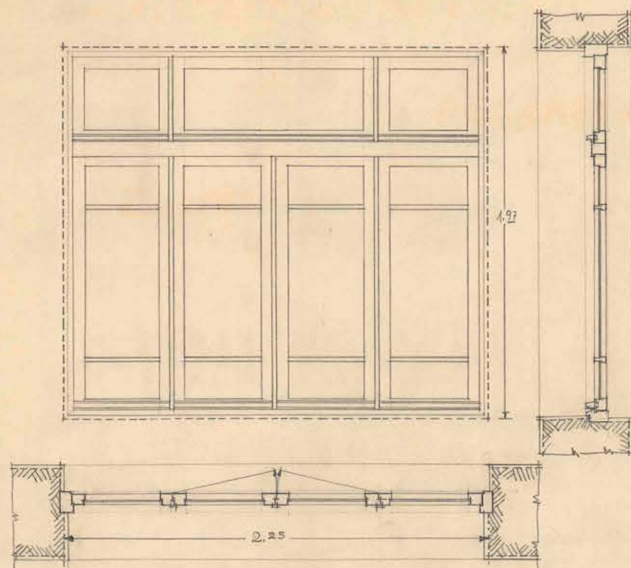
VENTANA/ TIPO "E4" / ON 3.
