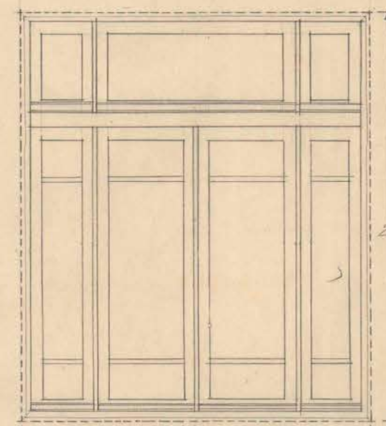
VENTANA/ TIPO "A4" / ON 10.
