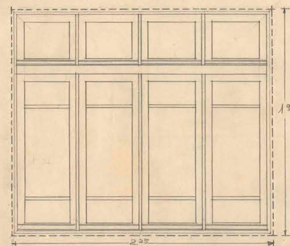
VENTANA/ TIPO "E2" y "E3" / ON 18.
