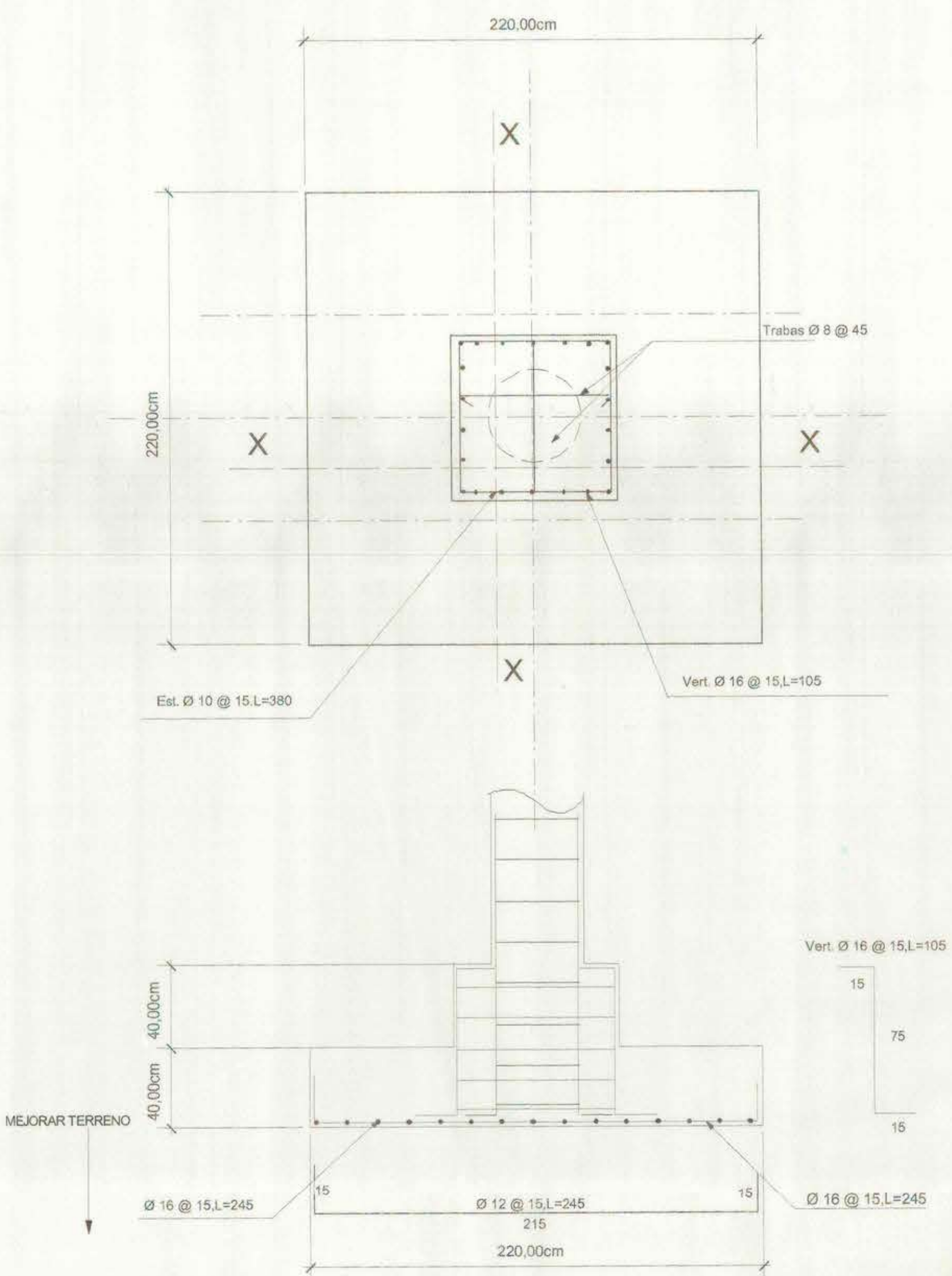
FUNDACIONES ESC. 1:20
