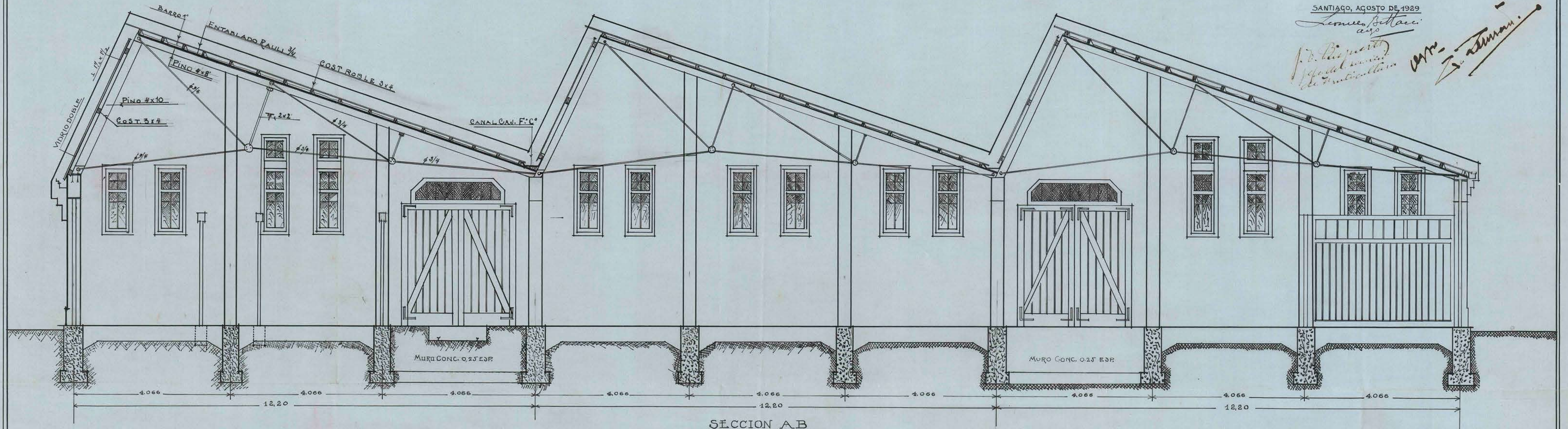
SECCION A-B
