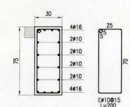
DETALLE VIGA V303 ESC. 1:20
