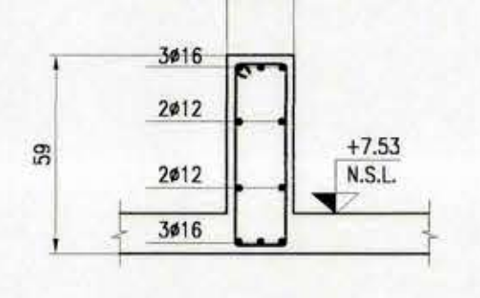
DETALLE VIGA V305 INV. ESC. 1:20
