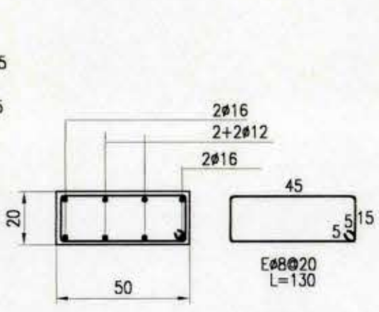
DETALLE PILAR P304 ESC. 1:20
