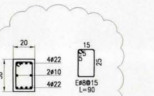
DETALLE PILAR P311 ESC. 1:20
