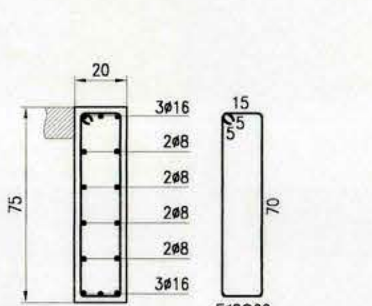
DETALLE VIGA V302 ESC. 1:20
