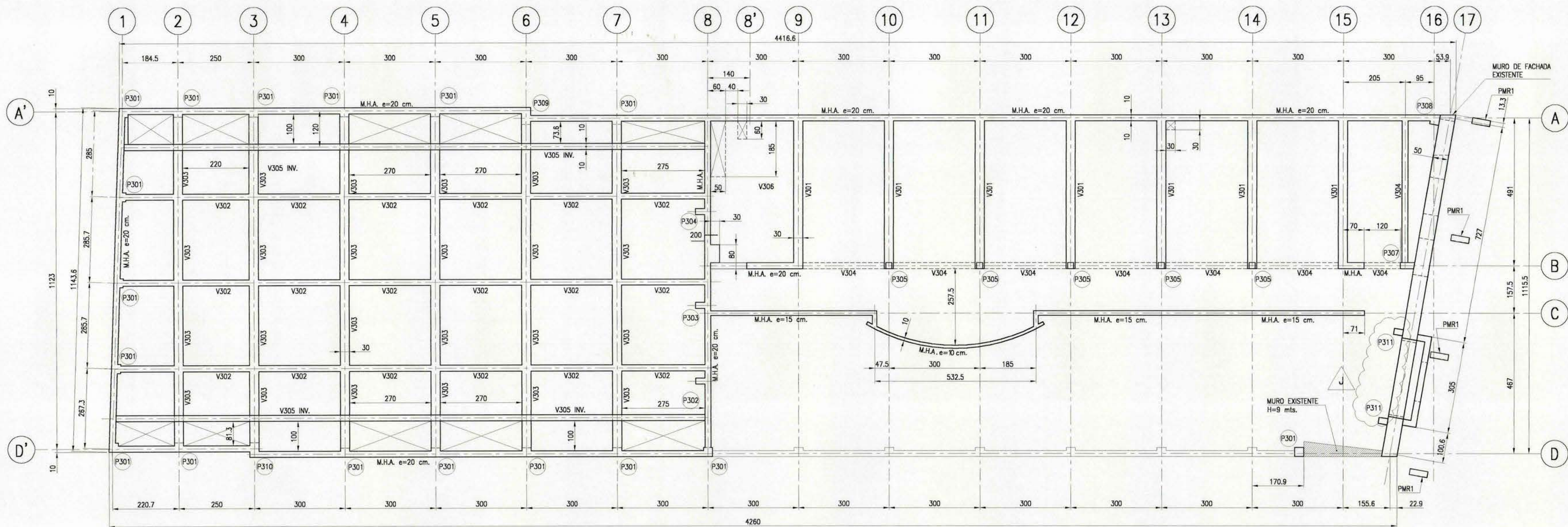
PLANTA DE ESTRUCTURA 3° PISO ESC. 1:75
