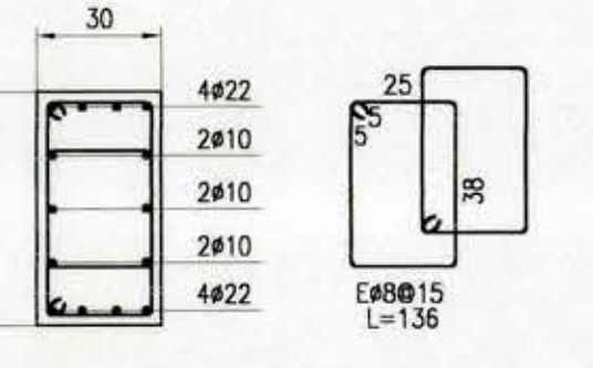
DETALLE PILAR P309 ESC. 1:20
