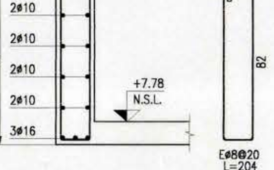
DETALLE VIGA V304 ESC. 1:20
