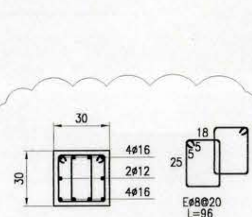
DETALLE PILAR P301 ESC. 1:20
