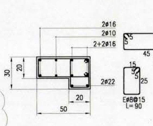
DETALLE PILAR P302 ESC. 1:20
