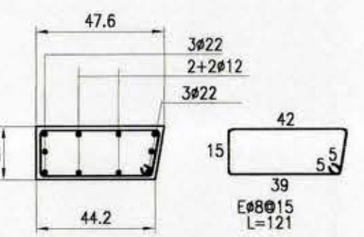
DETALLE PILAR P307 ESC. 1:20
