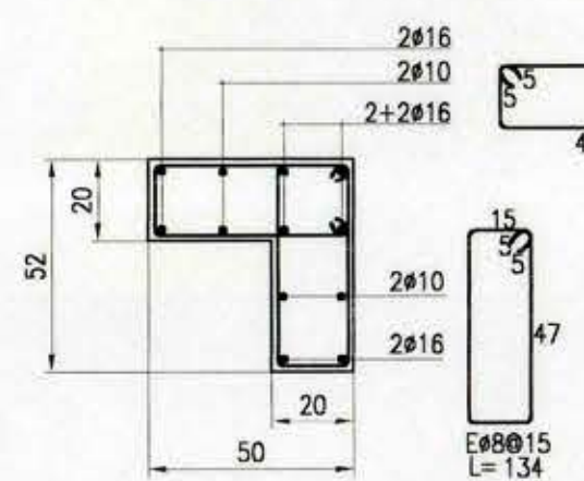
DETALLE PILAR P303 ESC. 1:20
