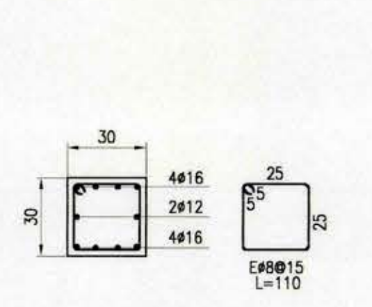
DETALLE VIGA V301 ESC. 1:20
