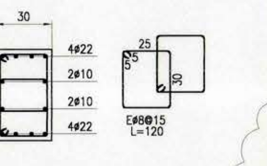
DETALLE PILAR P310 ESC. 1:20
