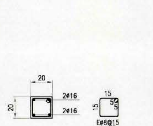
DETALLE PILAR P305 ESC. 1:20
