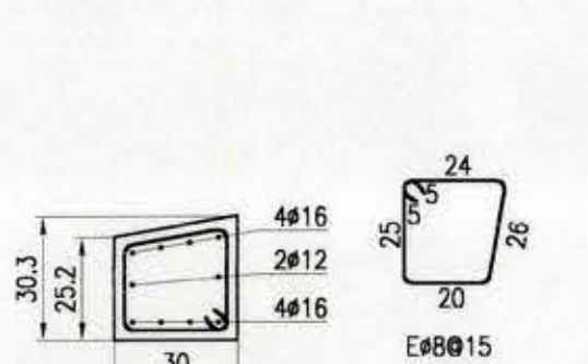
DETALLE PILAR P308 ESC. 1:20
