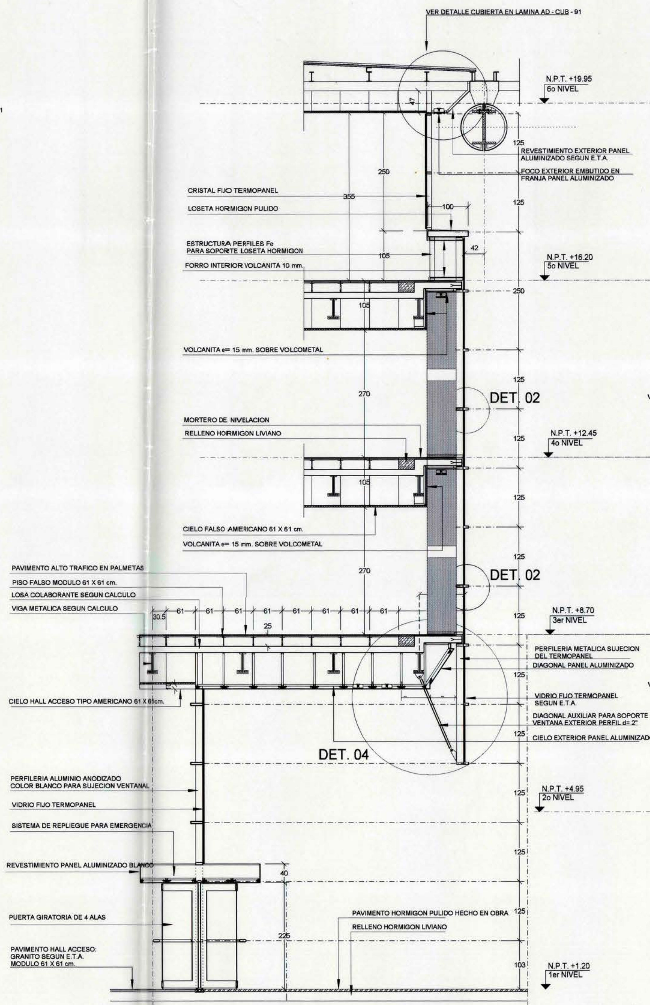
CORTE FACHADA ORIENTE ESCALA 1:50
