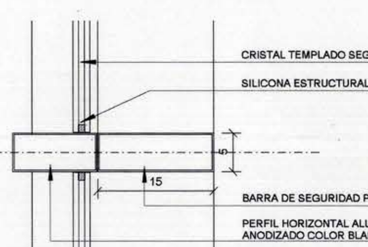
DETALLE 02 ESCALA 1:5
