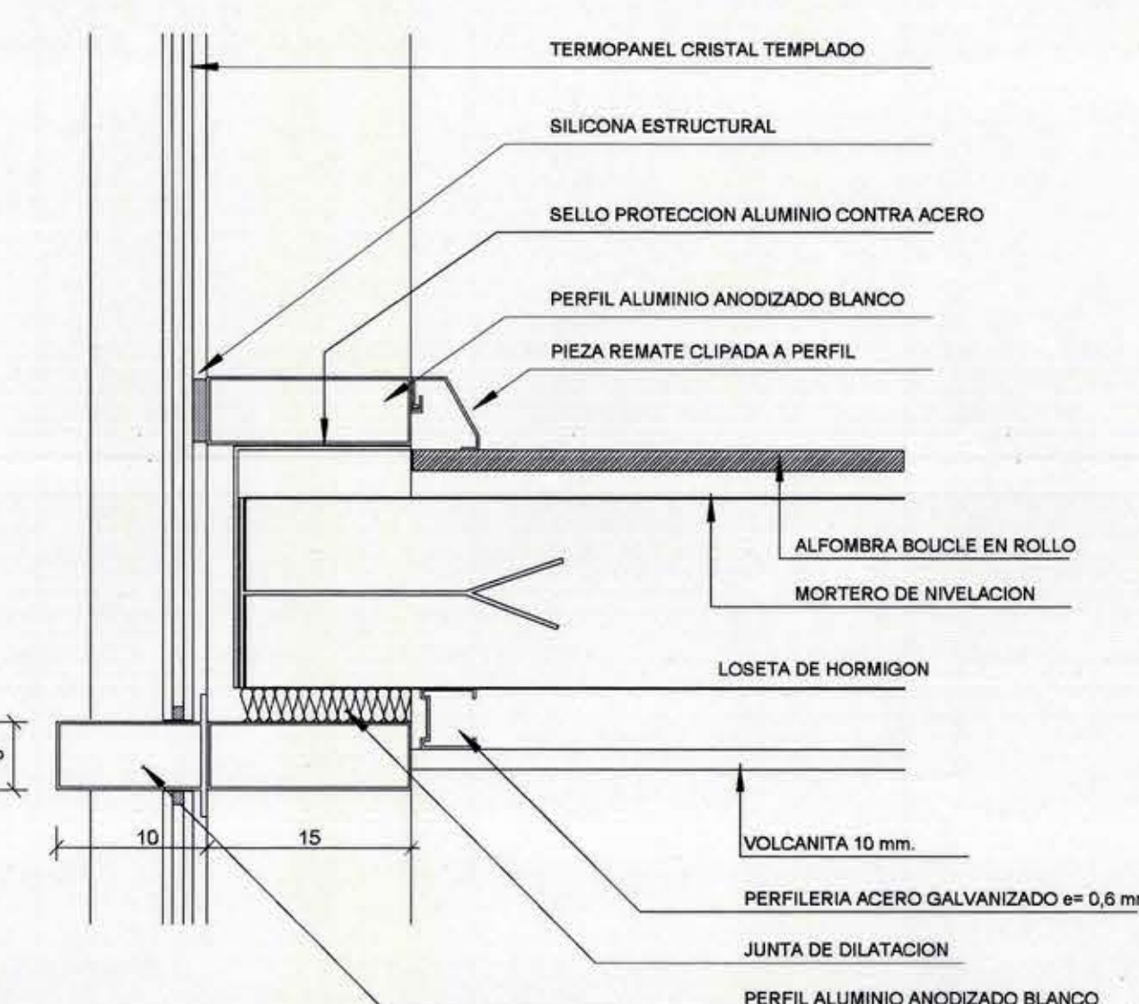
DETALLE 03 ESCALA 1:5
