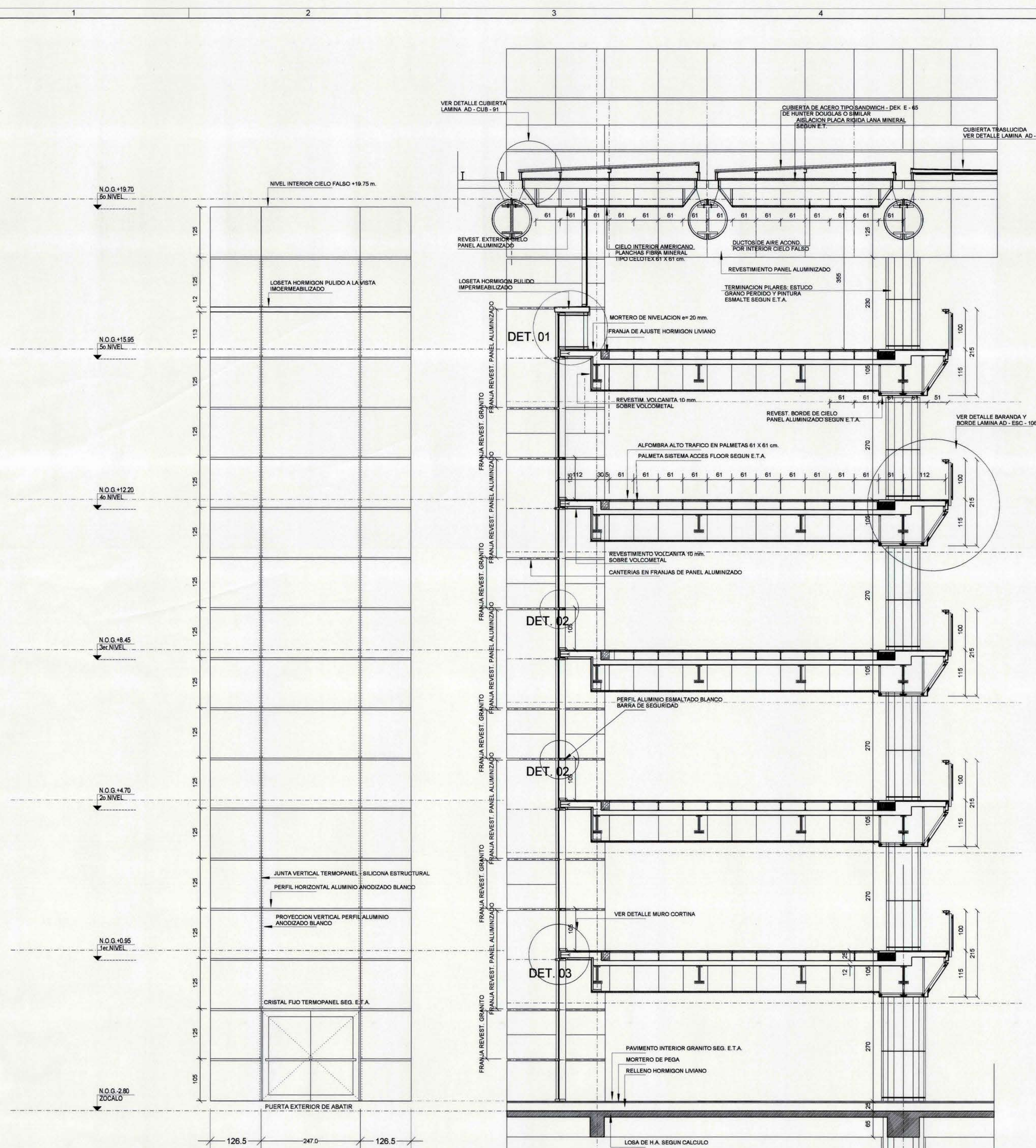
ELEVACION FACHADA PONIENTE ENTRE EJES E y F ESCALA 1:50
