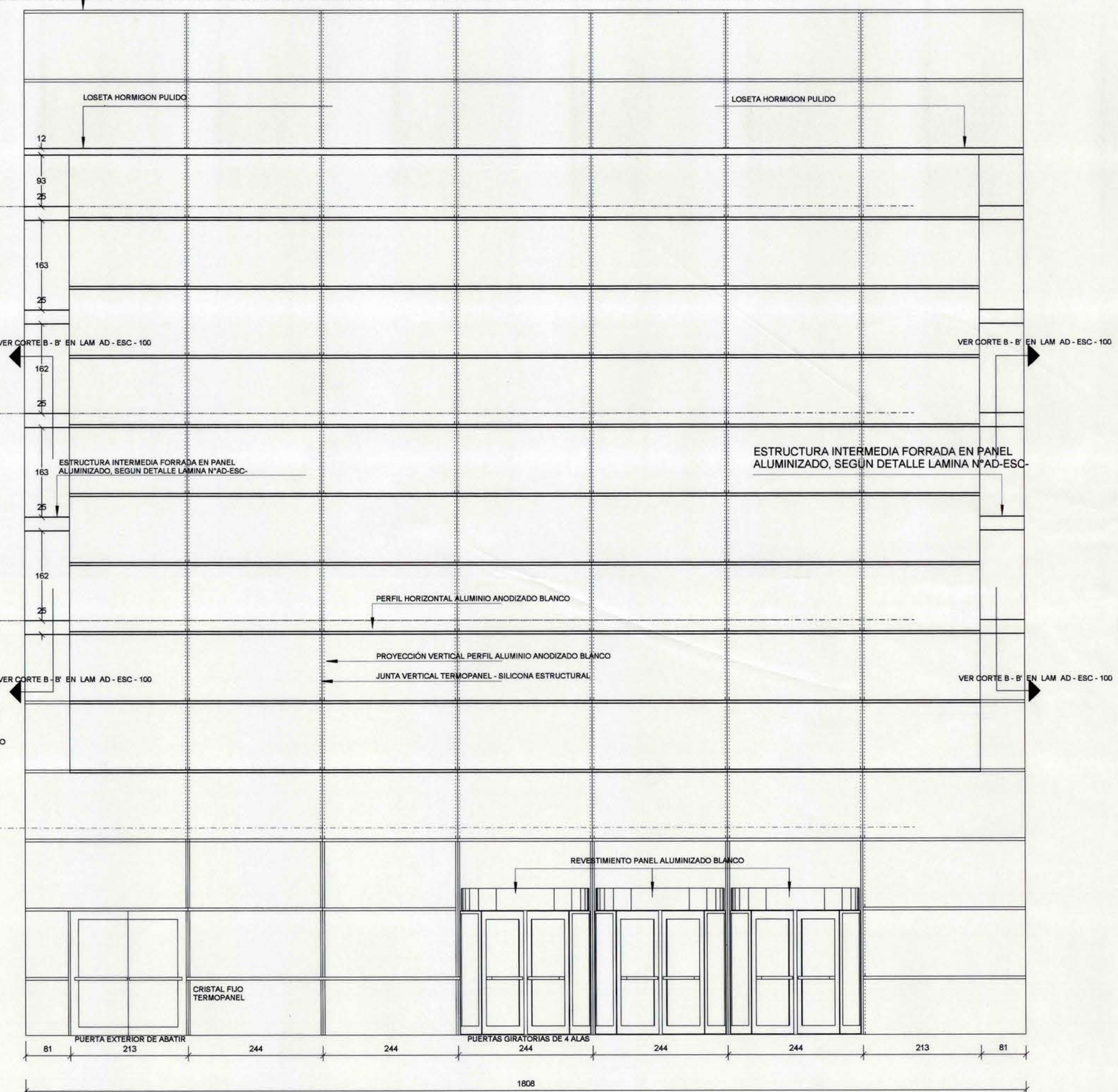
ELEVACION FACHADA ORIENTE ENTRE EJES D y F ESCALA 1:50
