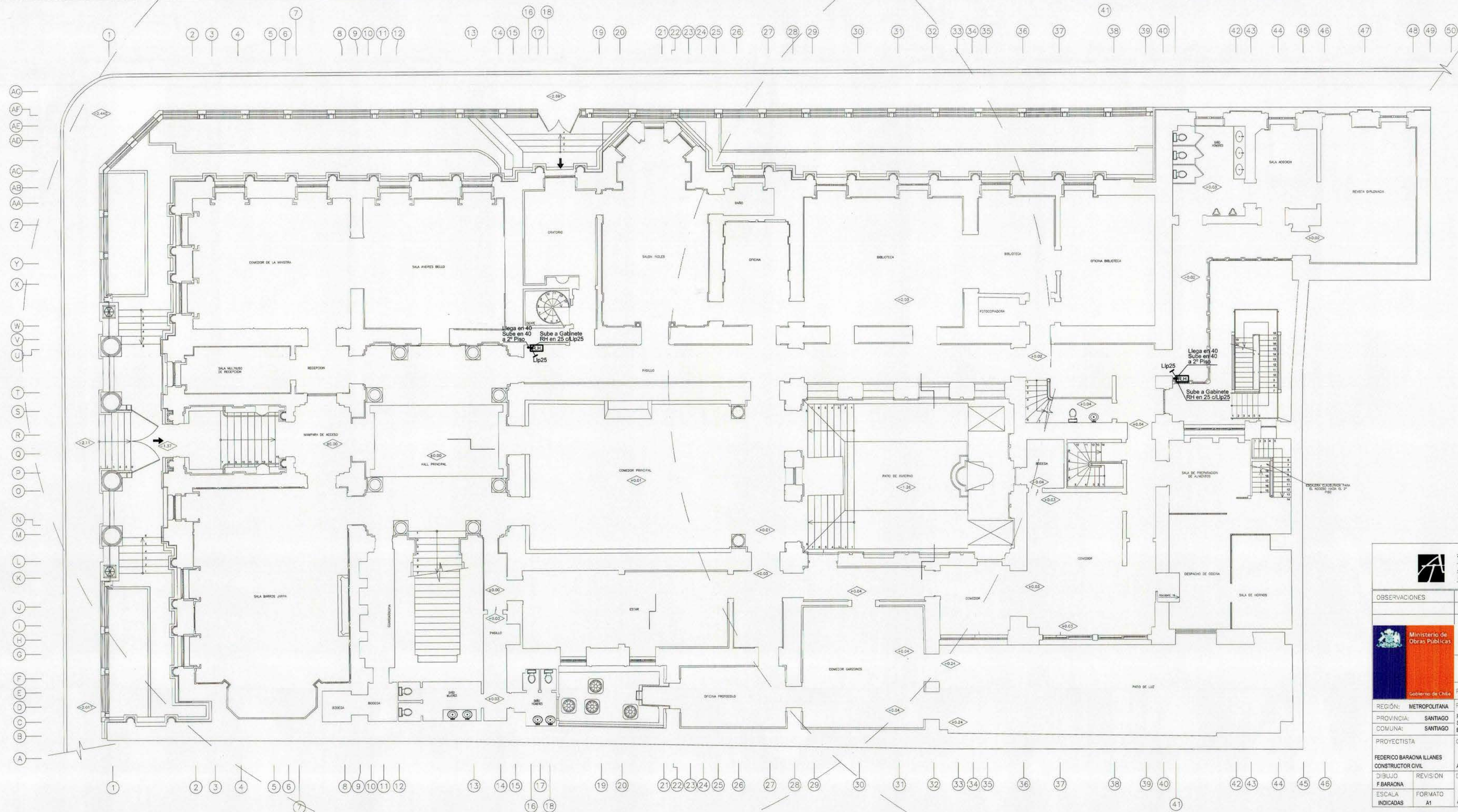
PLANTA PRIMER PISO AGUA FRIA ESC. 1 : 100
