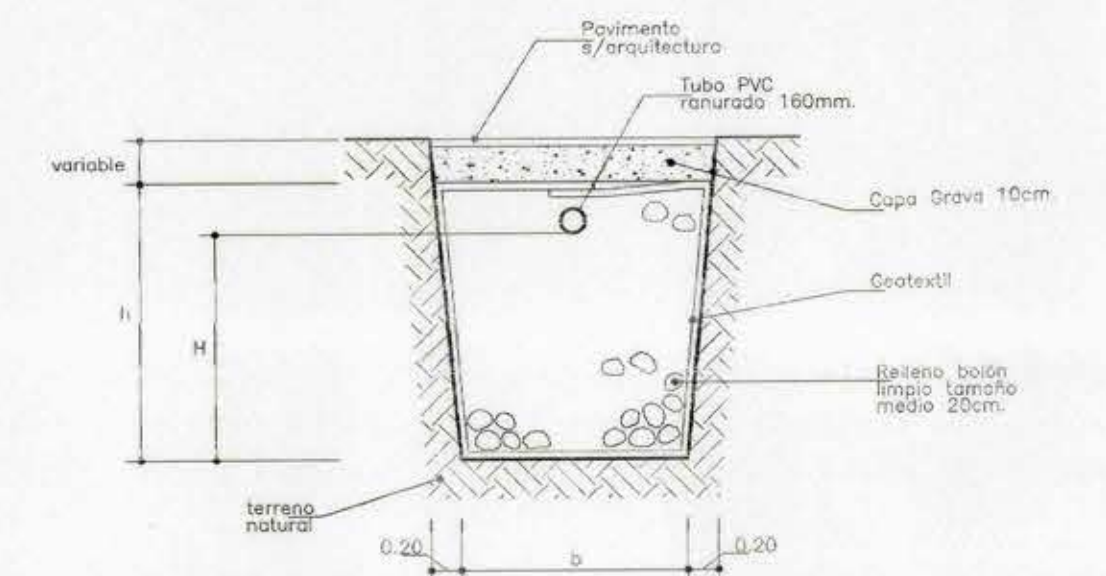
DETALLE ZANJA ABSORCION A. LLUVIA escala 1/50
