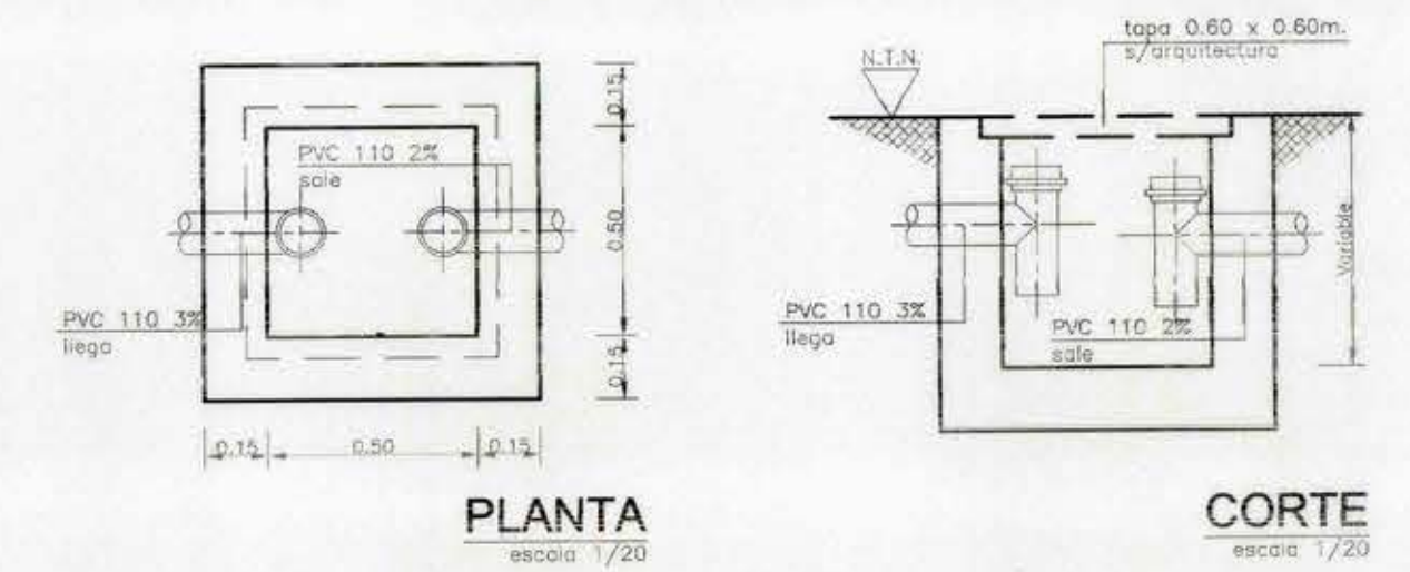
DETALLE CAMARA SUMIDERO
