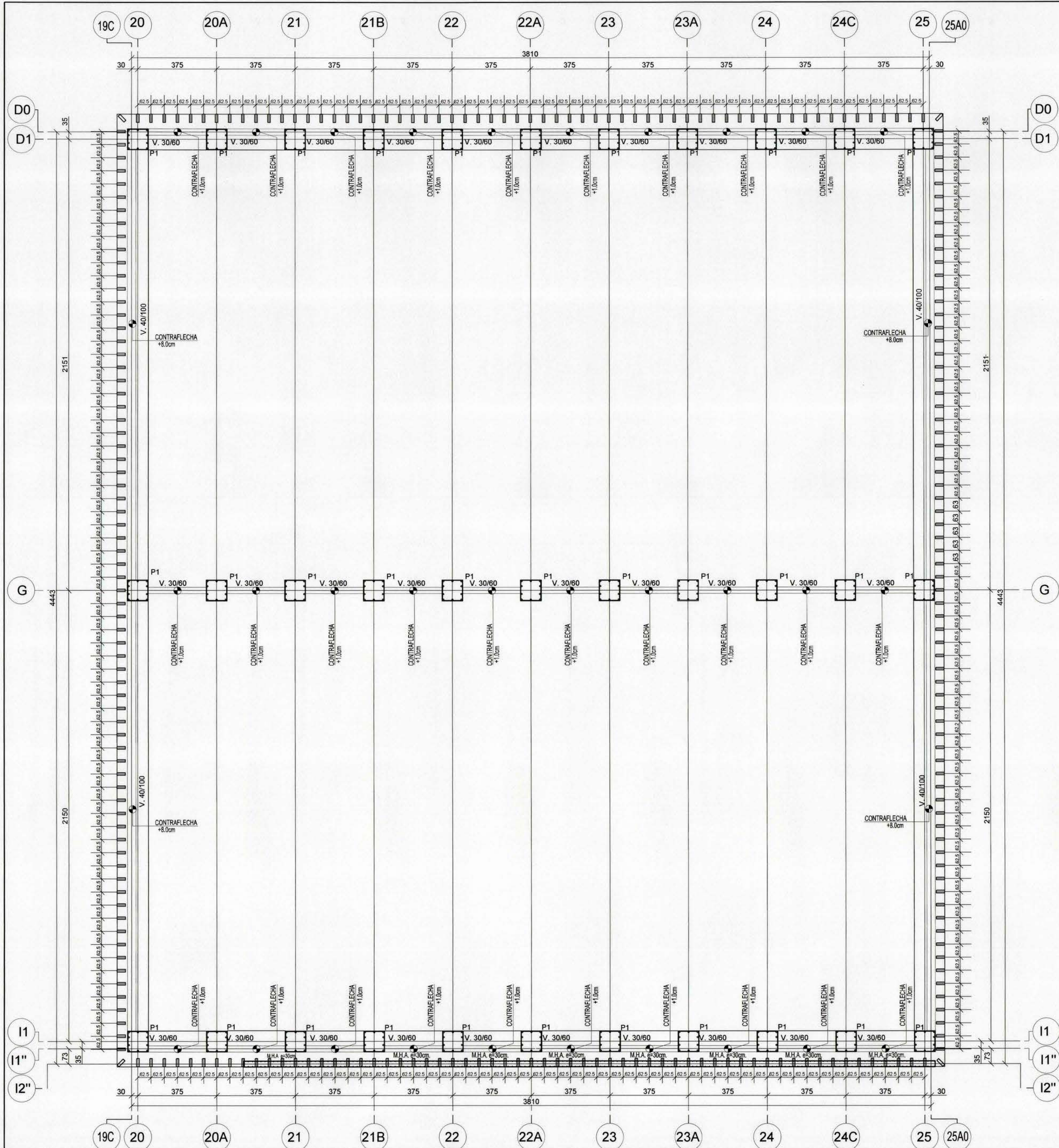
MULTICANCHA PLANTA DE ESTRUCTURAS CIELO PISO CENTRAL ESCALA 1:100
