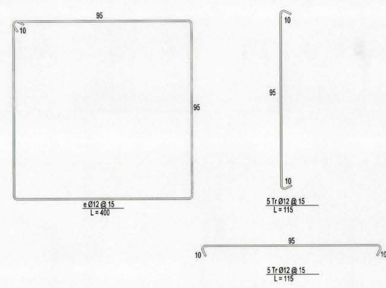
SECCION P1 100/100 ESCALA 1:12.5
