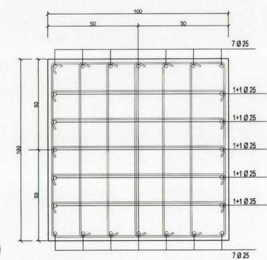
SECCION P1 100/100 ESCALA 1:12.5
