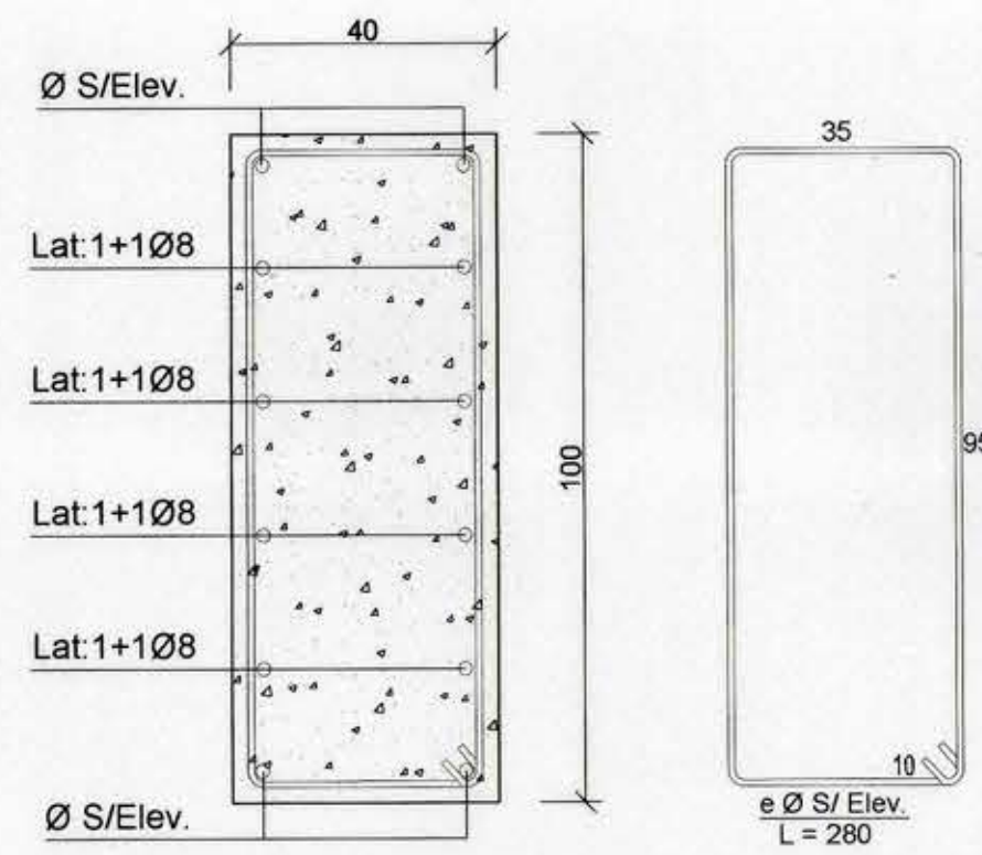
SECCION V. 40/100 ESCALA 1:12.5
