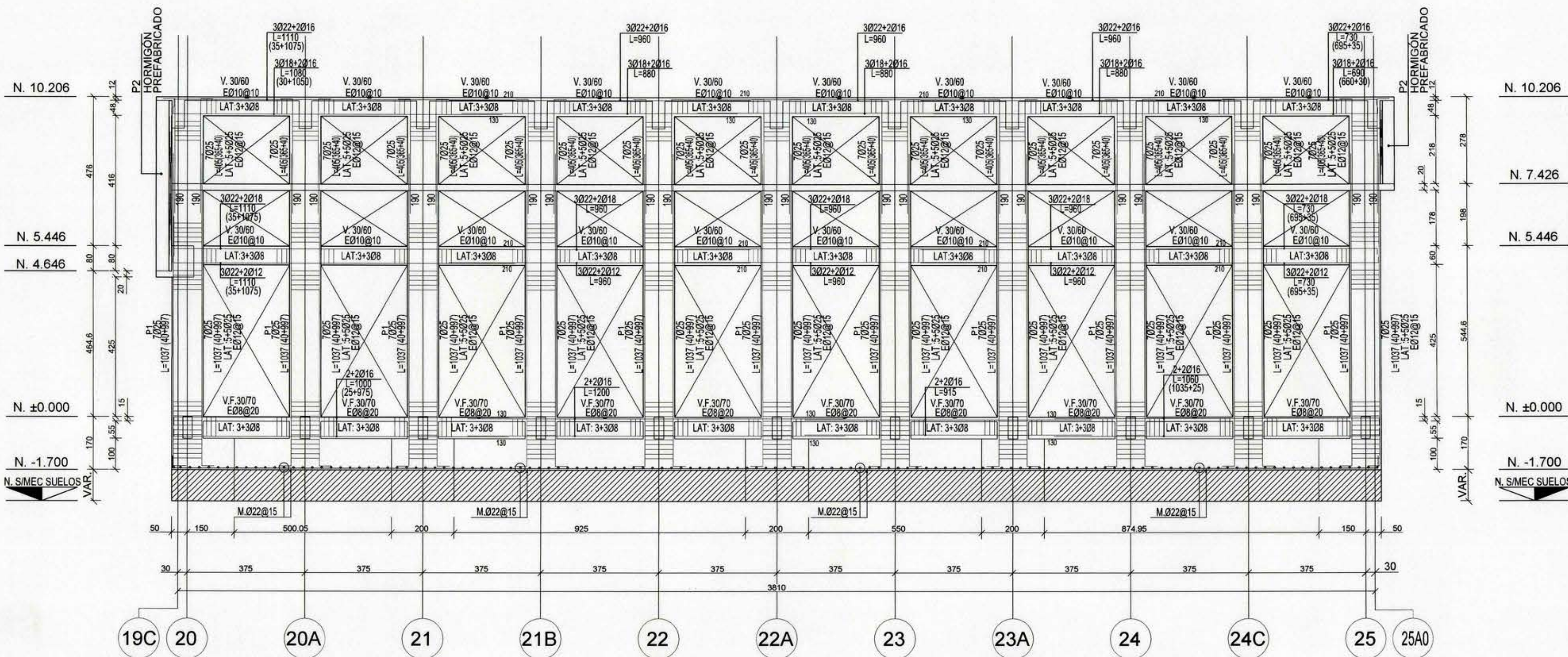
ELEVACIÓN DE EJE D1
