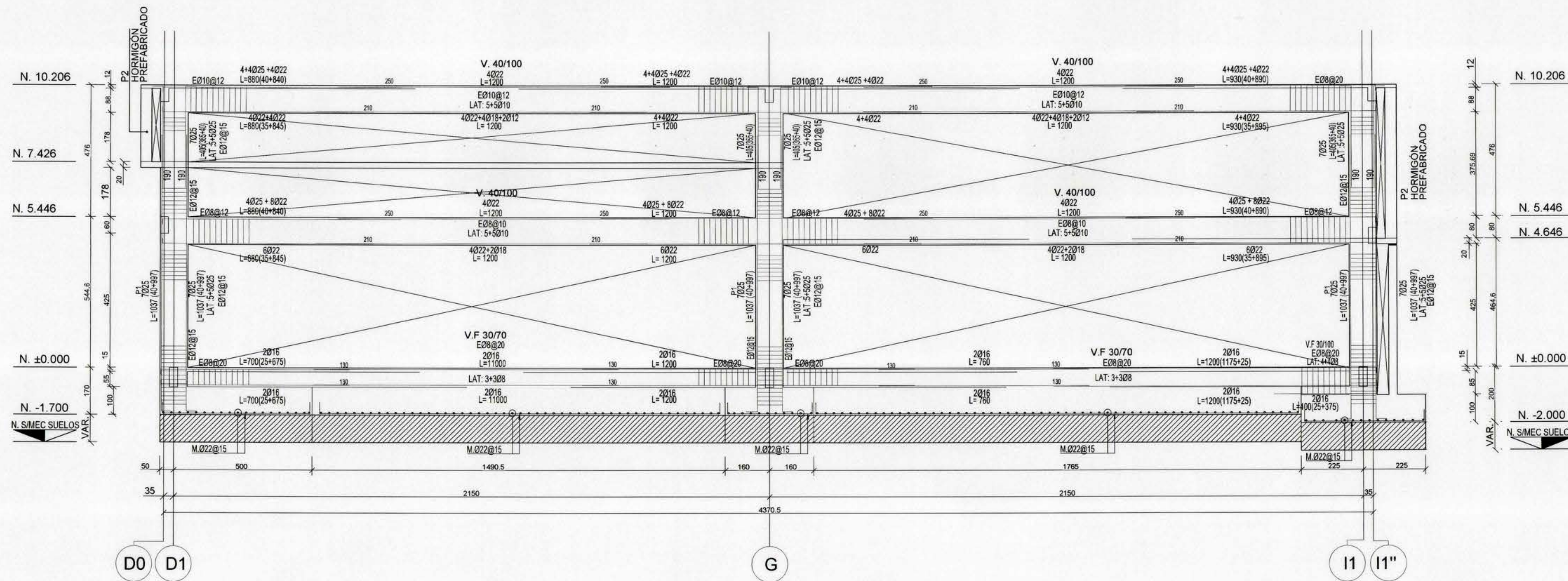
ELEVACIÓN DE EJE 25
