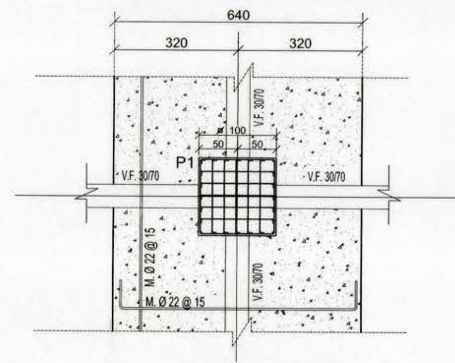
DETALLE F.C.3 ESCALA 1:50
