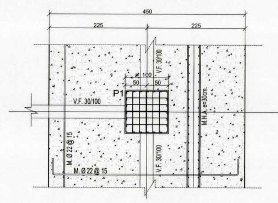
DETALLE F.C.4 ESCALA 1:50
