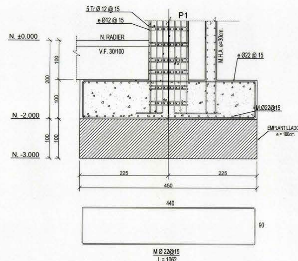
SECCION F.C.4 ESCALA 1:50
