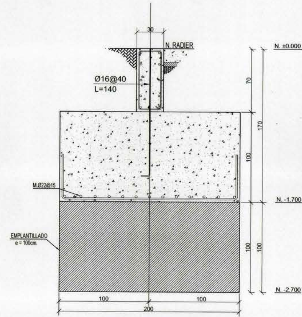
SECCION F.C.1 ESCALA 1:25
