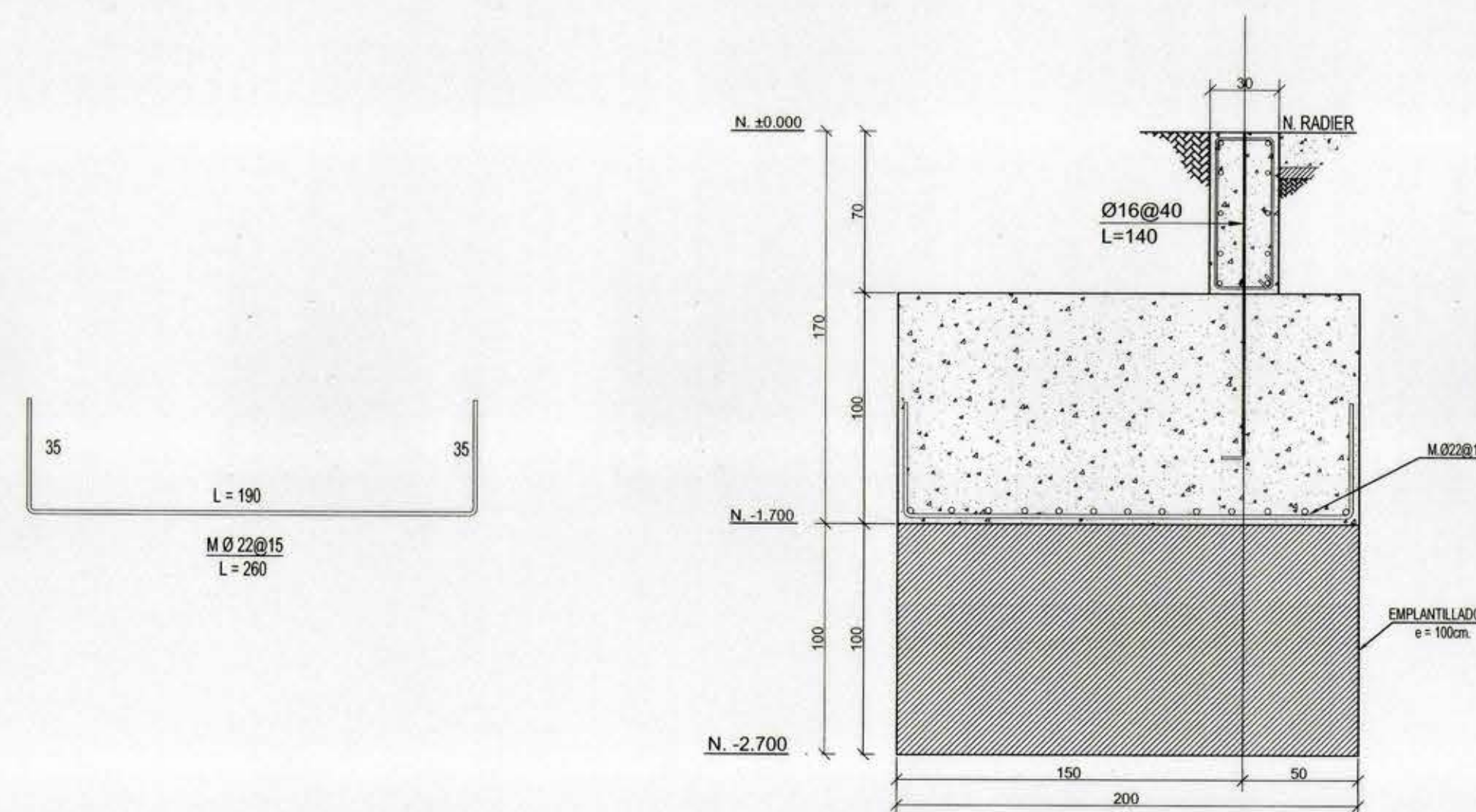
SECCION F.C.2 ESCALA 1:25
