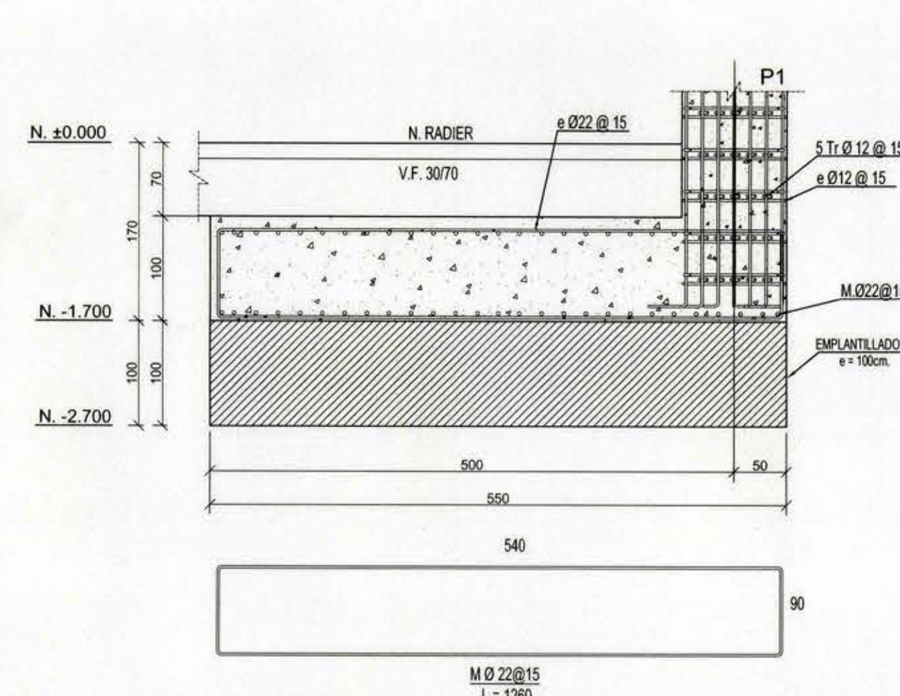
SECCION F.C.5 ESCALA 1:50
