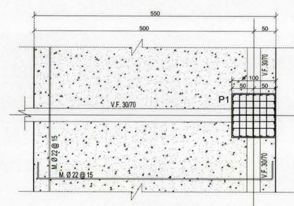
DETALLE F.C.5 ESCALA 1:50
