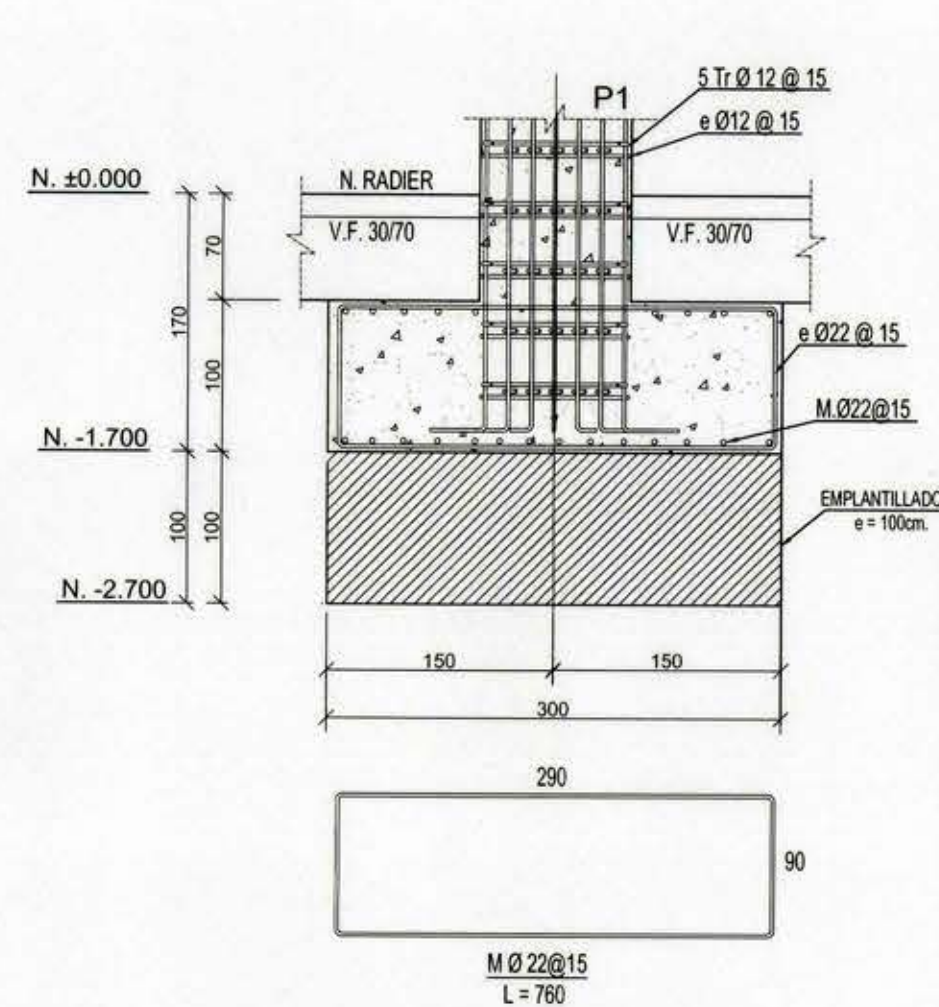
SECCION F.C.3 ESCALA 1:50
