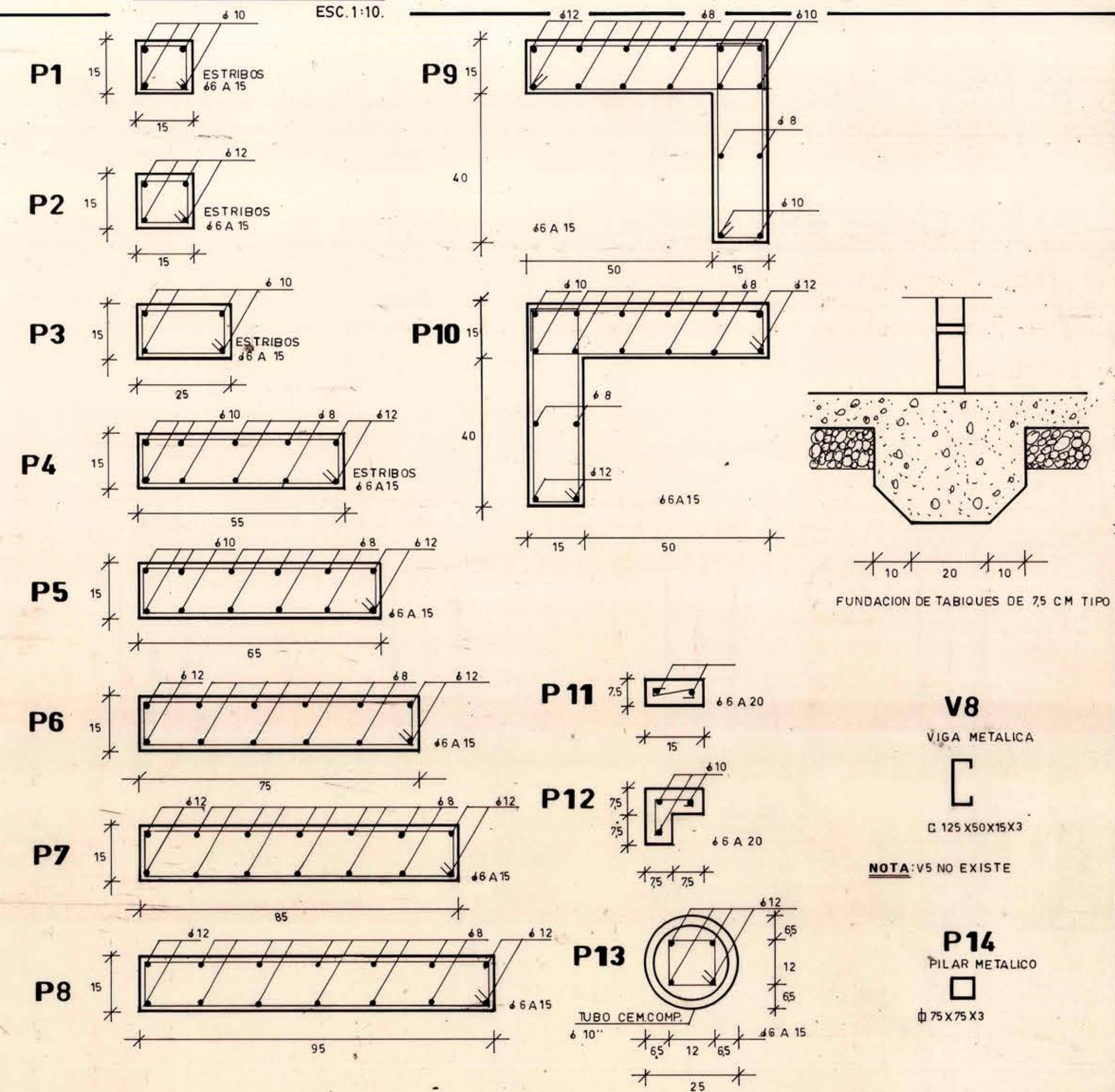
CUADRO PILARES ESC 1:10.
