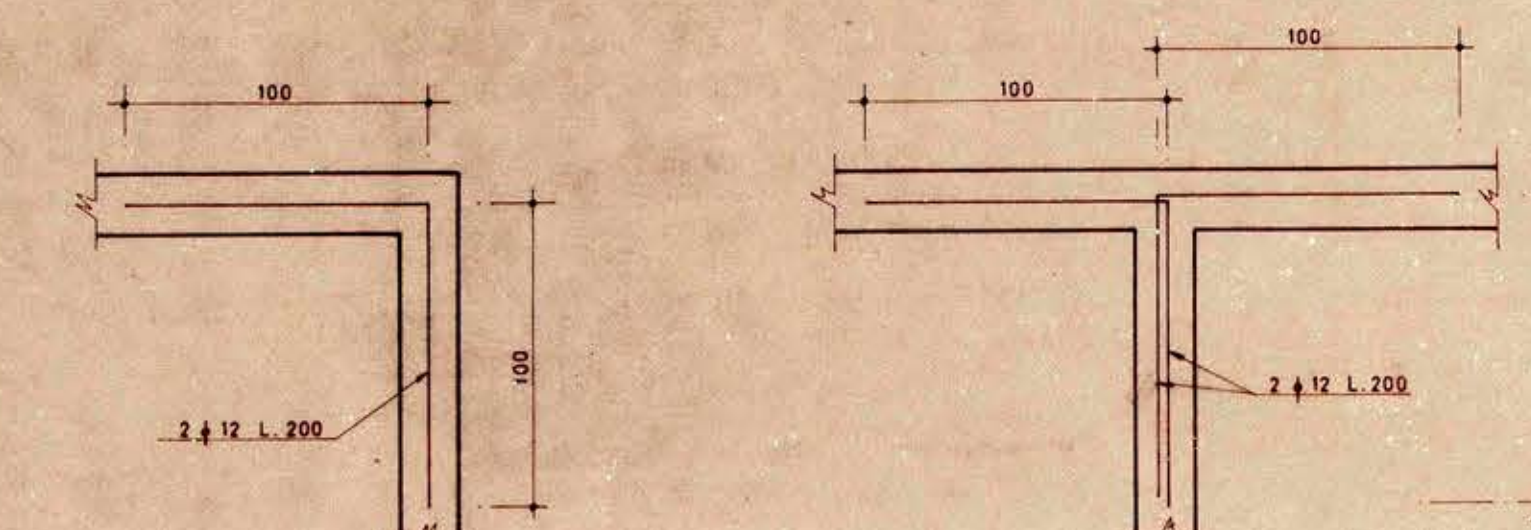
REFUERZOS EN CRUCES DE CADENAS DE FUNDACION
