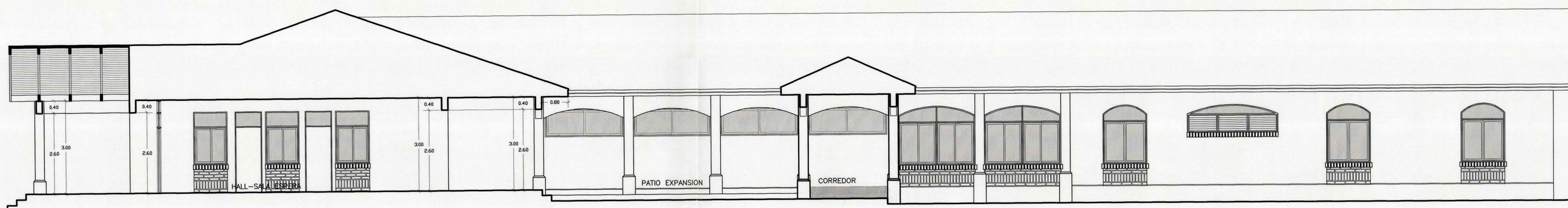
ELEVACION CORTE B-B ESCALA 1:50
