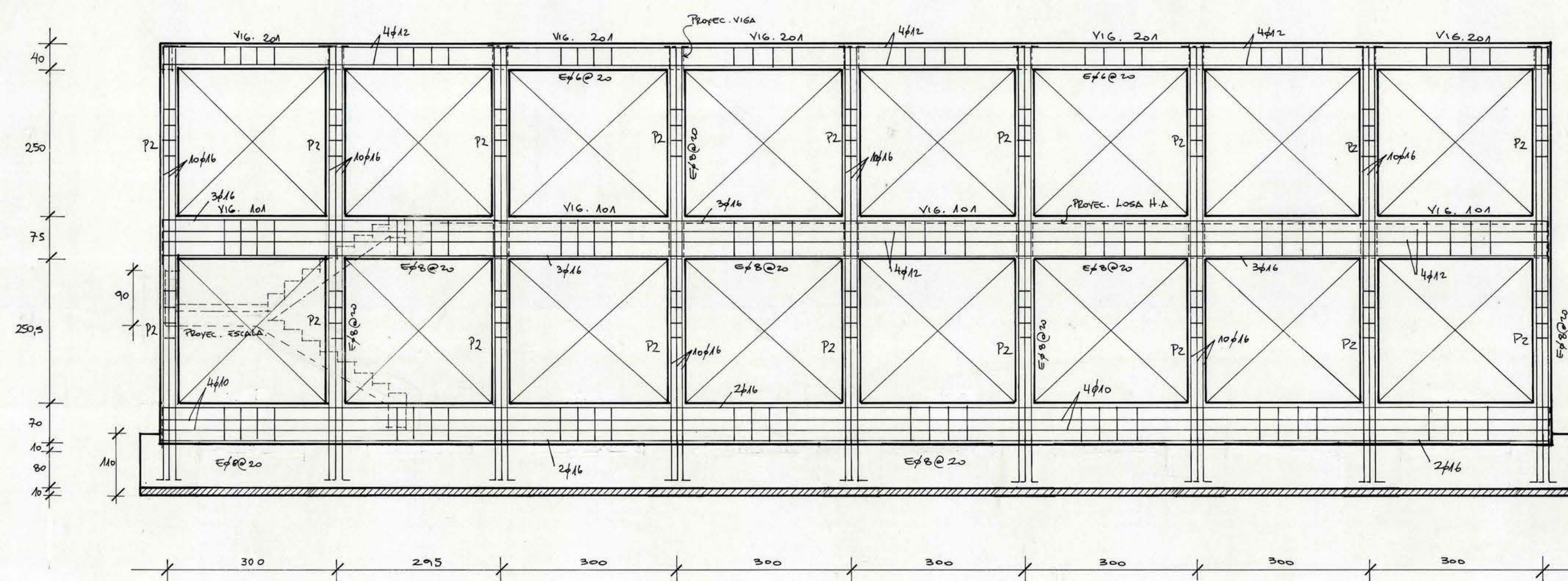
ELEVACION EJE C.
