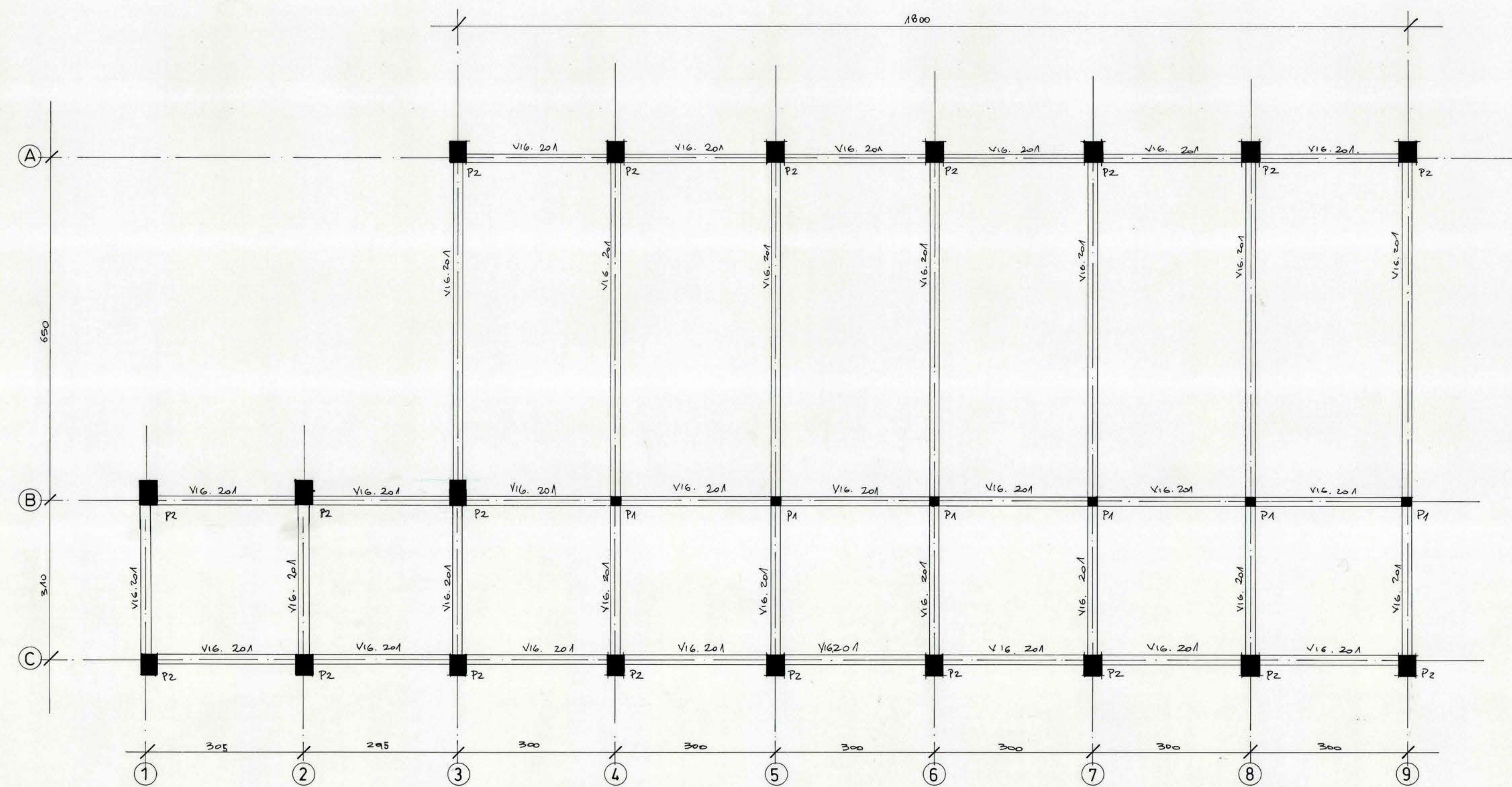
PLANTA DE ESTRUCTURAS 2º PISO.
