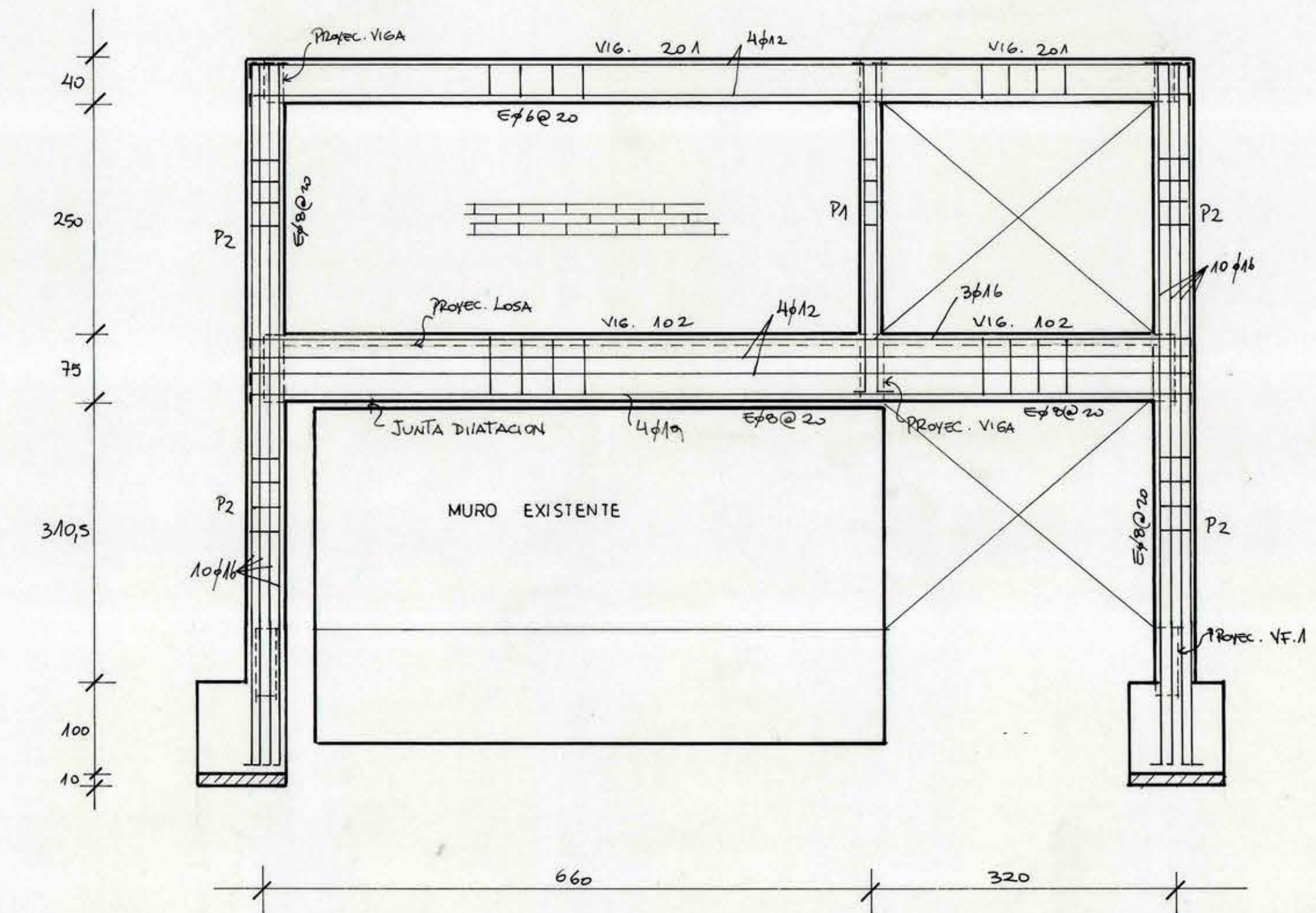
ELEVACION EJE 7.
