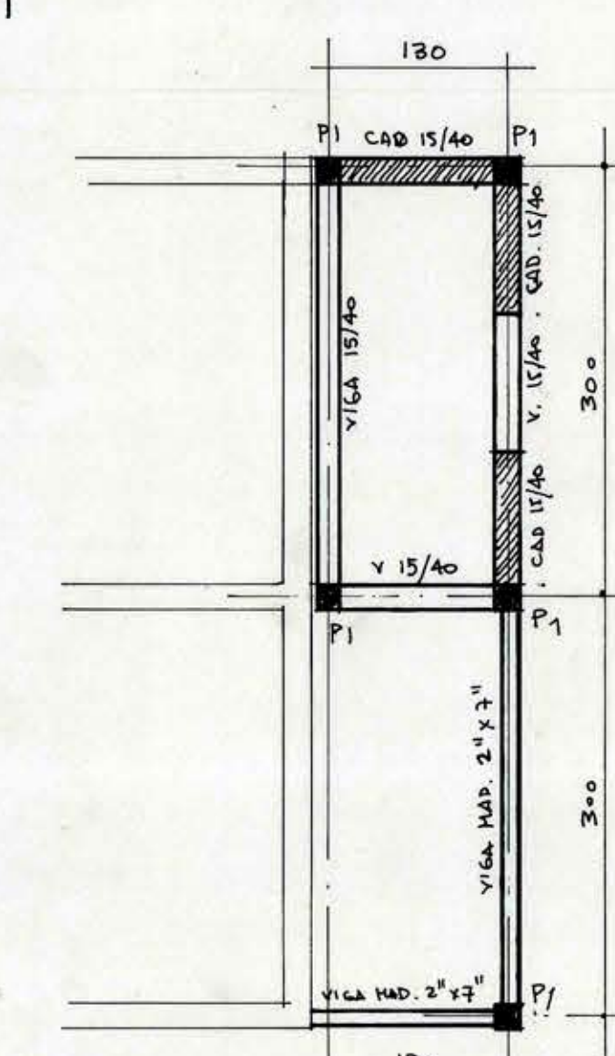
PLANTA ESTR.
