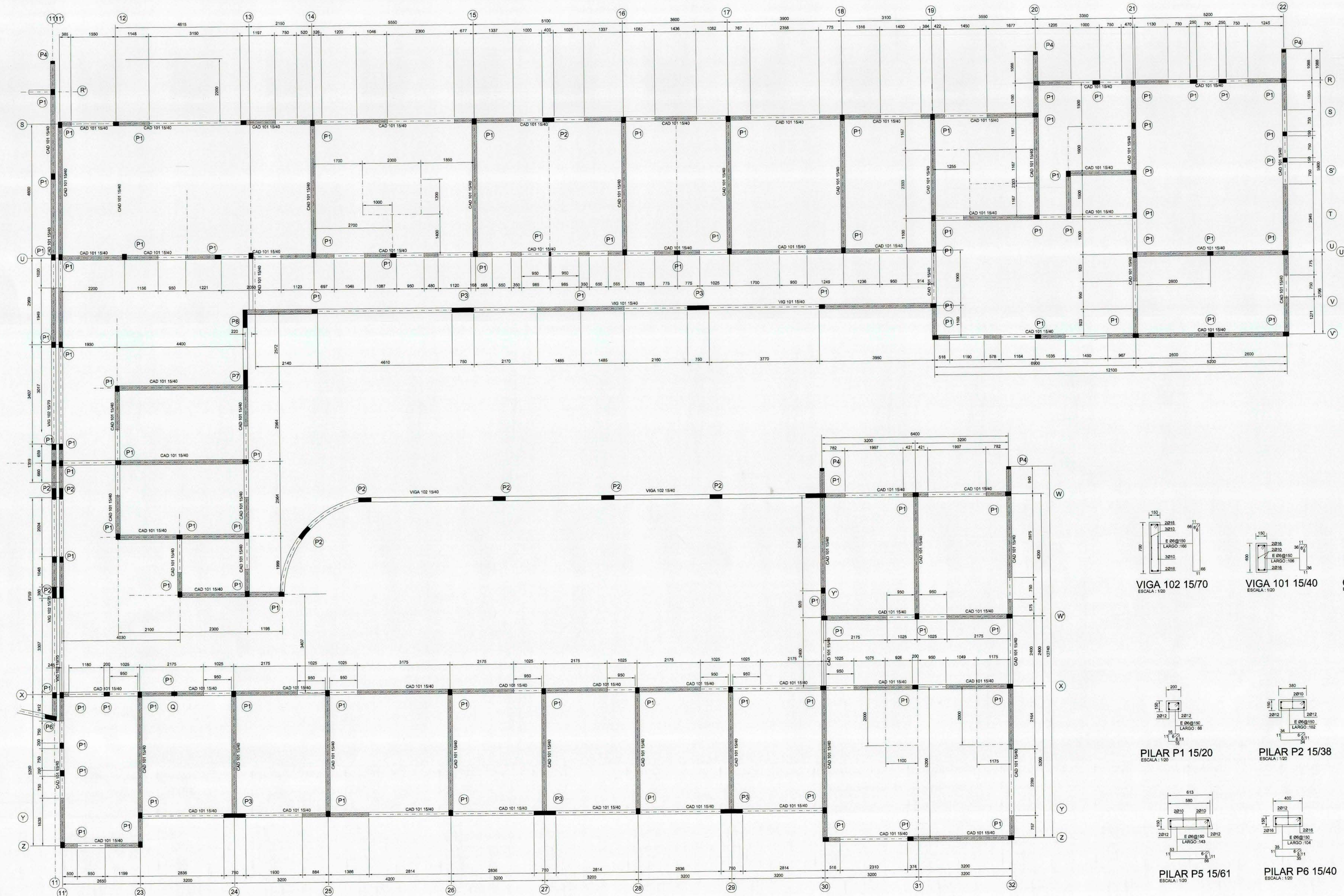
PLANTA DE ESTRUCTURAS (MODULO C) ESCALA: 1/50
