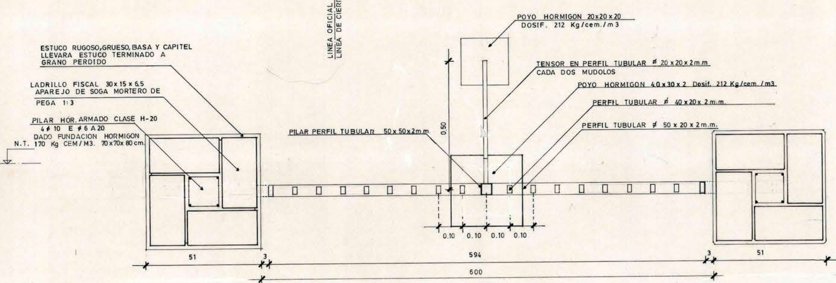
PLANTA MODULO REJA ESC. 1:10
