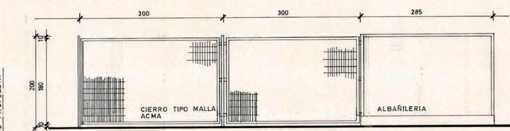
DETALLE TIPO CIERRO MALLA ACMA ESC. 1:50
