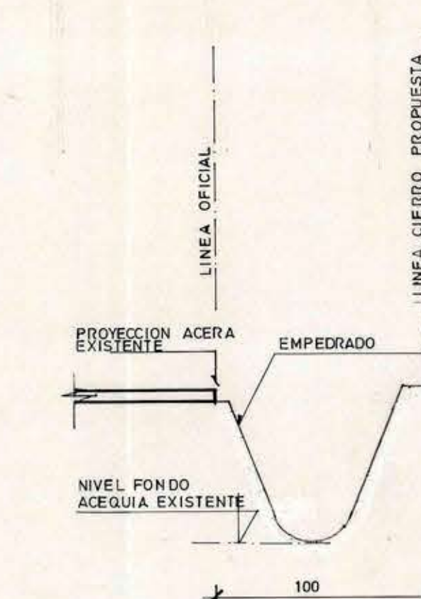
DETALLE TIPO CIERRO MALLA ACMA ESC. 1:50
