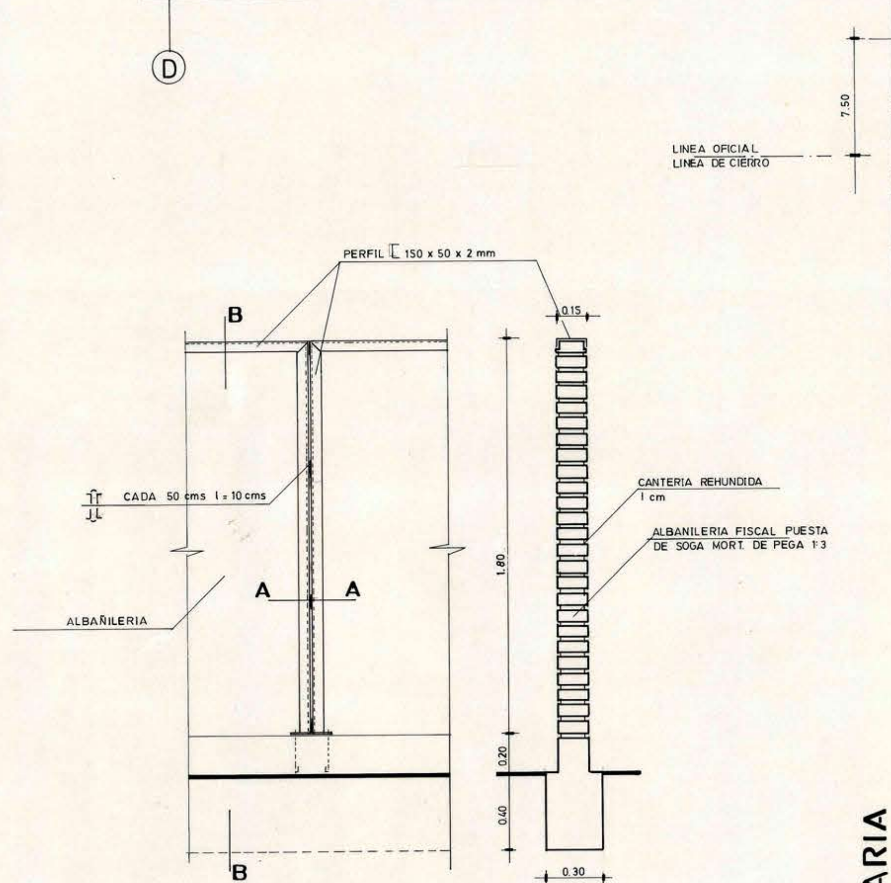
ELEVACION ESC. 1:20
