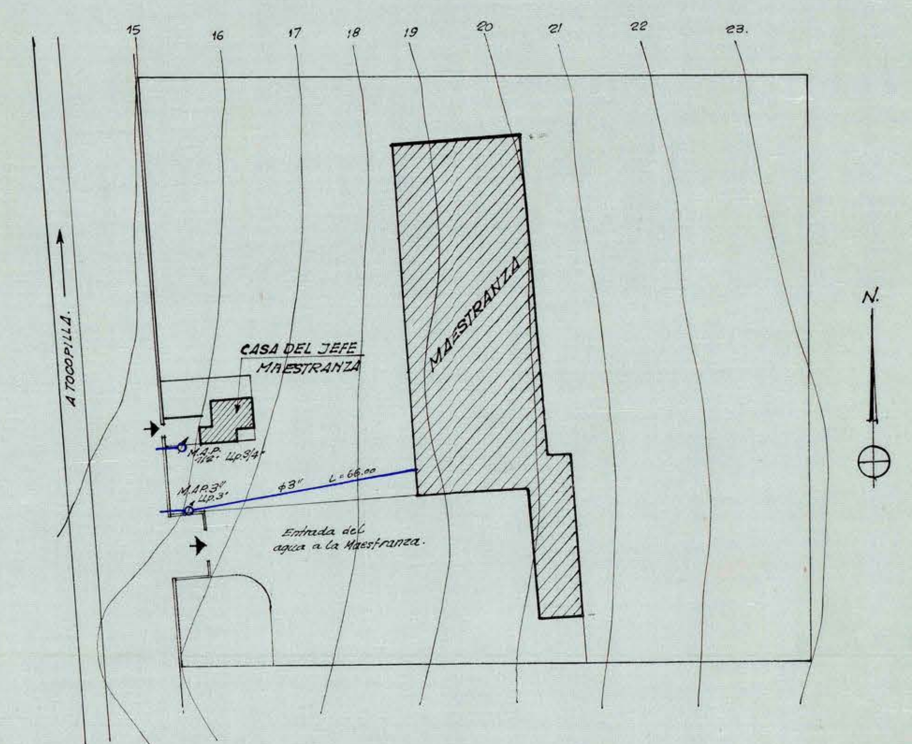
PLANO DE UBICACION ESCALA 1:1000.
