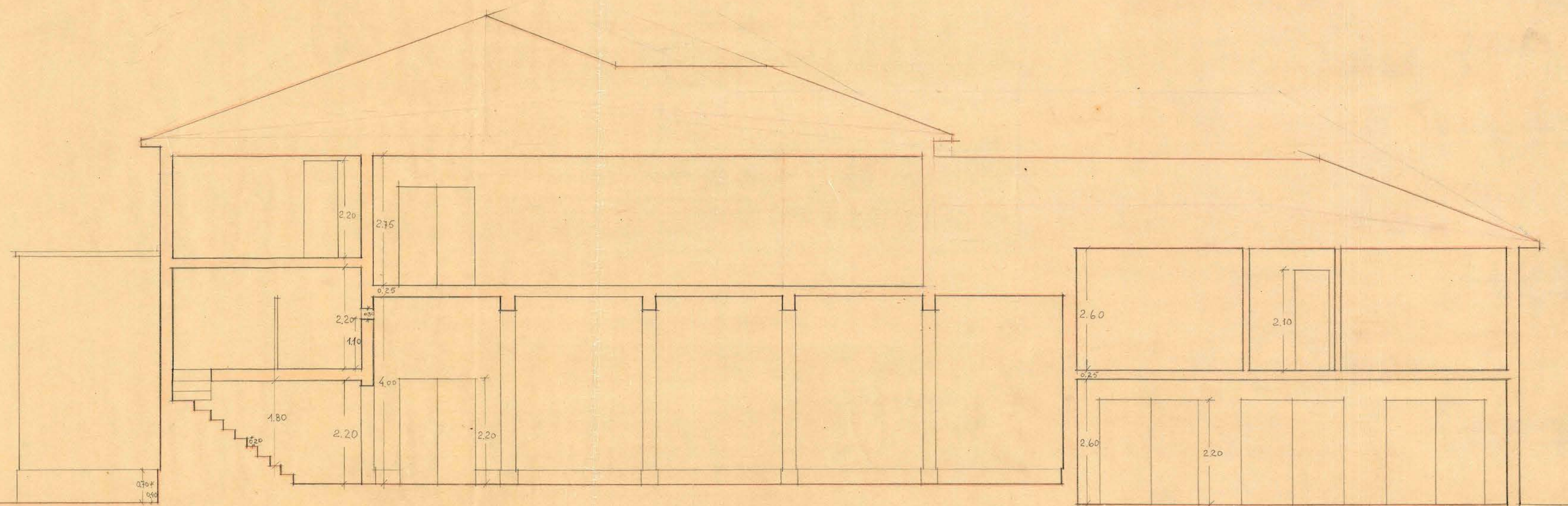
SECCION A-A
