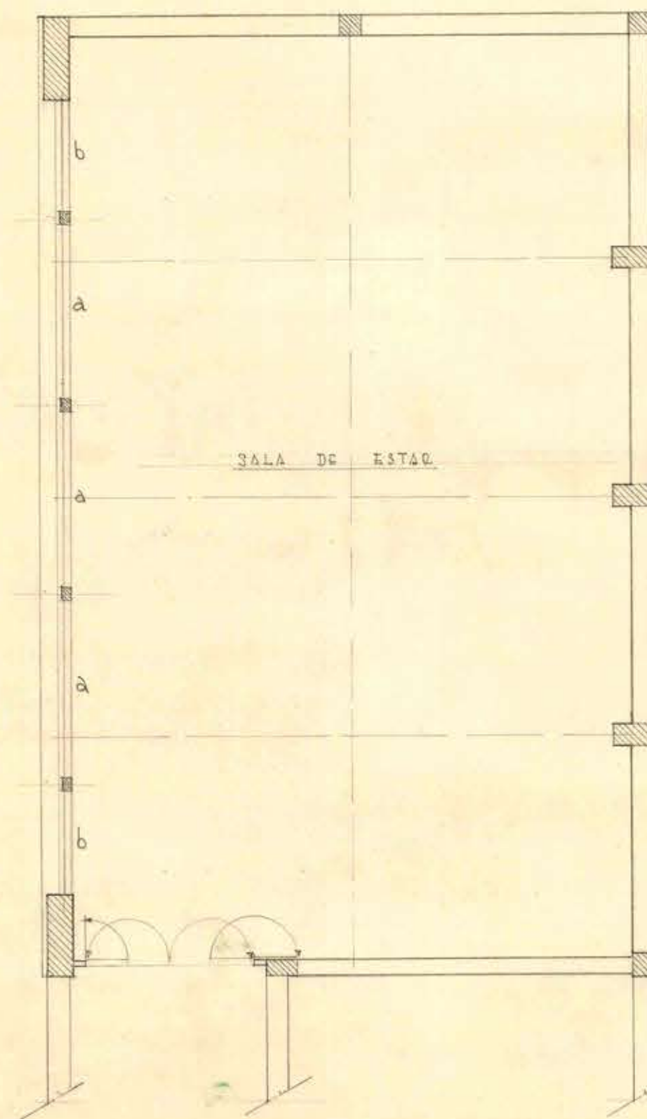
PLANTA 1 er PISO
