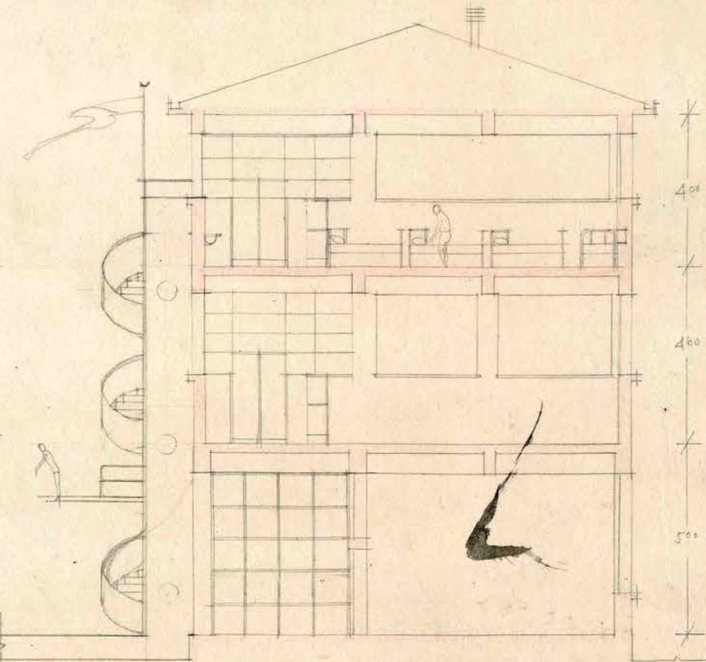
SECCION A-A
