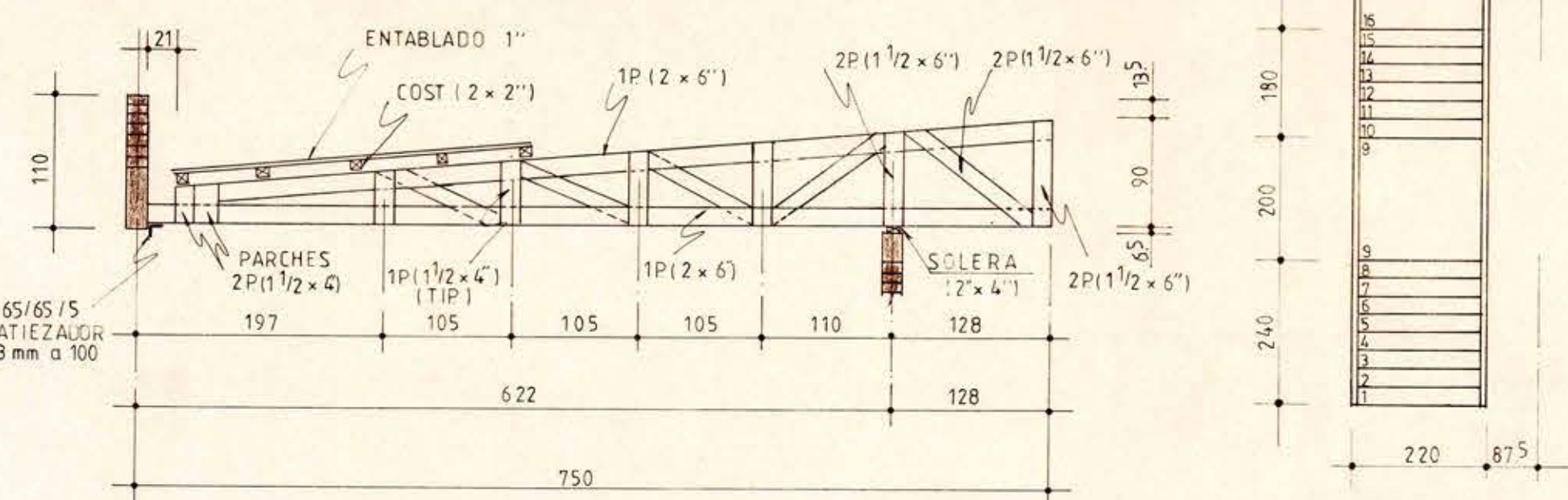
CERCHA C2
