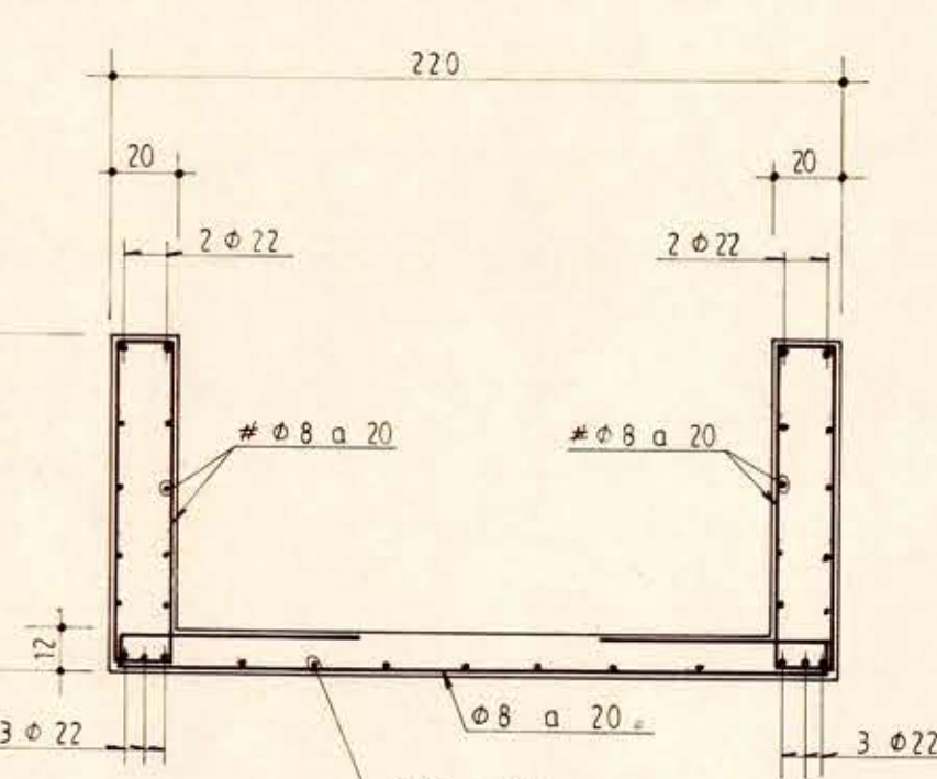
SECCION TRANSVERSAL ESCALERA
