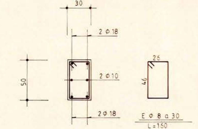
PILAR P3 30/50
