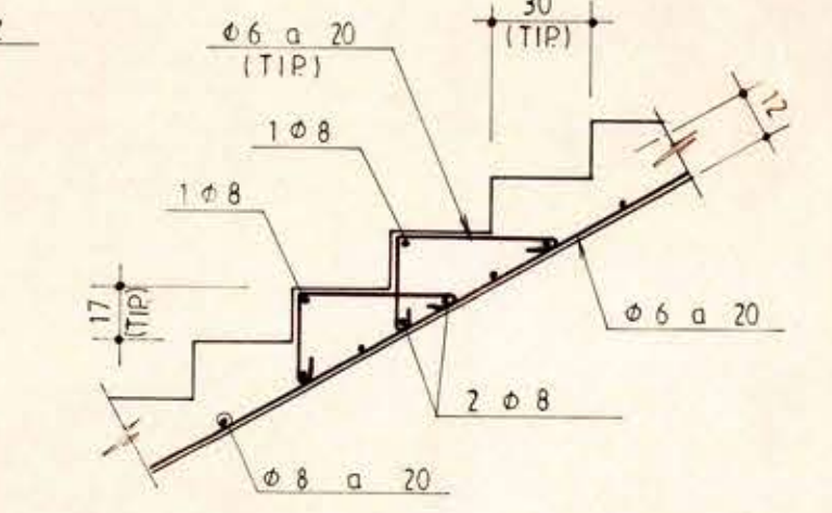
SECCION LONGITUDINAL ESCALERA
