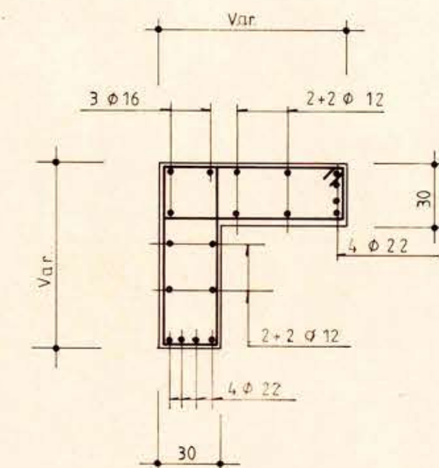
PILAR P2 30/Var.
