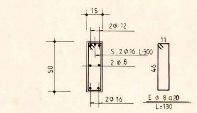
VIGA V 15/50
