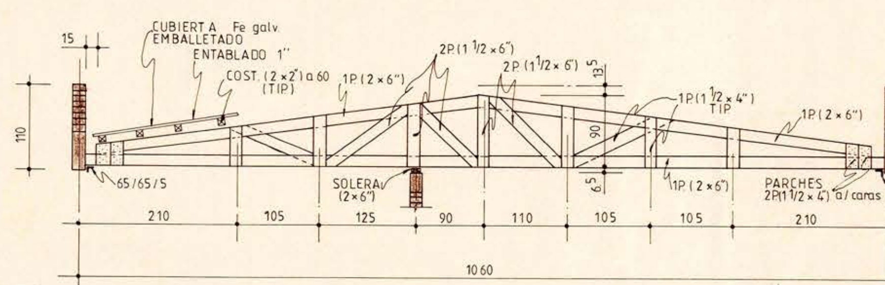
CERCHA C1
