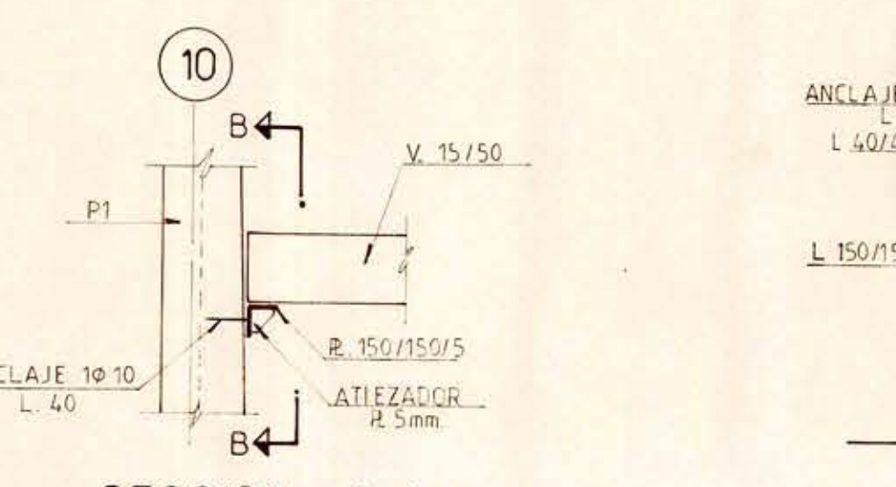
SECCION A-A
