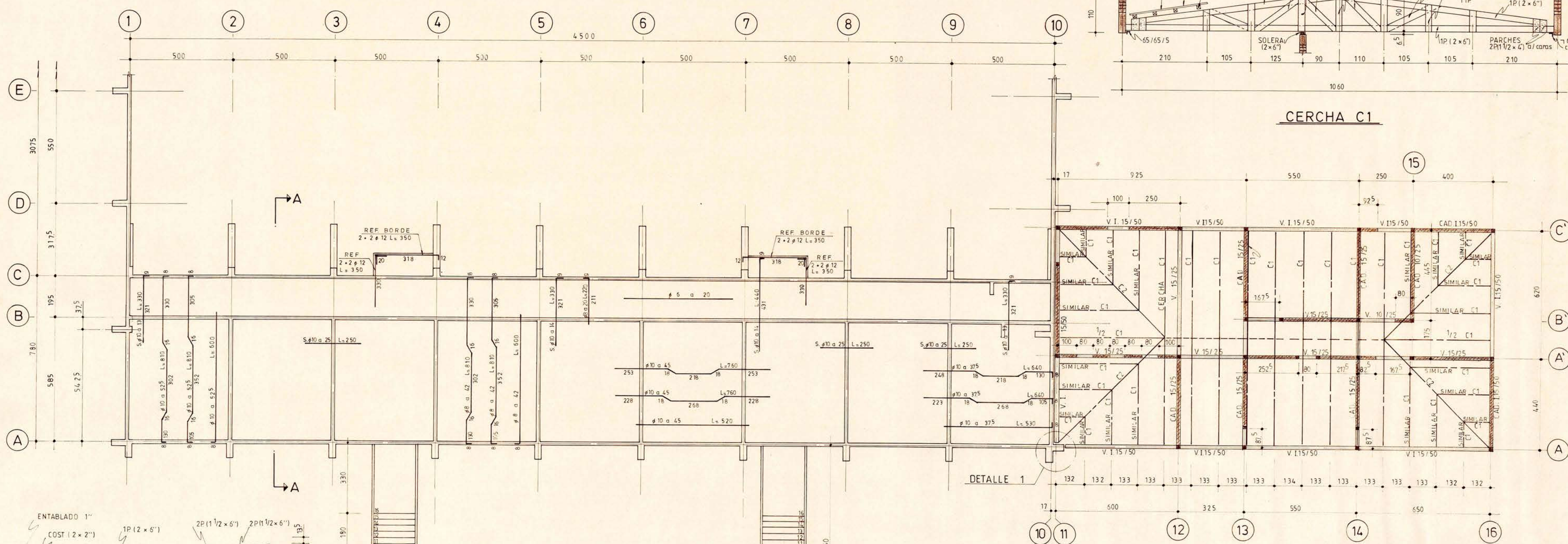
PLANTA ESTRUCTURA 2º PISO PLANTA DE TECHUMBRE
