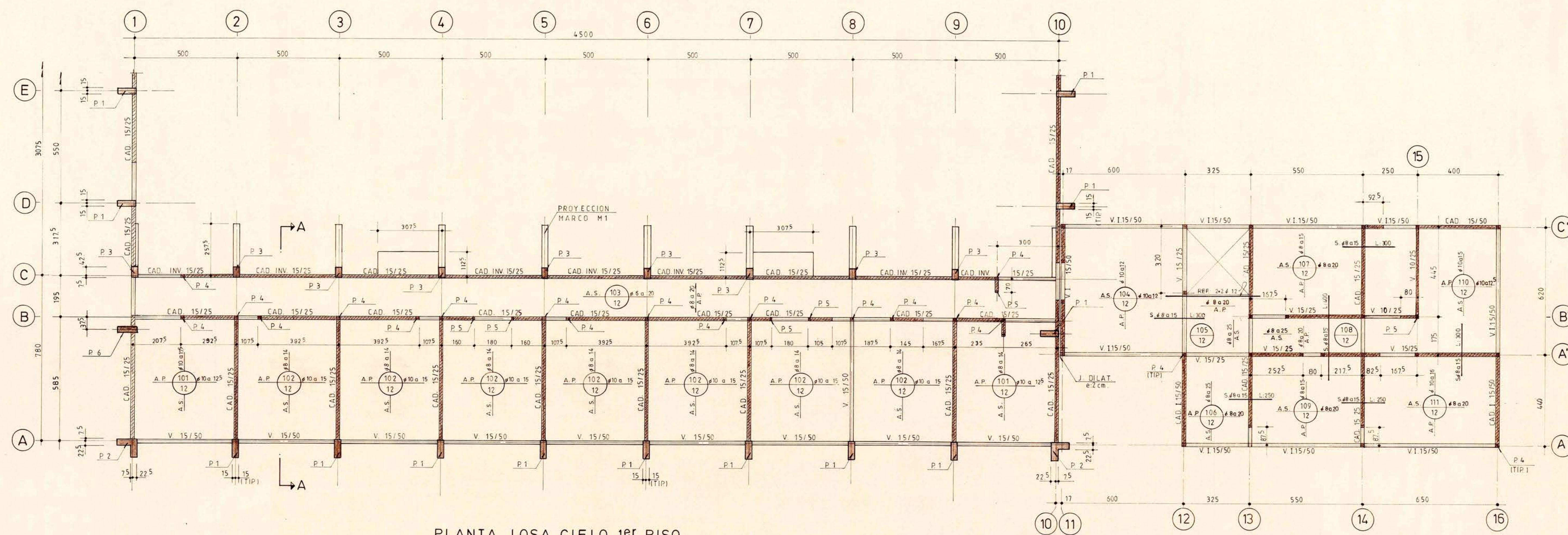
PLANTA LOSA CIELO 1er PISO DIMENSIONES (NIVEL + 275)
