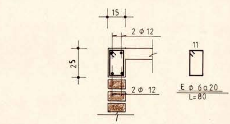
CADENA CAD 15/25 SIMILAR CADENA INV. 15/25
