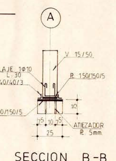
SECCION B-B
