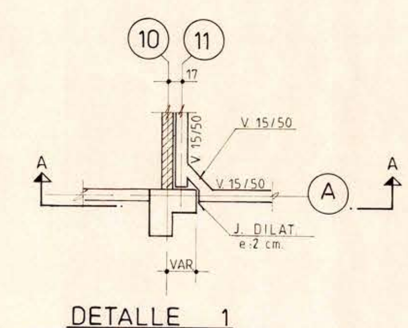
DETALLE 1
