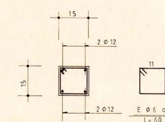
PILAR P4 15/15
