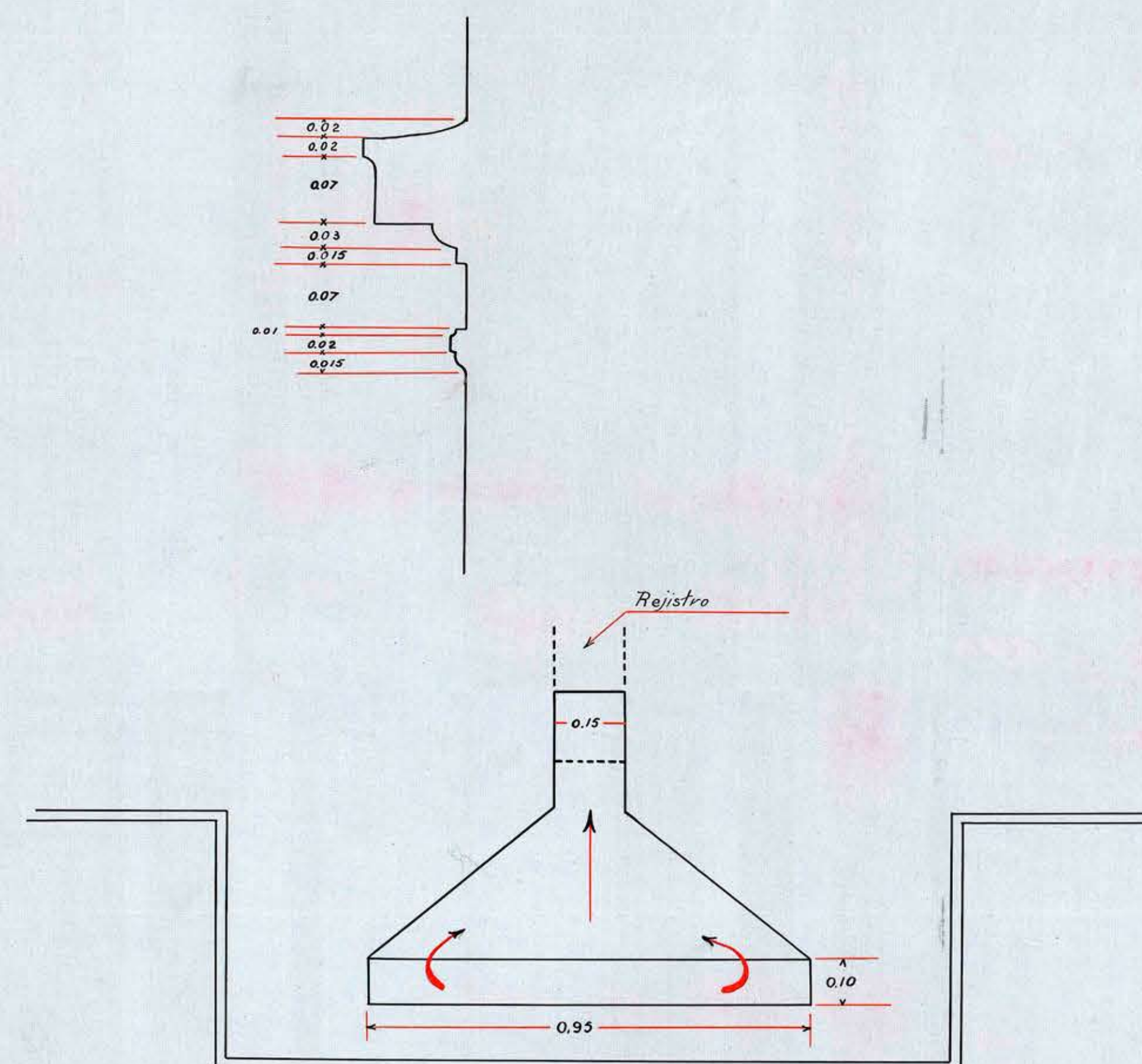
CORTE CD
