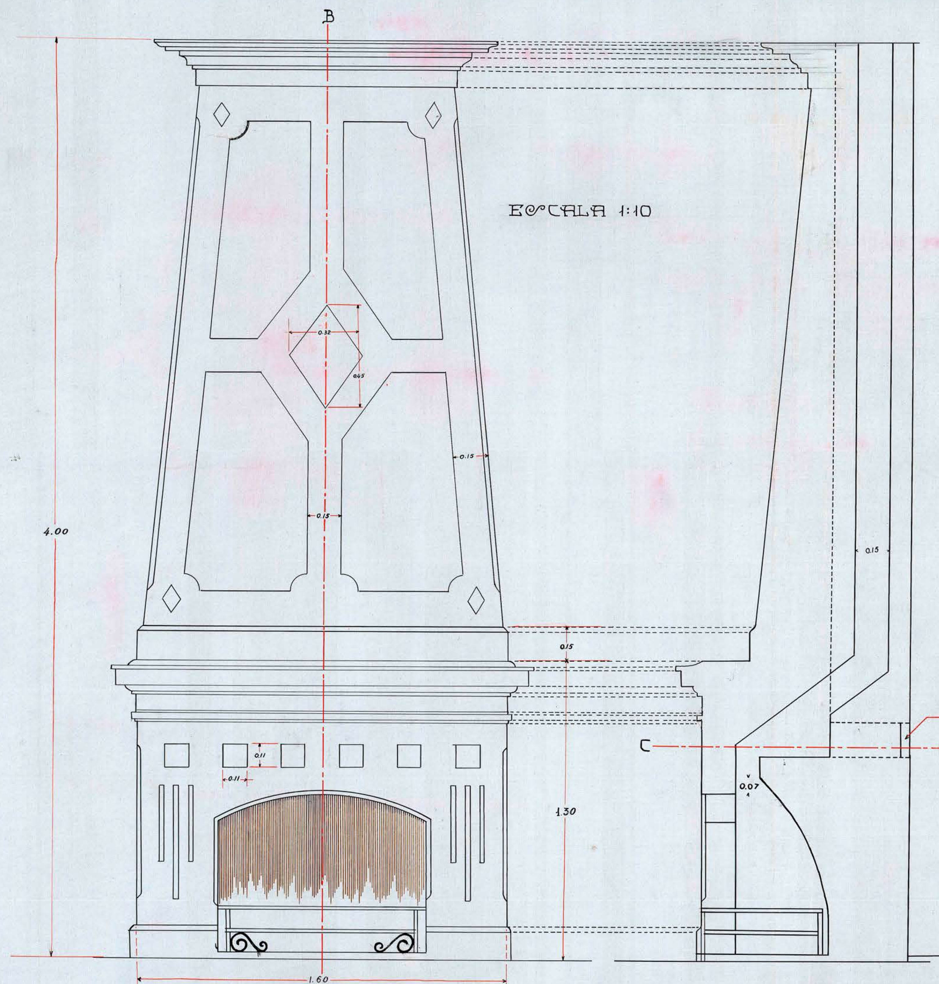
FACHADA
