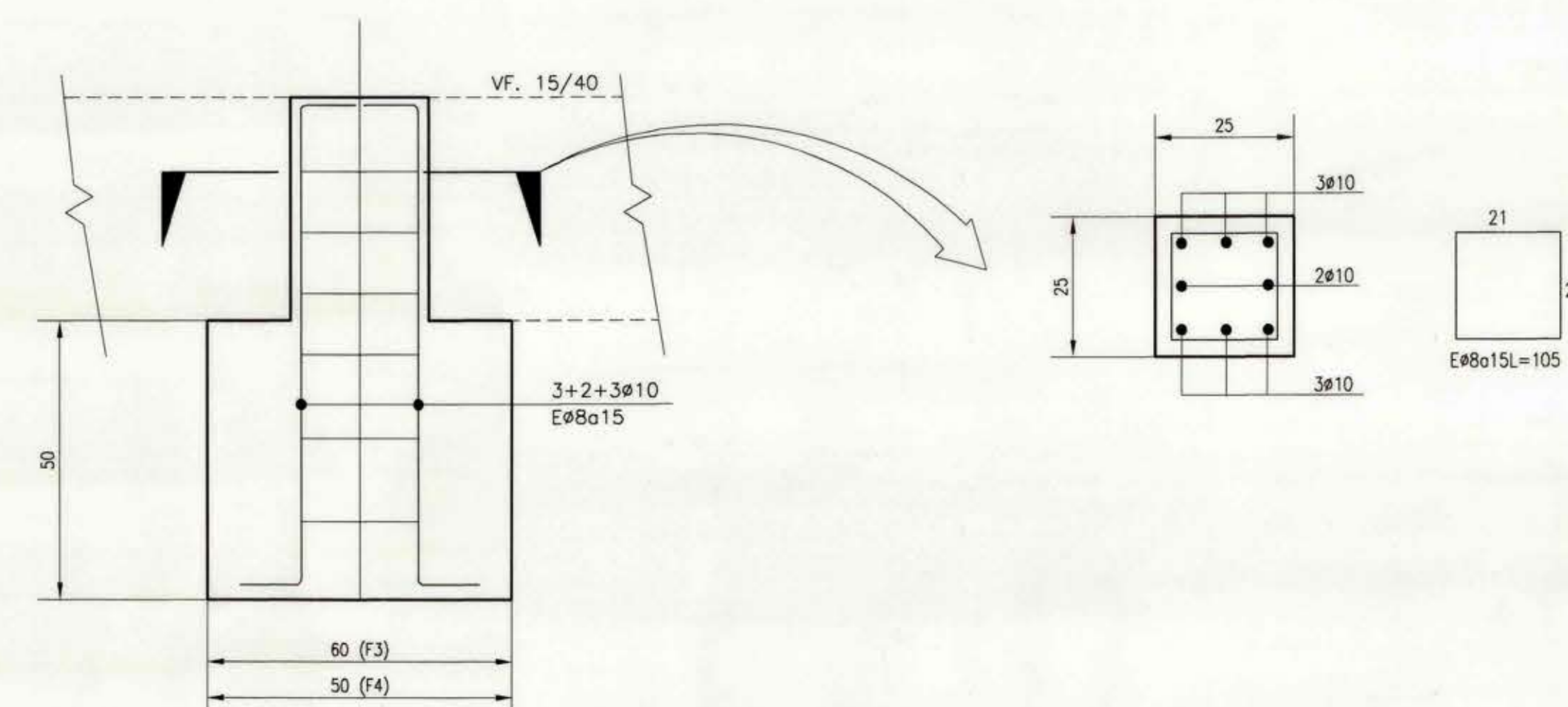
ZAPATA F3-F4 ESC. 1:10
