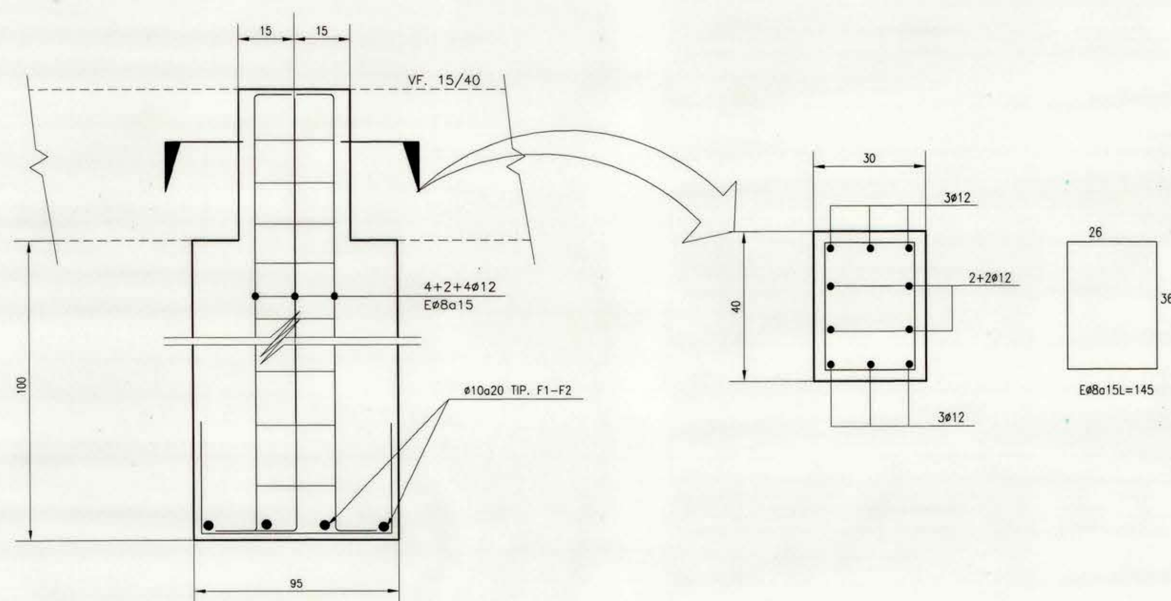
ZAPATA F2 ESC. 1:10
