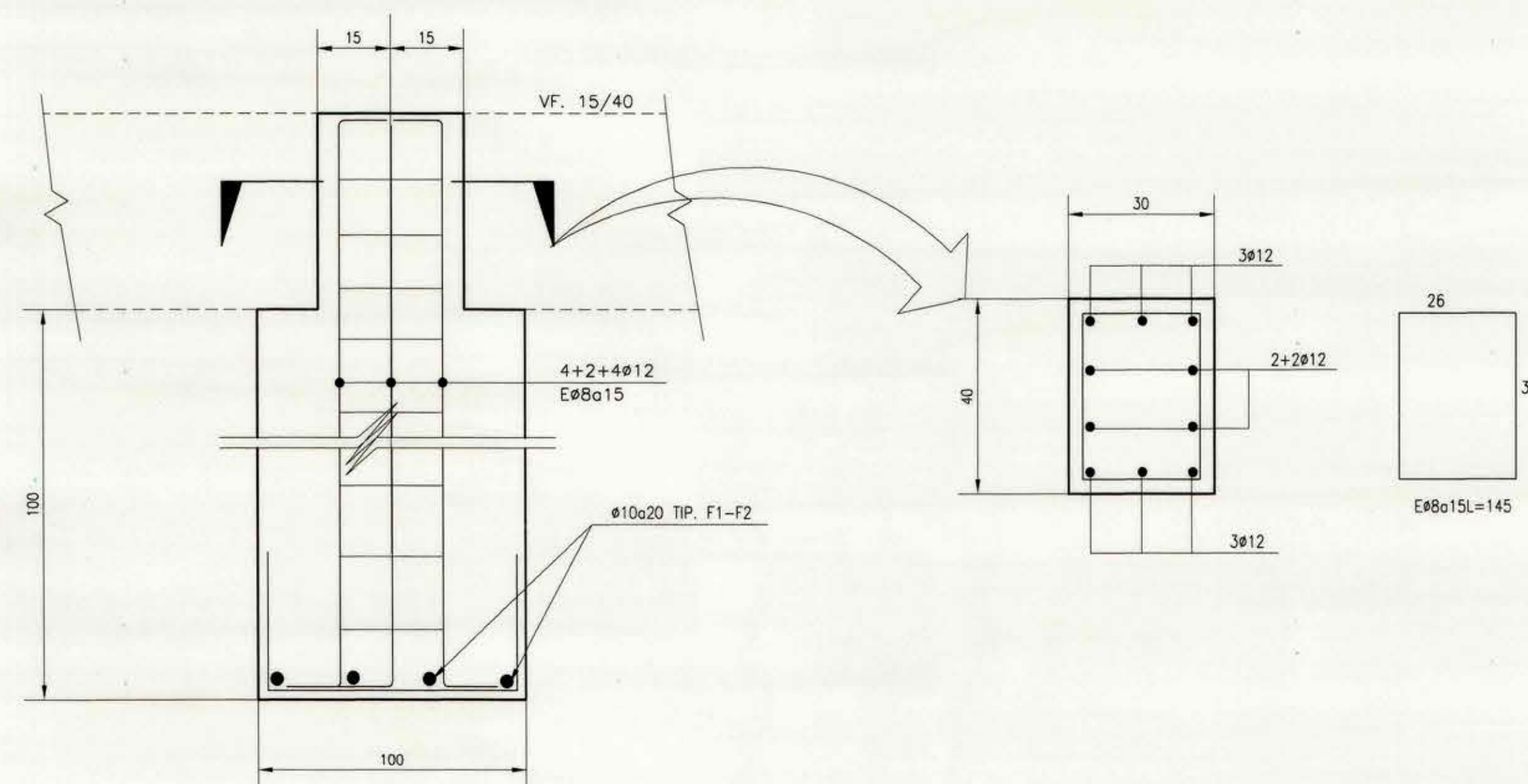
ZAPATA F1 ESC. 1:10
