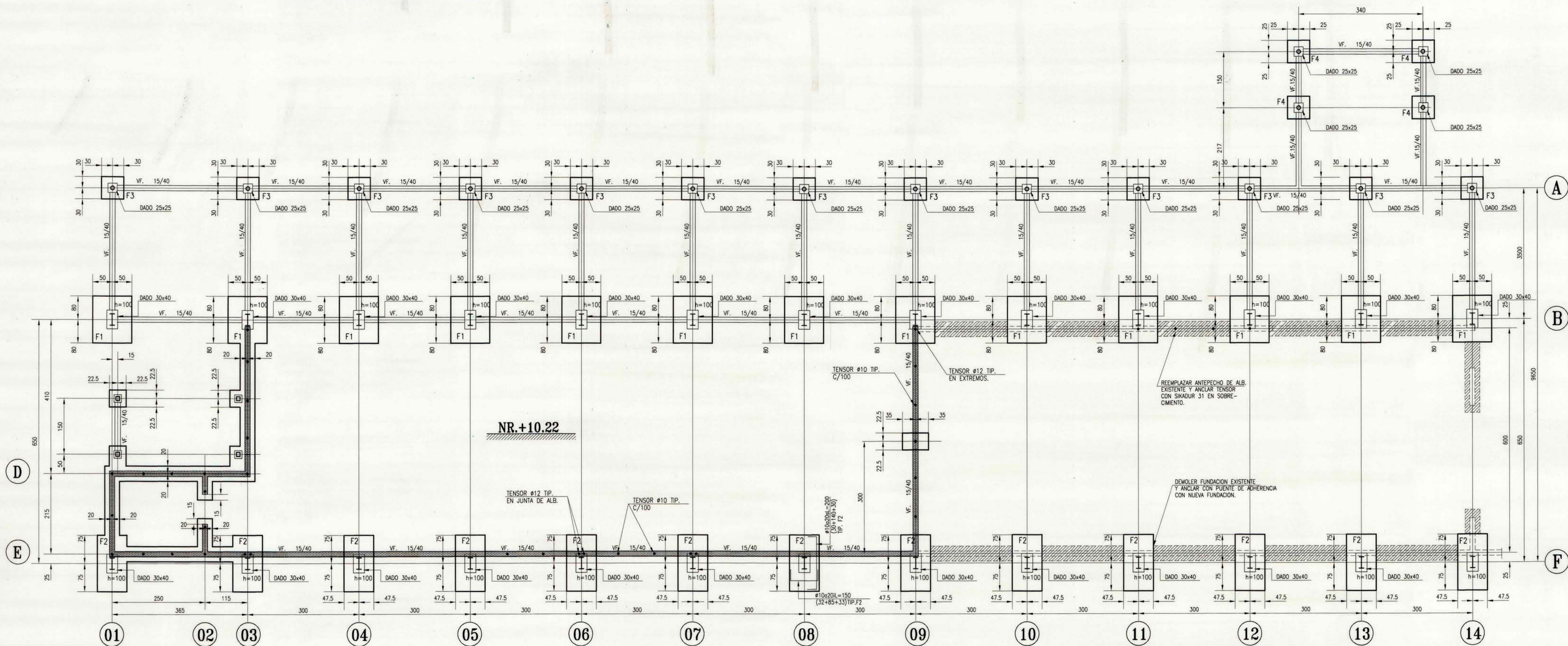
PLANTA DE FUNDACIONES ESC. 1:50
